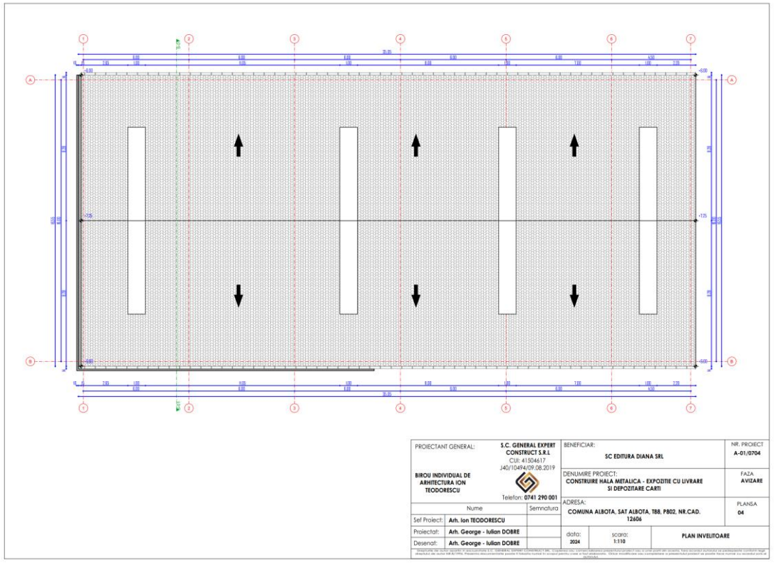
-plan invelitoare:
