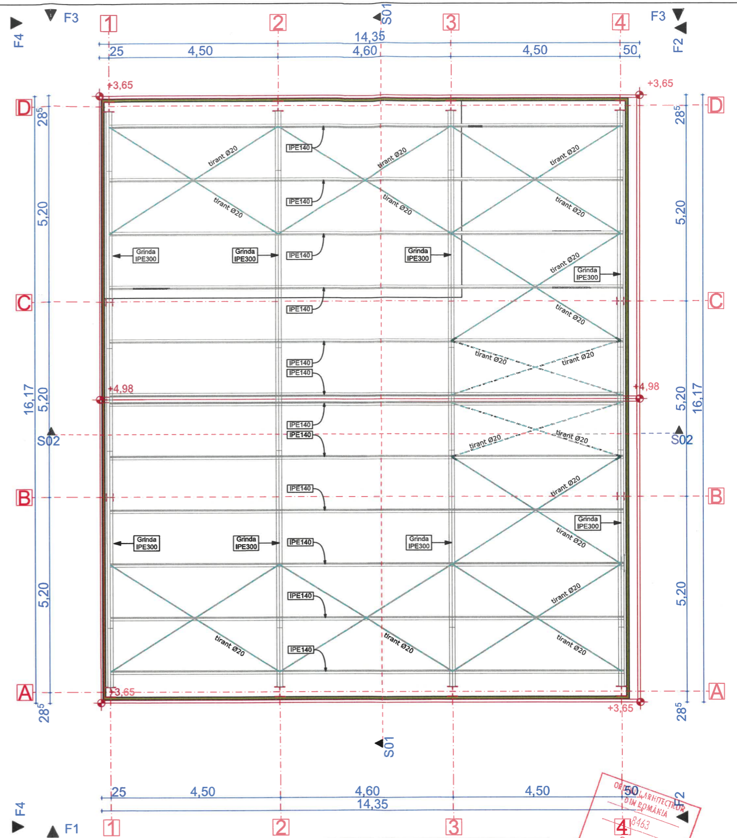
Plan Invelitoare
