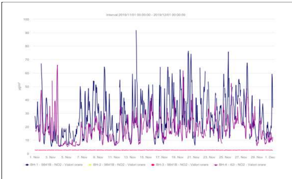
Fig.2.2.7. Concentrații NO 2
