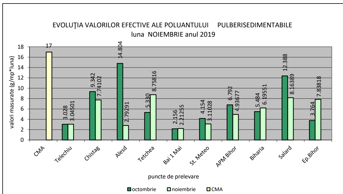
Fig.2.1.1.1. Pulberi sedimentabile
