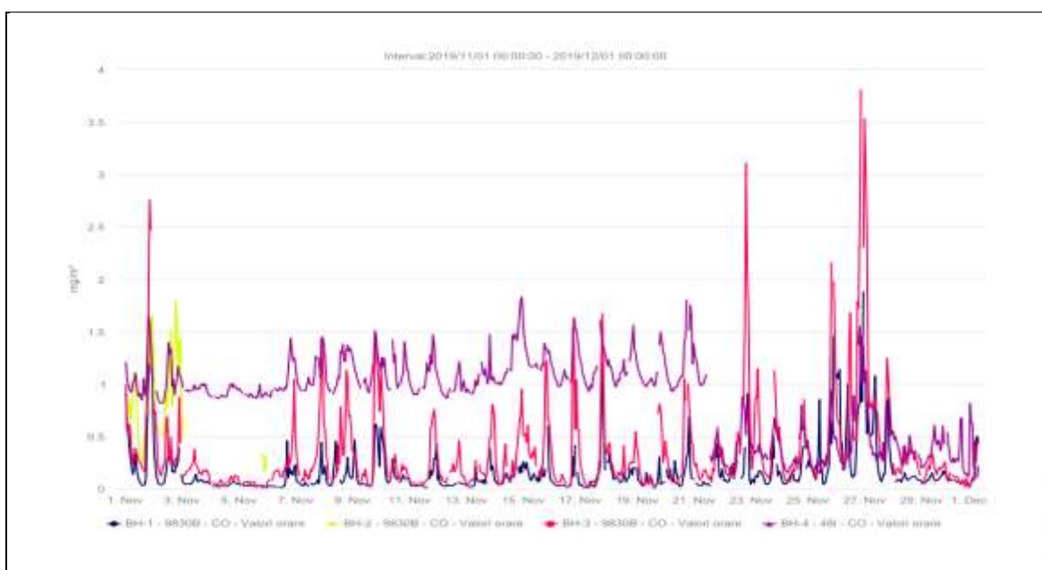
Fig.2.2.8. Concentrații CO
