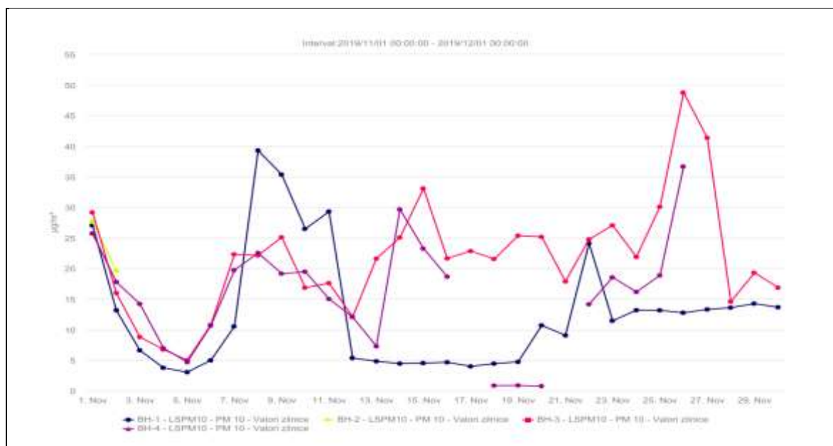
Fig.2.2.9. Concentrații PM_{10}
