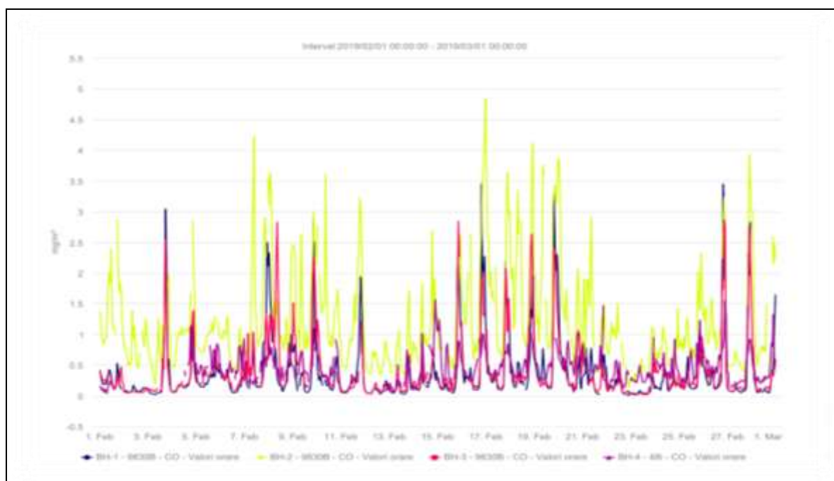
Fig.2.2.5. Concentrații CO
