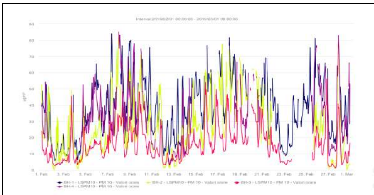
Fig.2.2.6. Concentrații PM_{10}
