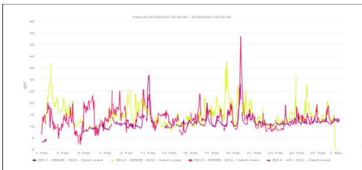
Fig.2.2.3. Concentrații \text{SO}_2
