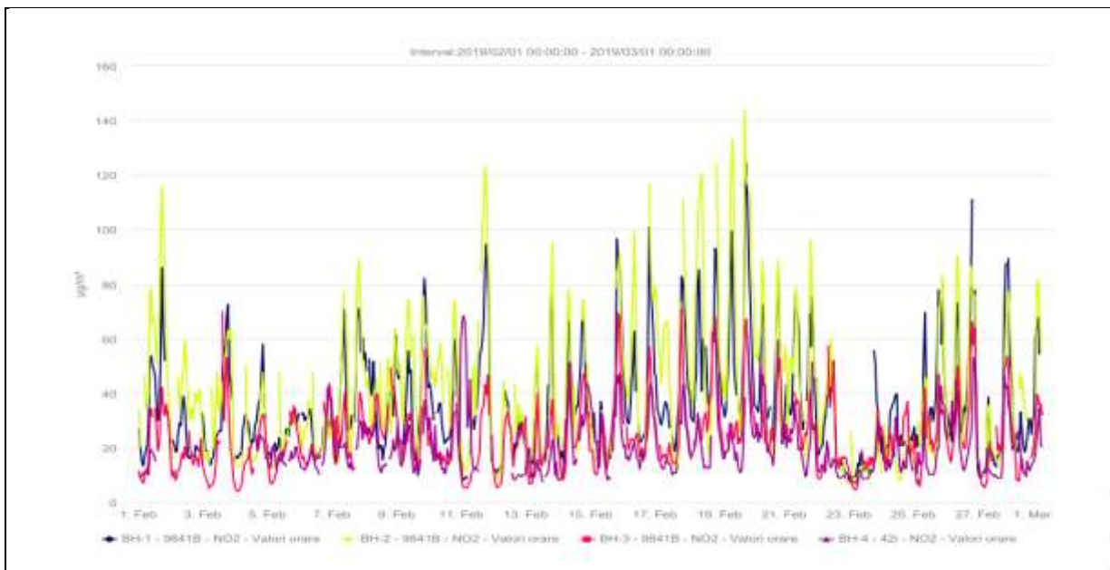
Fig.2.2.4. Concentrații NO 2
