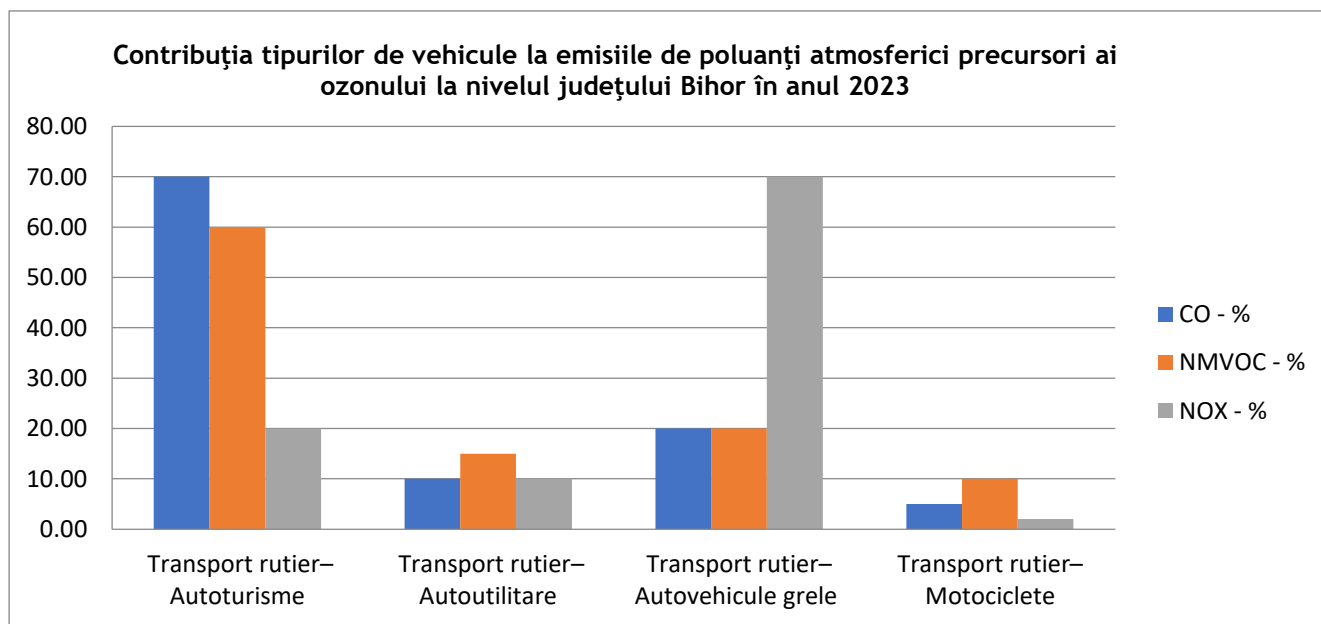
Fig. I.2.1.3.2 Contribuția transportului la emisiile de poluanți precursori ai ozonului
