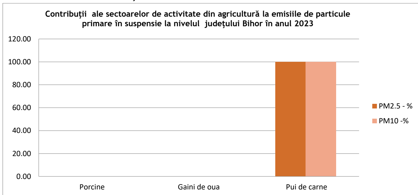
Fig. I.2.1.4.3 Contribuția sectoarelor de activitate din agricultură la emisiile de particule primare
