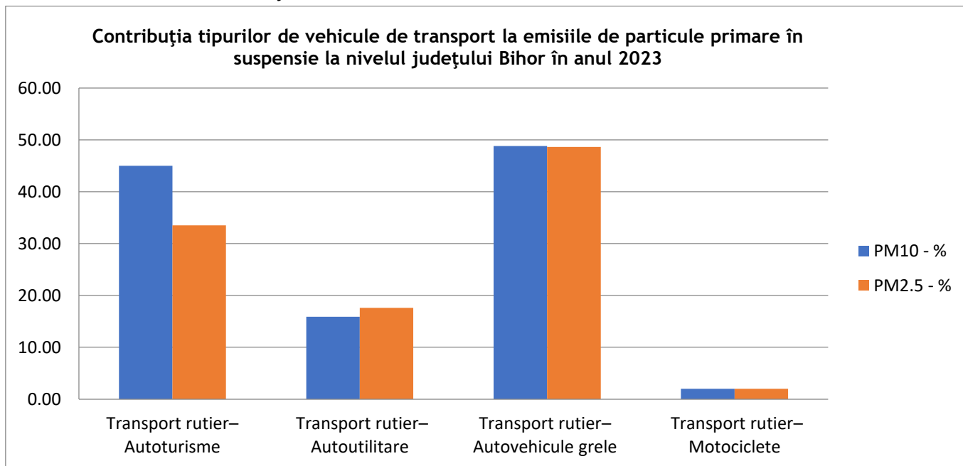
Fig. I.2.1.3.3 Contribuția transportului la emisiile de particule în suspensie
