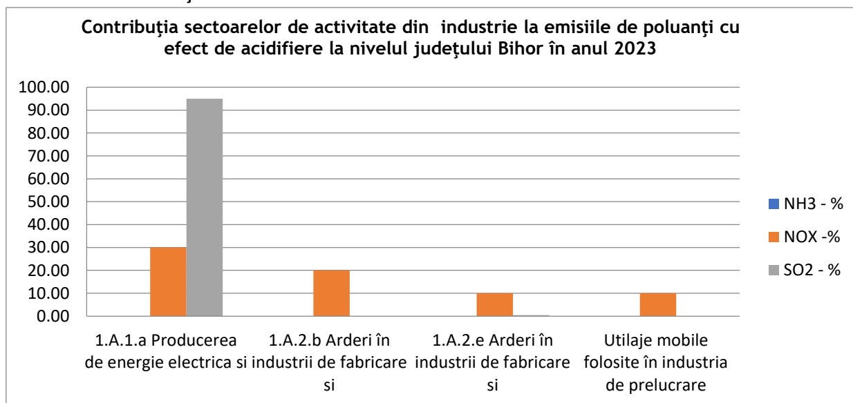
Fig. I.2.1.2.1 Contribuția sectoarelor de activitate din industrie la emisiile de poluanți cu efect de acidifiere
