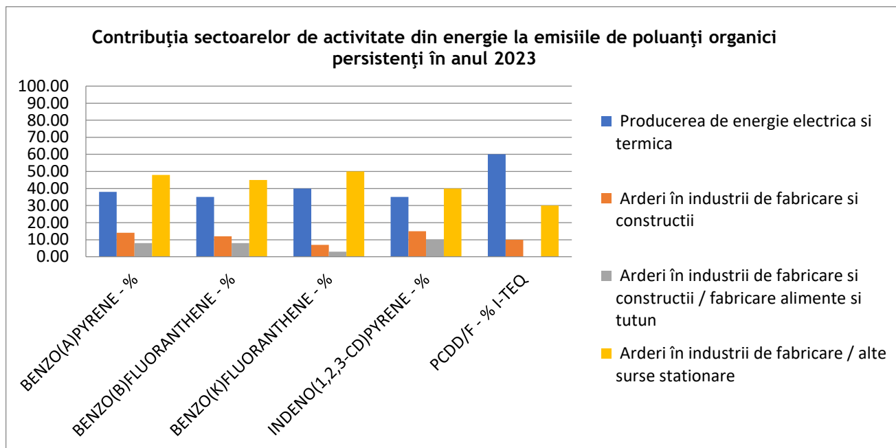
Fig. I.2.1.5 Contribuția sectoarelor din energie la emisiile de poluanți organici persistenți
