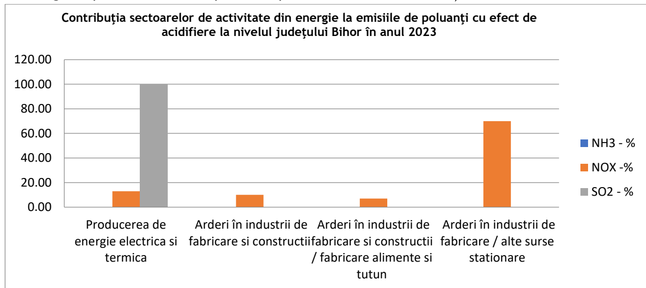
Fig. I.2.1.1 Contribuția emisiilor de substanțe acidifiante din energie
