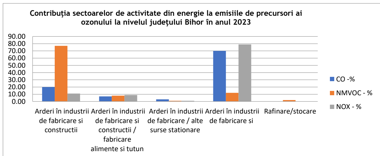
Fig. I.2.1.2 Contribuția energiei la emisiile de poluanți precursori ai ozonului
