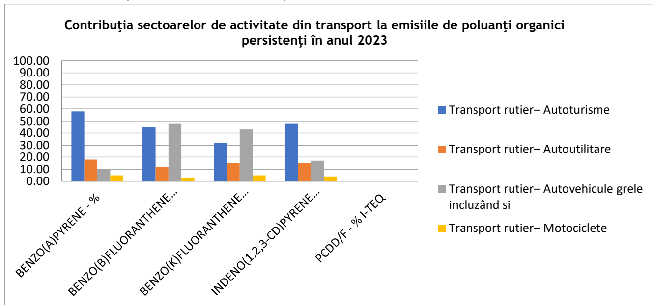
Fig. I.2.1.3.5 Contribuția transportului la emisiile de poluanți organici persistenți
