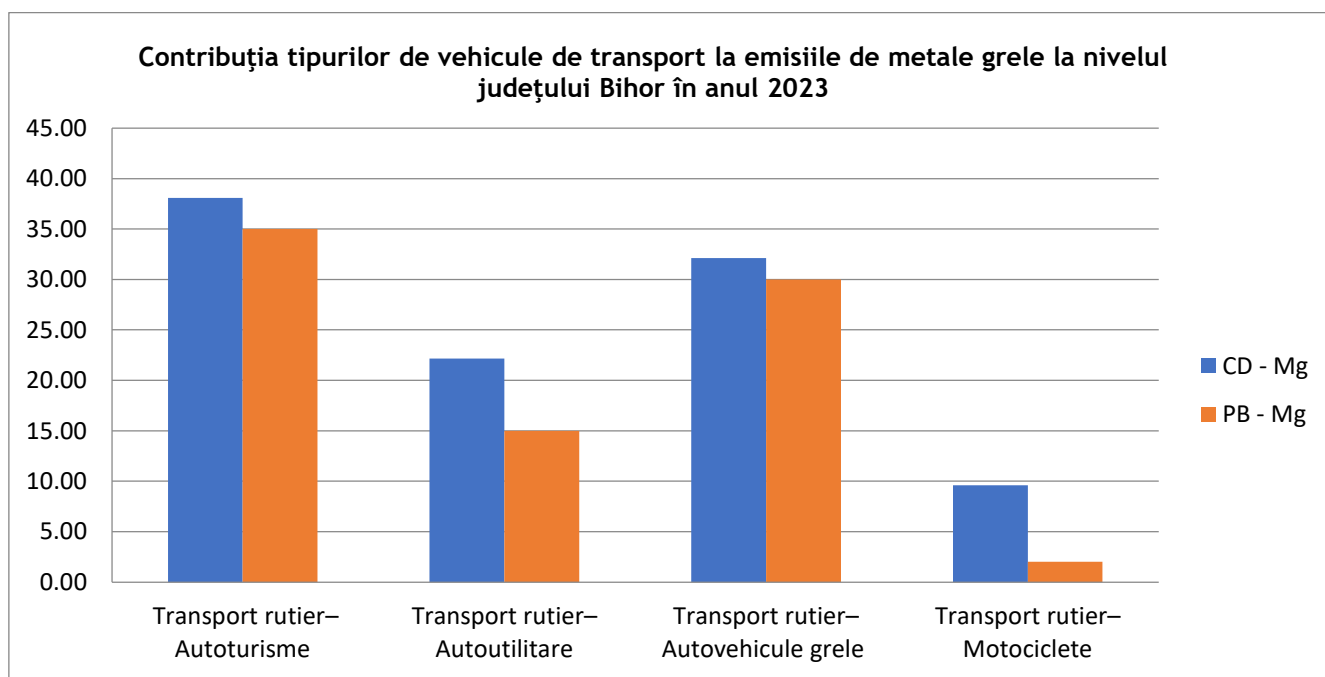
Fig. I.2.1.3.4 Contribuția transportului la emisiile de metale grele
