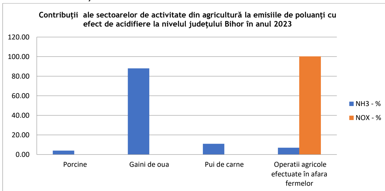
Fig. I.2.1.4.1 Contribuția sectoarelor de activitate din agricultură la emisiile de poluanți cu efect de acidifiere
