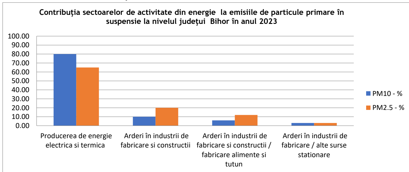
Fig. I.2.1.3 Contribuția sectoarelor din energie la emisiile de particule primare în suspensie
