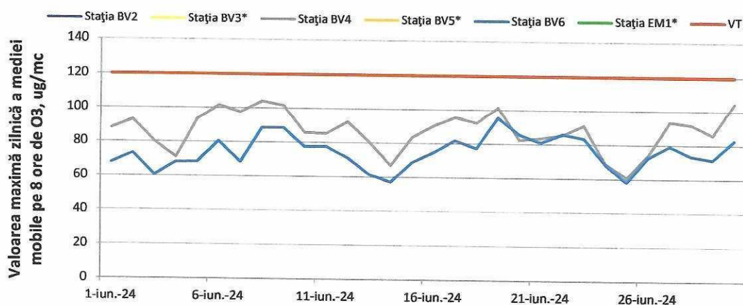
Figura 3. Evoluția concentrațiilor maximelor zilnice ale mediilor mobile pe 8 ore de O 3 în luna iunie 2024
