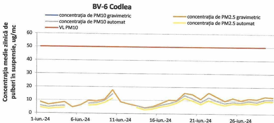
Figura 9. Evoluția concentrațiilor medii zilnice de PM10 gravimetric și automat și PM2,5 gravimetric și automat în stația de fond urban BV-6 în luna iunie 2024
