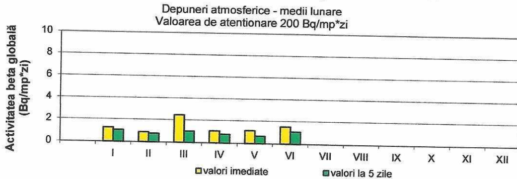
Figura 18. Activitatea beta globală pentru depuneri atmosferice
