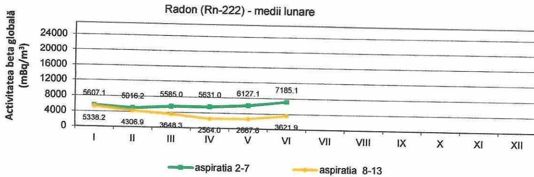
Figura 16. Activitatea calculată a Radonului
