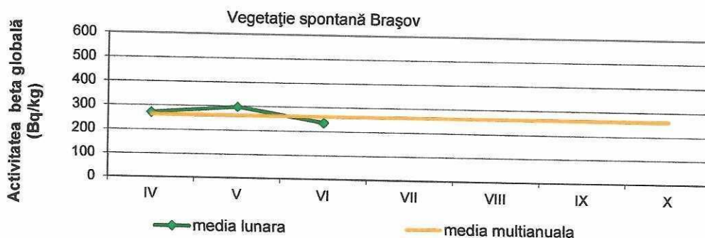
Fig. 23. Activitatea beta globală la 5 zile pentru vegetație spontană
