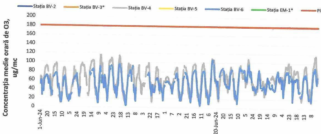
Figura 4. Evoluția concentrațiilor medii orare de O 3 în luna iunie 2024
