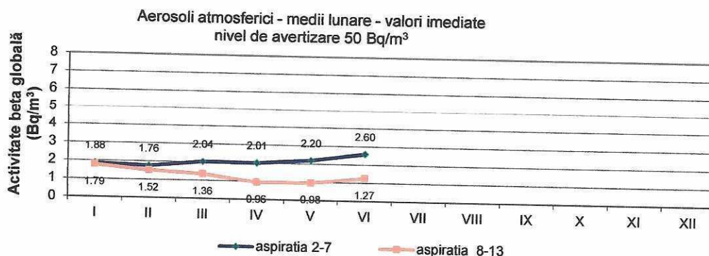
Figura 15. Activitatea beta globală pentru aerosoli atmosferici
