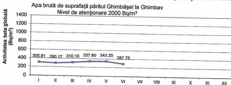
Figura 19. Activitatea beta globală imediată pentru apa de suprafață Pârâul Ghimbășel
