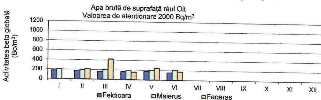
Fig. 21. Activitatea beta globală la 5 zile pentru apa de suprafață Râul Olt
