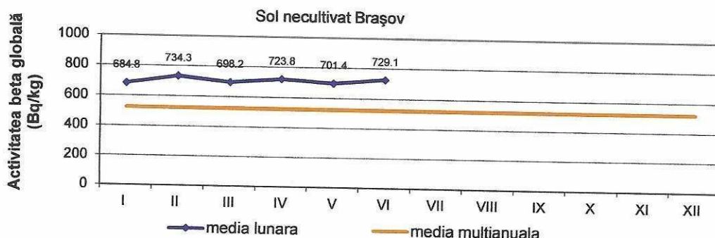
Fig. 22. Activitatea beta globală la 5 zile pentru solul necultivat
