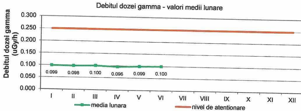
Figura 17. Debitul dozei gamma
