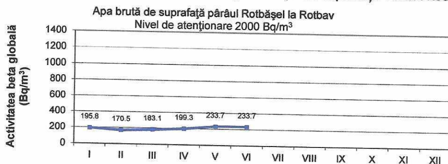
Figura 20. Activitatea beta globală la 5 zile pentru apa de suprafață-Pârâul Rotbășel
