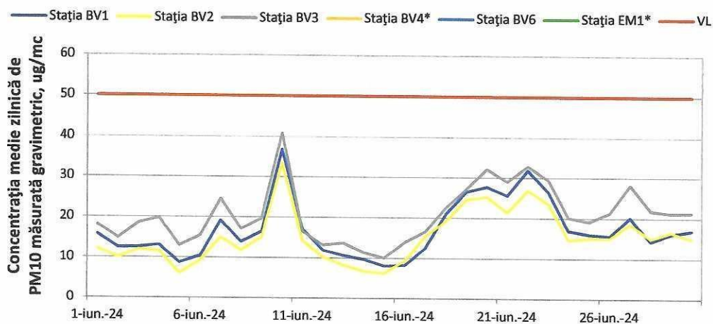
Figura 5. Evoluția concentrațiilor medii zilnice de PM 10 (gravimetric) în luna iunie 2024
