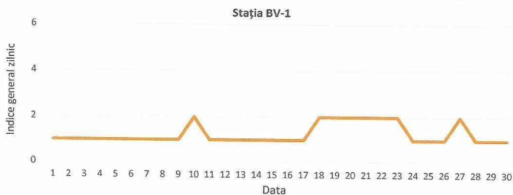
Figura 10. Evoluția indicelui general de calitate a aerului din stația BV-1
