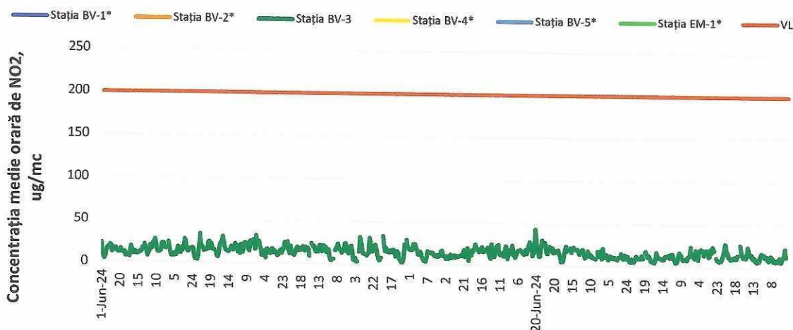
Figura 1. Concentrații medii orare de NO 2 în luna iunie 2024
