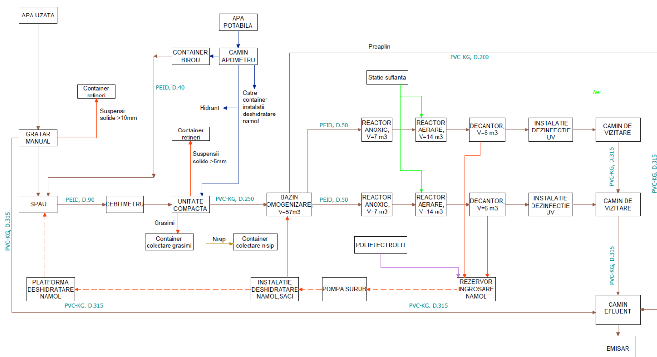
Fig. 1 – Flux tehnologic stație de epurare
