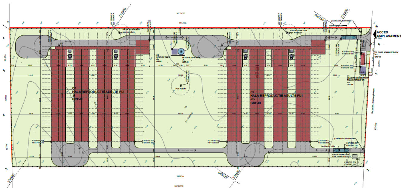
Fig. 4. Plan de situatie
