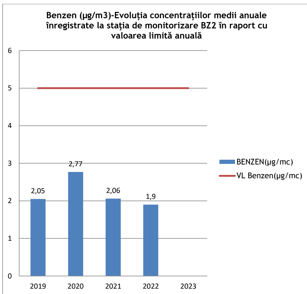
Fig. I.1.1.2.5.2. Evoluția concentrațiilor medii anuale BENZEN la stația BZ-2
