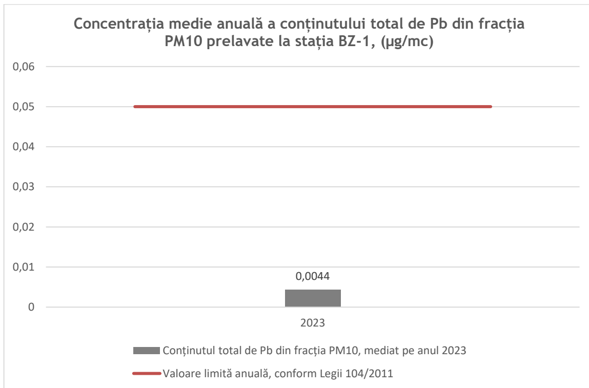
Fig. I.1.1.1.7.1. Concentrația medie anuală a conținutului total de Pb din fracția PM10 prelevate la stația BZ-1, pentru anul 2023 ( \mu\text{g}/\text{mc} )
