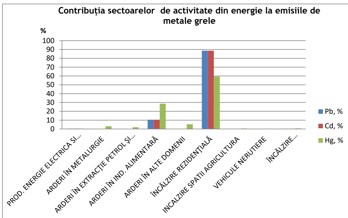
Figura 1.2.1.1.4. Contribuția sectoarelor de activitate din energie la emisiile de metale grele
