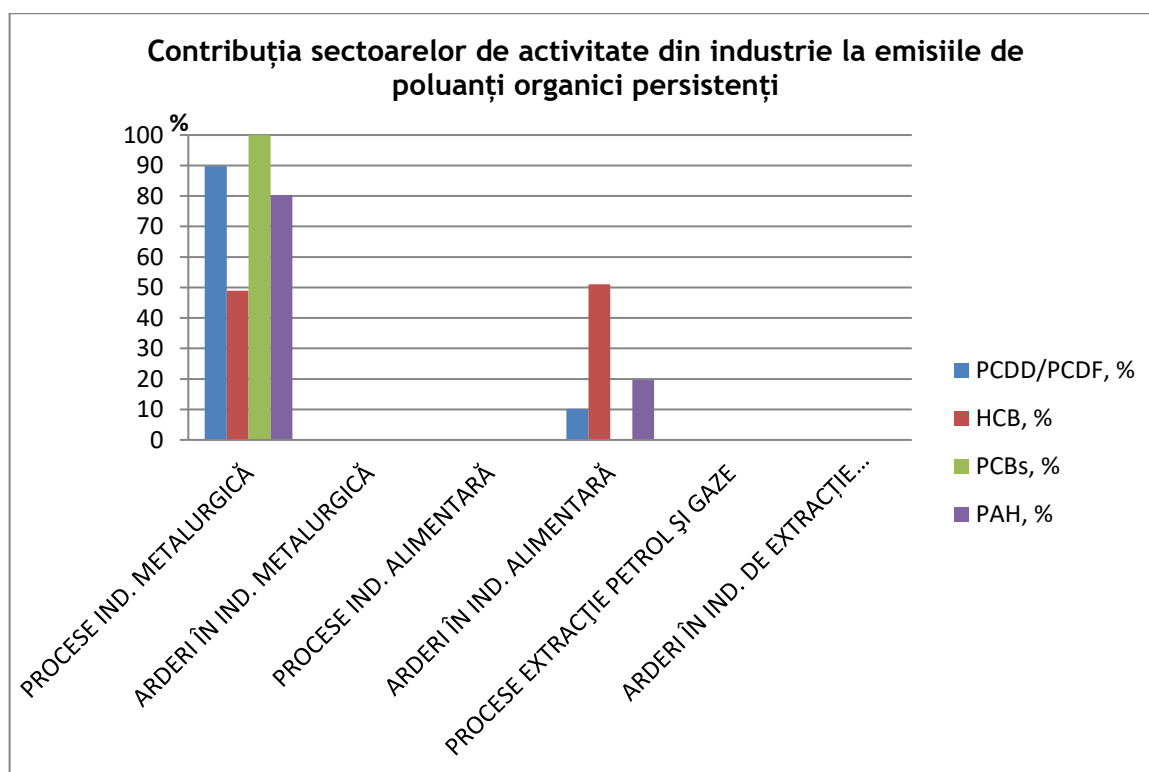
Figura I.2.1.2.11. Contribuția sectoarelor de activitate din industrie la emisiile de poluanți organici persistenți
