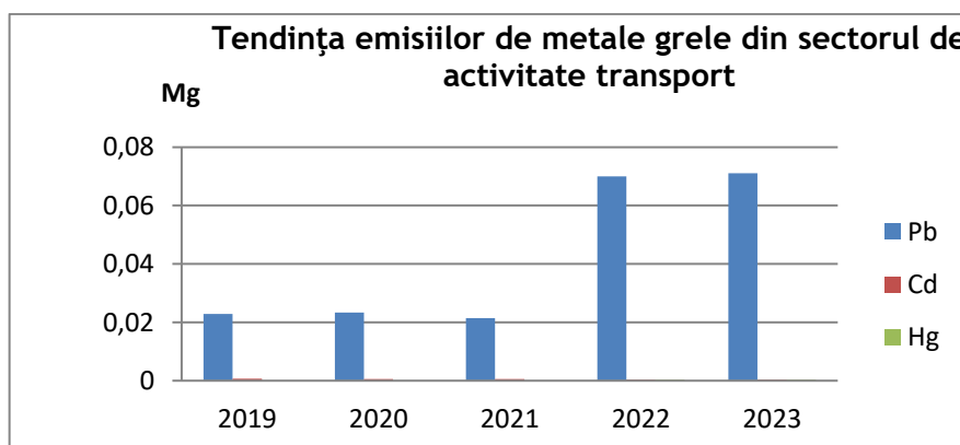
Figura I.3.1.19. Tendința emisiilor de metale grele din transport
