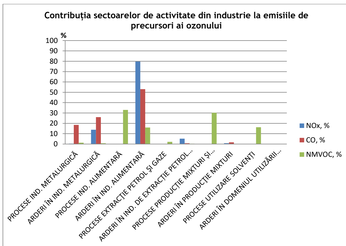
Figura 1.2.1.2.5. Contribuția sectoarelor de activitate din industrie la emisiile de precursori ai ozonului
