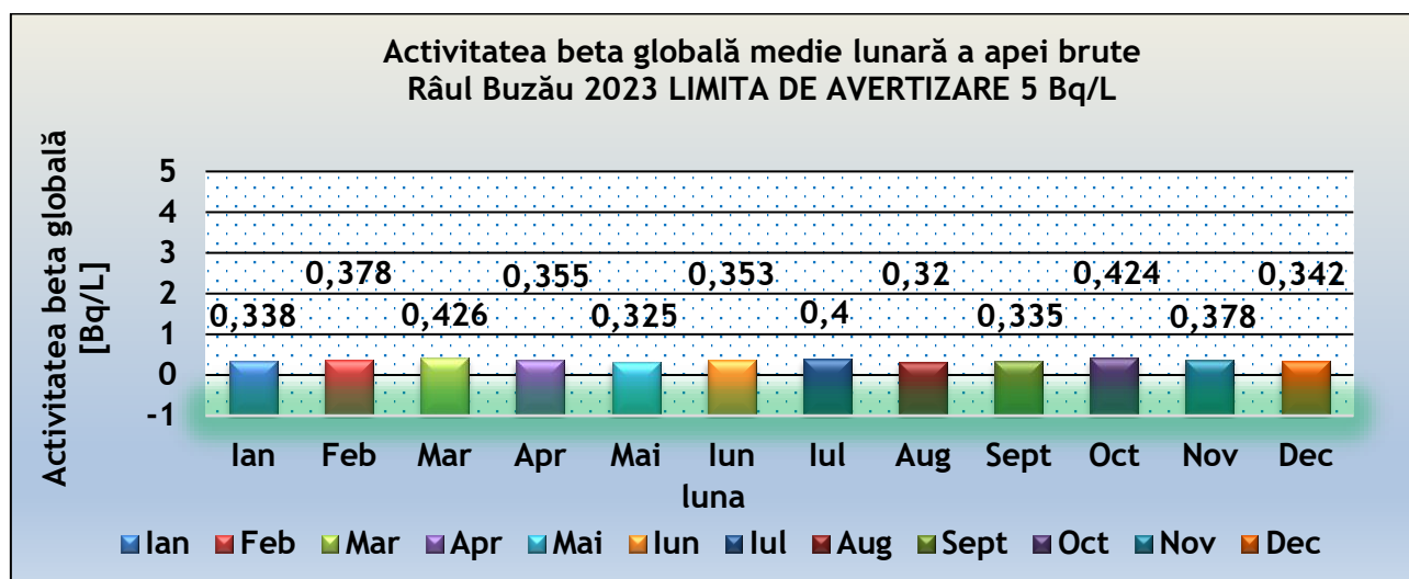
Figura IX.1.2.1.1. Activitatea specifică beta globală medie lunară pentru apa brută Râu Buzău (valori imediate), comparativ cu limita de avertizare, în anul 2023
