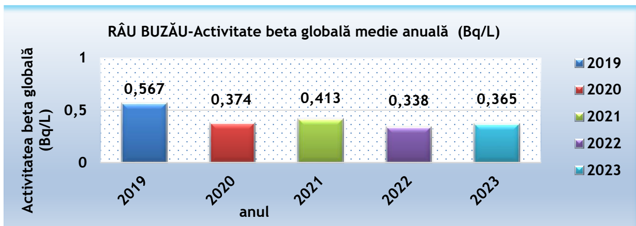
Figura IX.1.2.1.3. Activitatea specifică beta globală medie anuală pentru apa de Râu Buzău (valori imediate), comparativ în perioada 2019-2023
