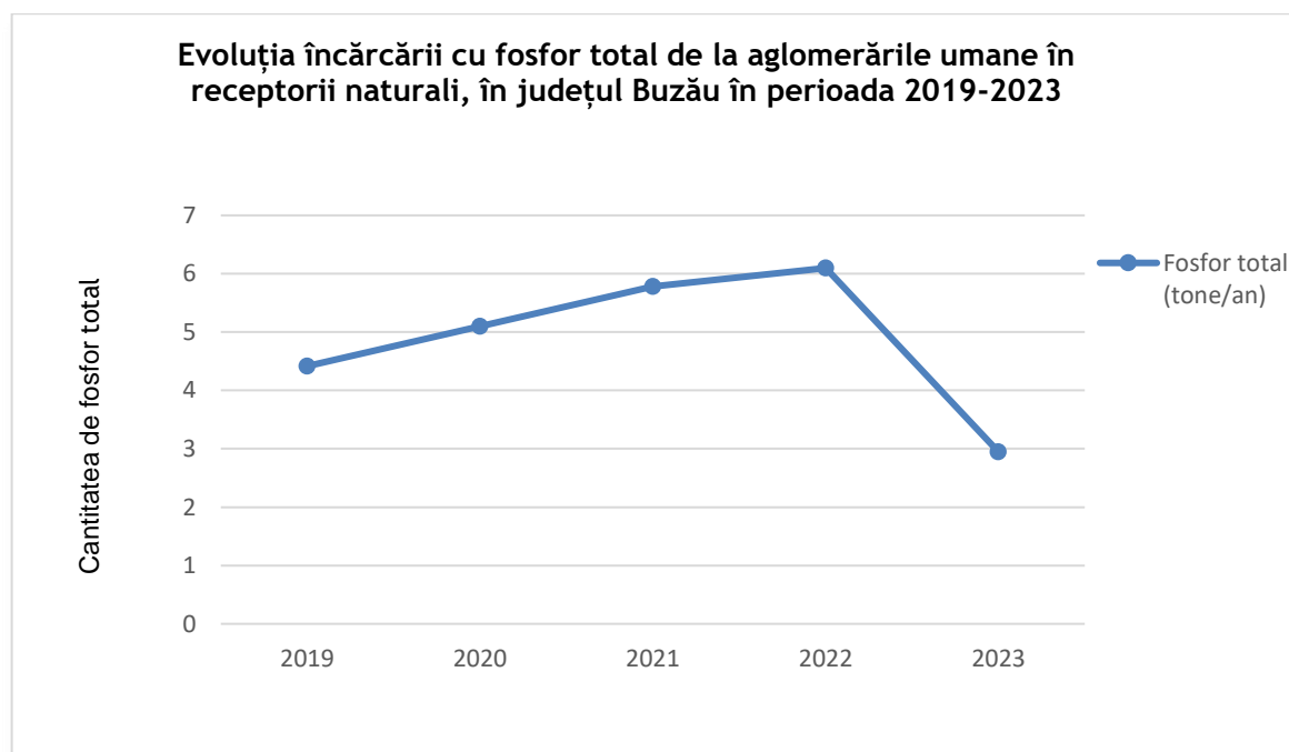
Figura II.2.2.2.5. Evoluția încărcării cu fosfor total de la aglomerările umane în receptori naturali, în județul Buzău în perioada 2019-2023
