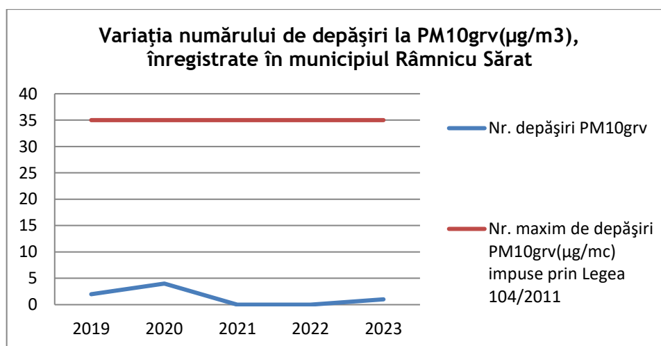
Fig. I.1.1.3.3. Variația numărului de depășiri la PM10 gravimetric în Râmnicu Sărat
