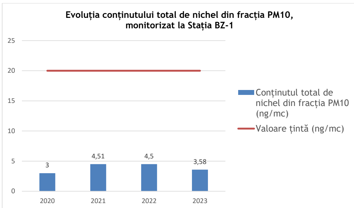
Figura I.1.1.2.9.1. Evoluția conținutului de nichel din fracția PM10, mediat pe un an calendaristic
