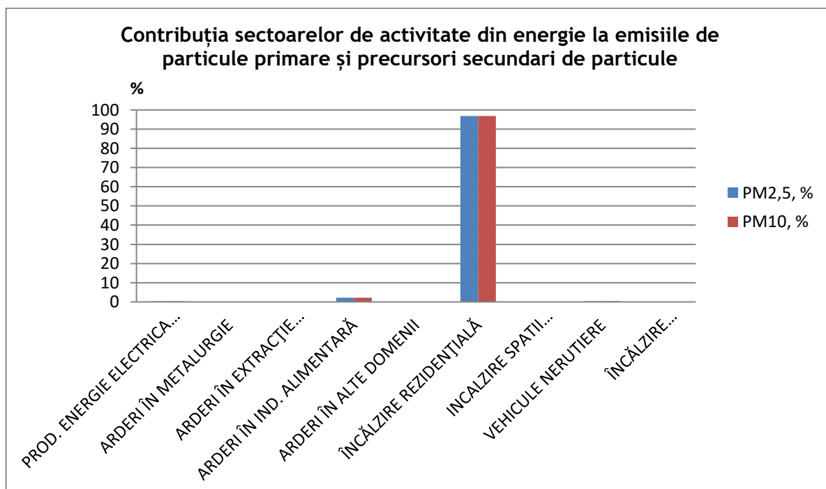
Figura I.2.1.1.3. Contribuția sectoarelor de activitate din energie la emisiile de particule primare și precursori secundari de particule
