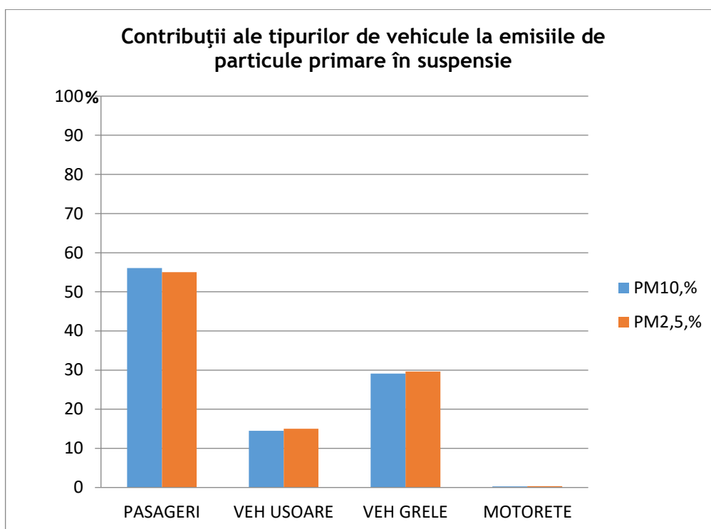
Figura I.2.1.3.5. Contribuția tipurilor de vehicule la emisiile de particule primare și precursori secundari de particule în județul Buzău în anul 2023
