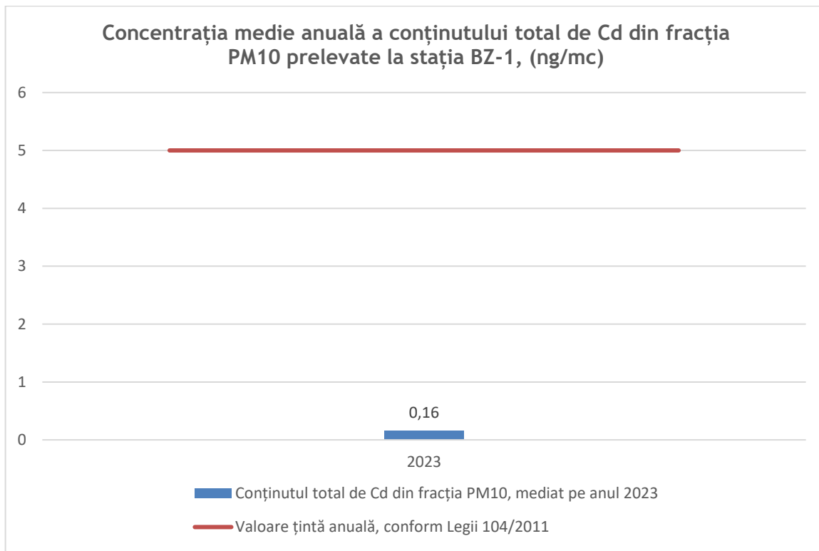
Fig. I.1.1.1.7.3. Concentrația medie anuală a conținutului total de Cd din fracția PM10 prelevate la stația BZ-1, pentru anul 2023 (ng/mc)
