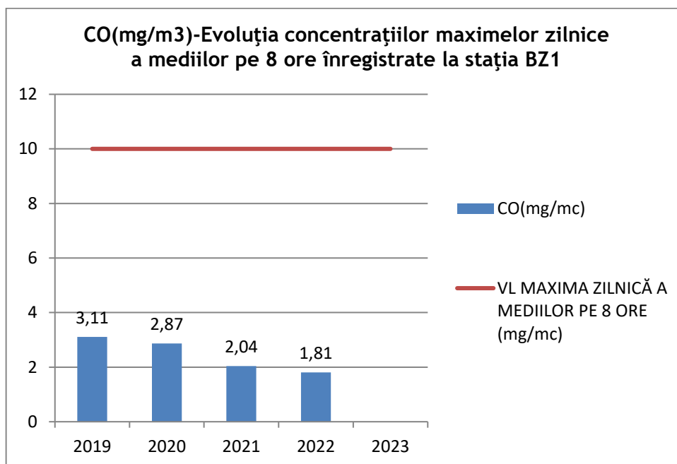
Fig. I.1.1.2.4.1. Evoluția concentrațiilor maximelor zilnice a mediilor pe 8 ore CO la stația BZ-1
