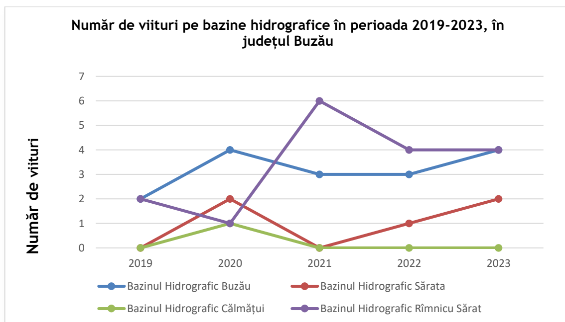
Figura II.1.1.3.1. Număr de viituri pe principalele cursuri de apă din județul Buzău în perioada 2019-2023 în județul Buzău
