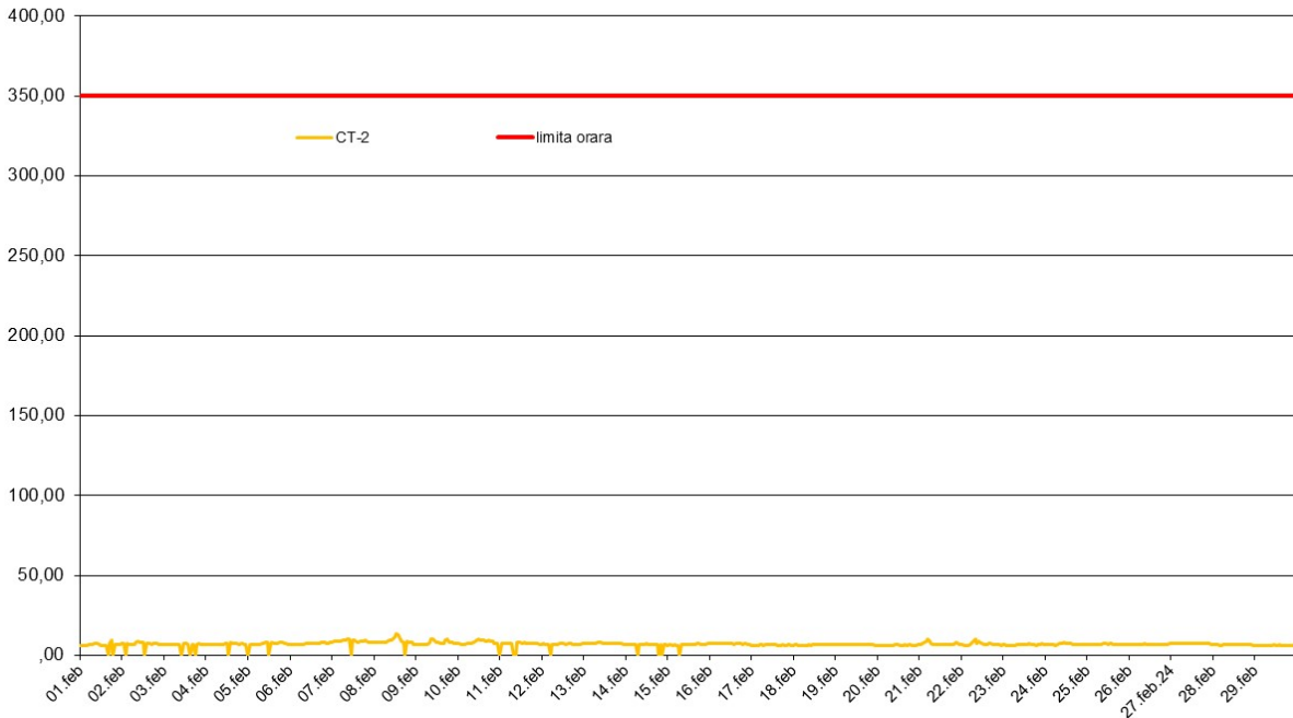
SO 2 (ug/m 3 ), perioada: 01 - 29 Februarie 2024 - Date validate
