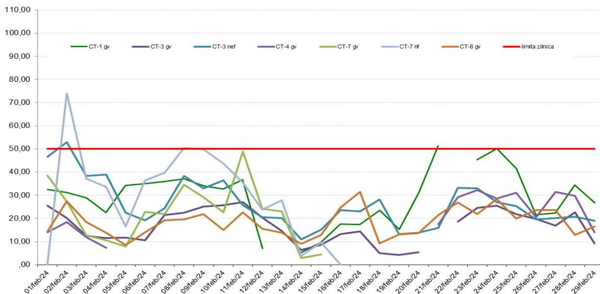
PM10 nef și PM10 gv (ug/m3), perioada: 01 - 29 Februarie 2024 - Date validate
