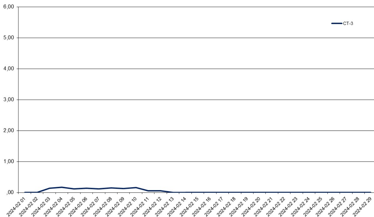
Benzen (ug/ m3), perioada: 01 - 29 Februarie 2024 - Date validate
