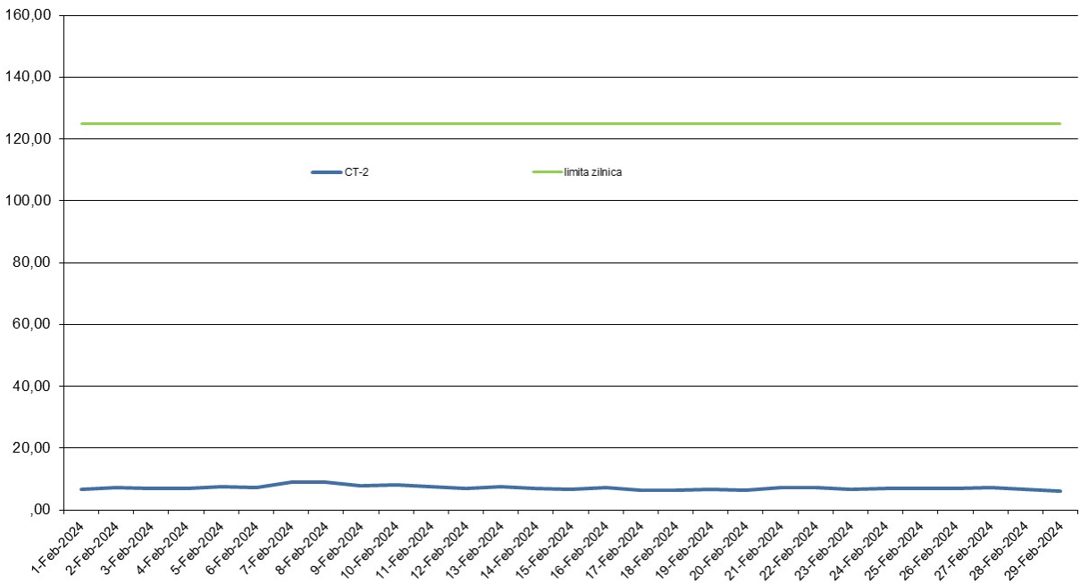
SO 2 (ug/m 3 ), perioada: 01 - 29 Februarie 2024 - Date validate
