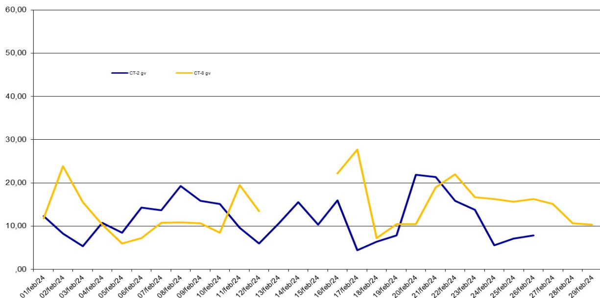
PM2.5 gv (ug/m3), perioada: 01 - 29 Februarie 2024 - Date validate
