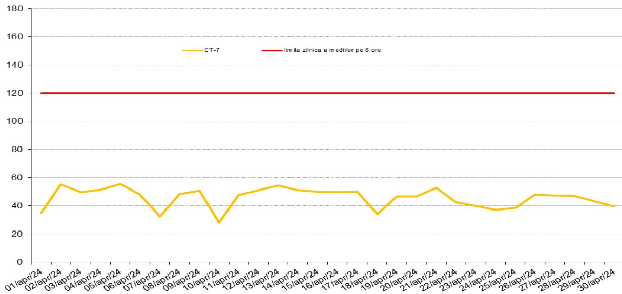
O3 (mg/m3) - maximul zilnic medie mobila perioada: 01 - 30 Aprilie 2024 - date validate
