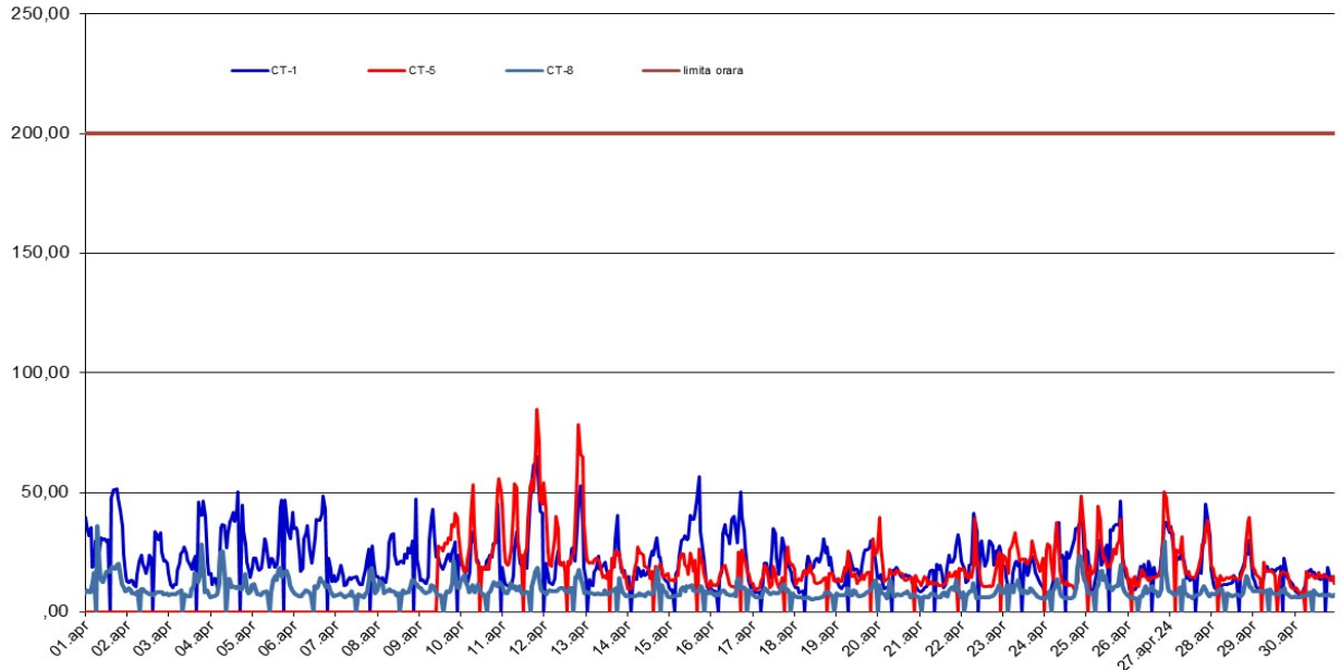
NO2 (ug/m3), perioada: 01 - 30 Aprilie 2024 - Date validate
