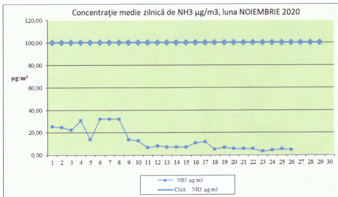
Figura 2. Evoluția concentrației medii zilnice de \text{NH}_3
