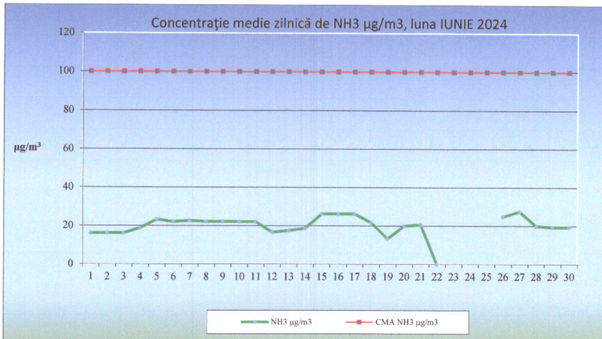
Figura 3. Evoluția concentrației medii zilnice de NH 3
