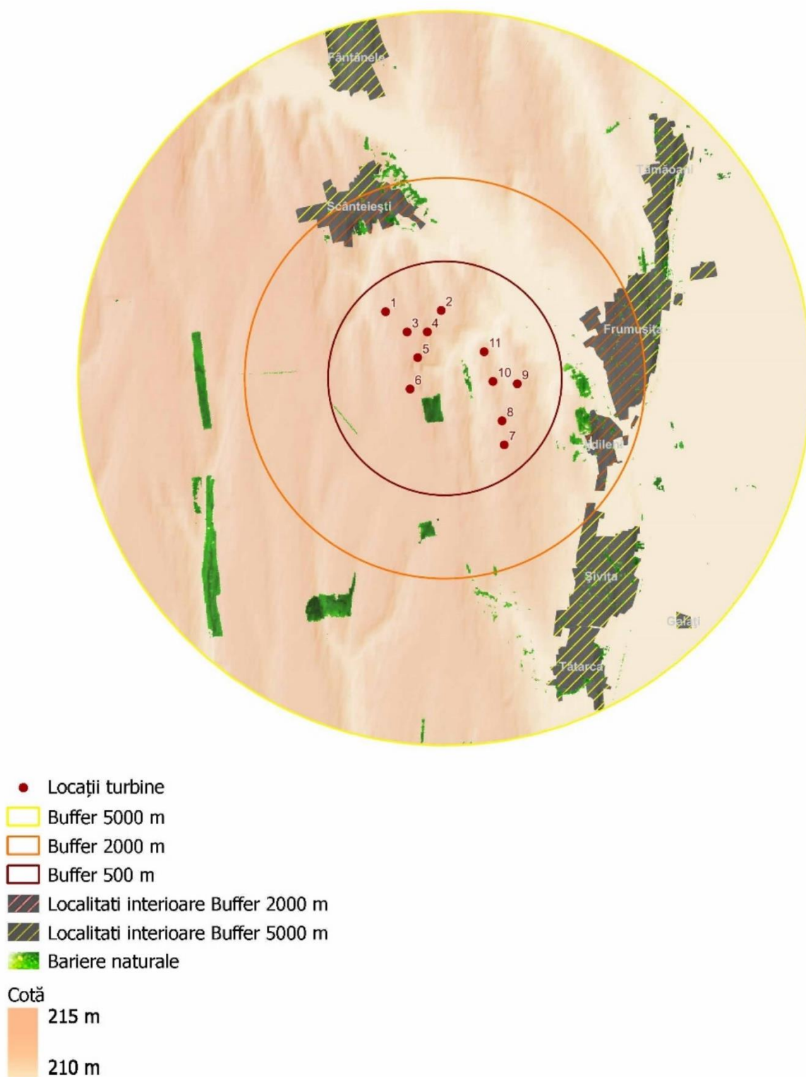
Figura 1. Amplasament turbine
