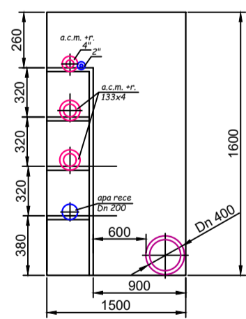
Sectiune standard tunel tehnic
