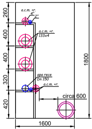
Sectiune standard tunel tehnic
