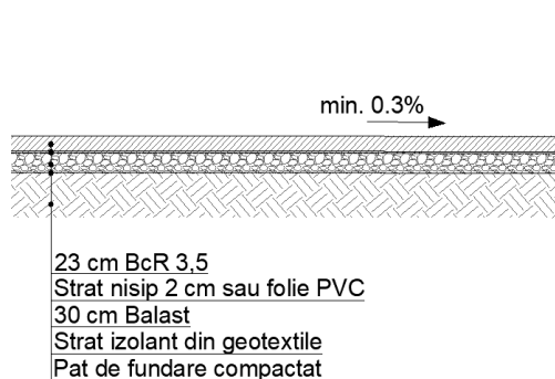
fig.1 Detaliu alcătuire
