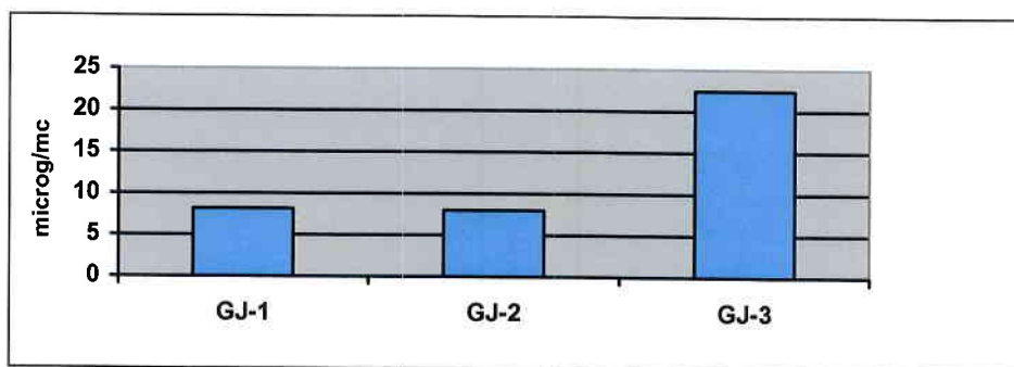
Fig. 6 Medii anuale SO 2 stații automate, anul 2017
