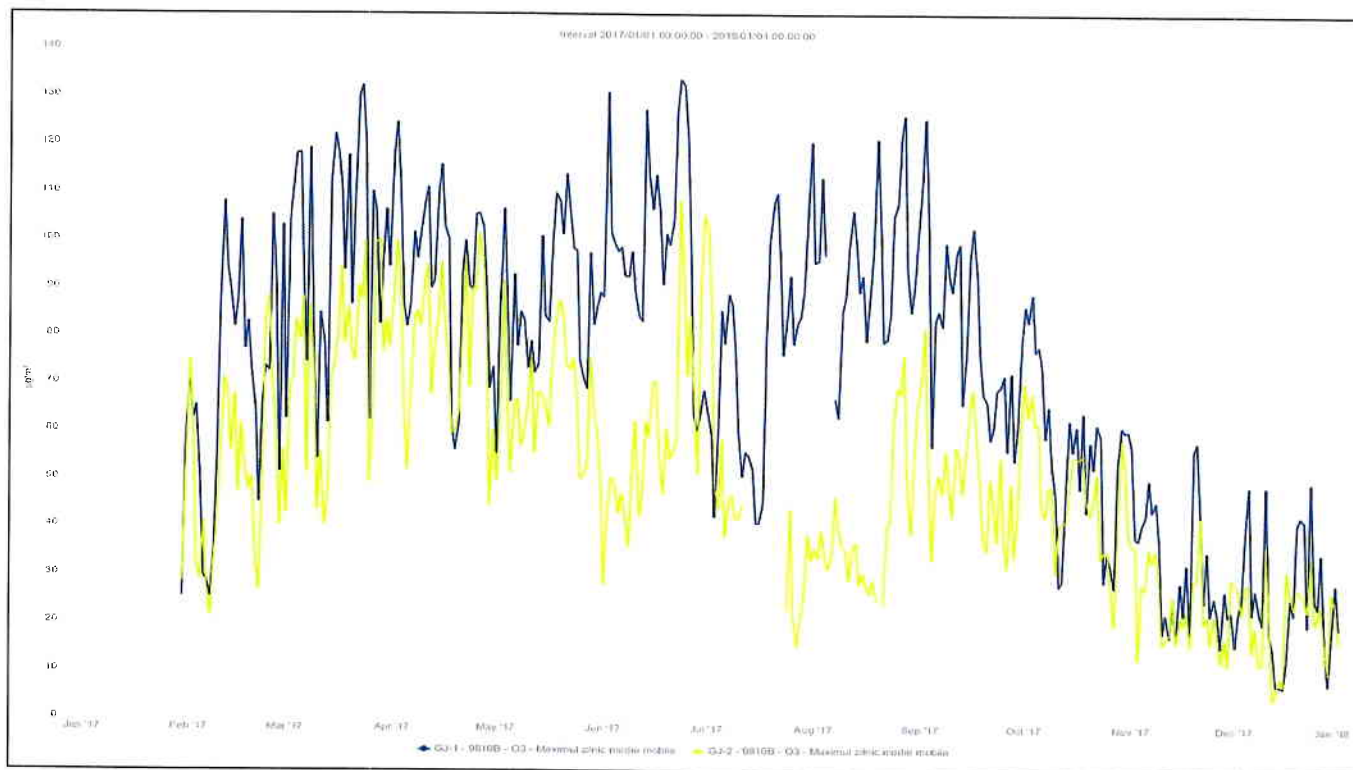
Fig. 10. Medii mobile ozon, anul 2017
