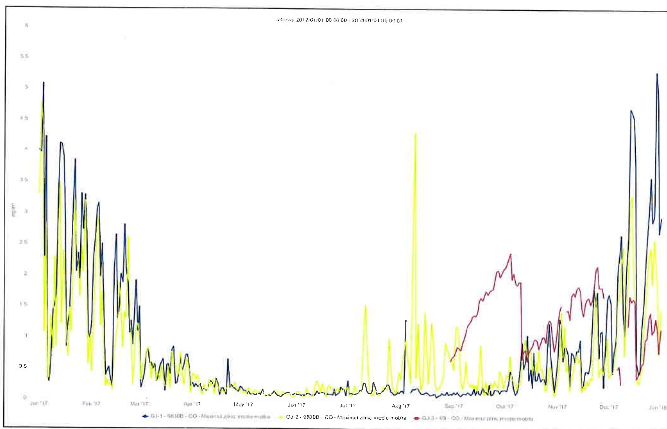
Fig. 9. Medii mobile CO, anul 2017
