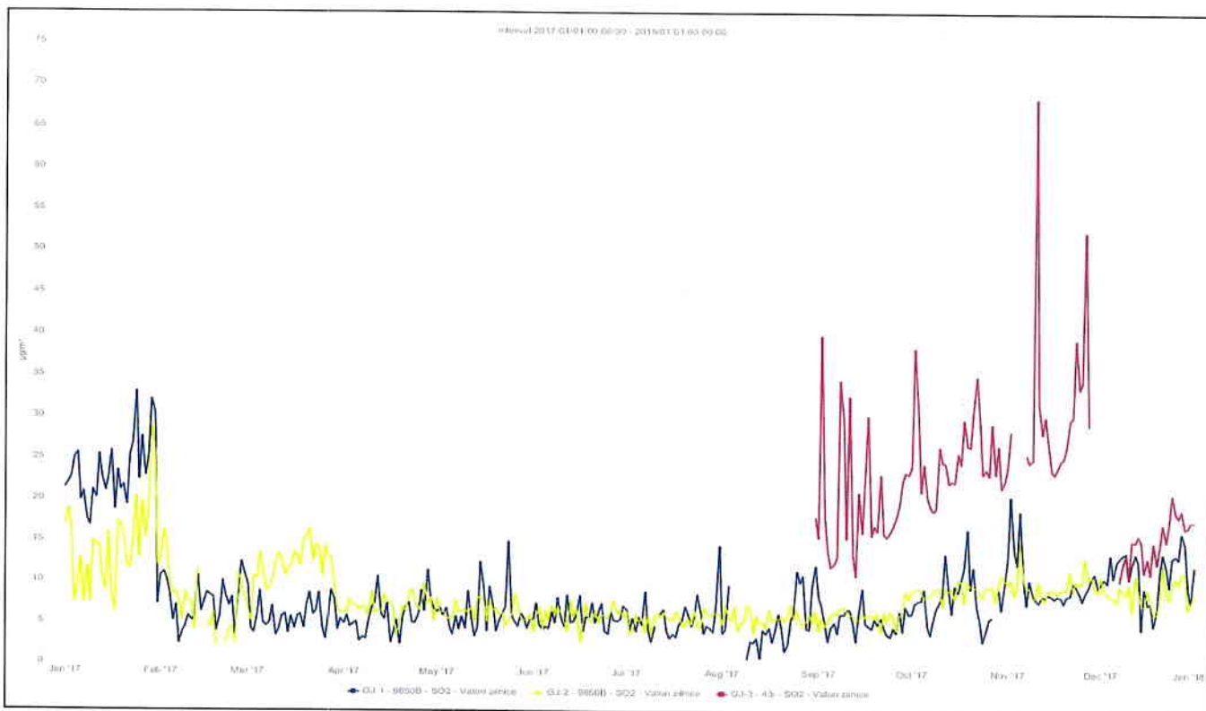
Fig. 5. Medii zilnice SO 2 anul 2017
