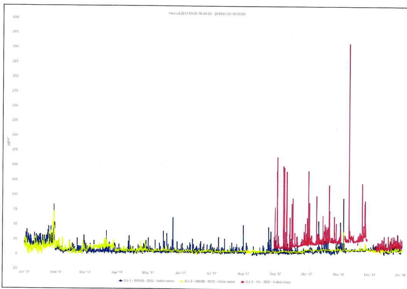
Fig. 4. Medii orare \text{SO}_2 anul 2017
