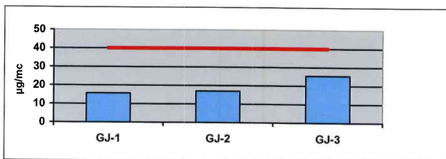
Fig. 3. Medii anuale NO 2 anul 2017
