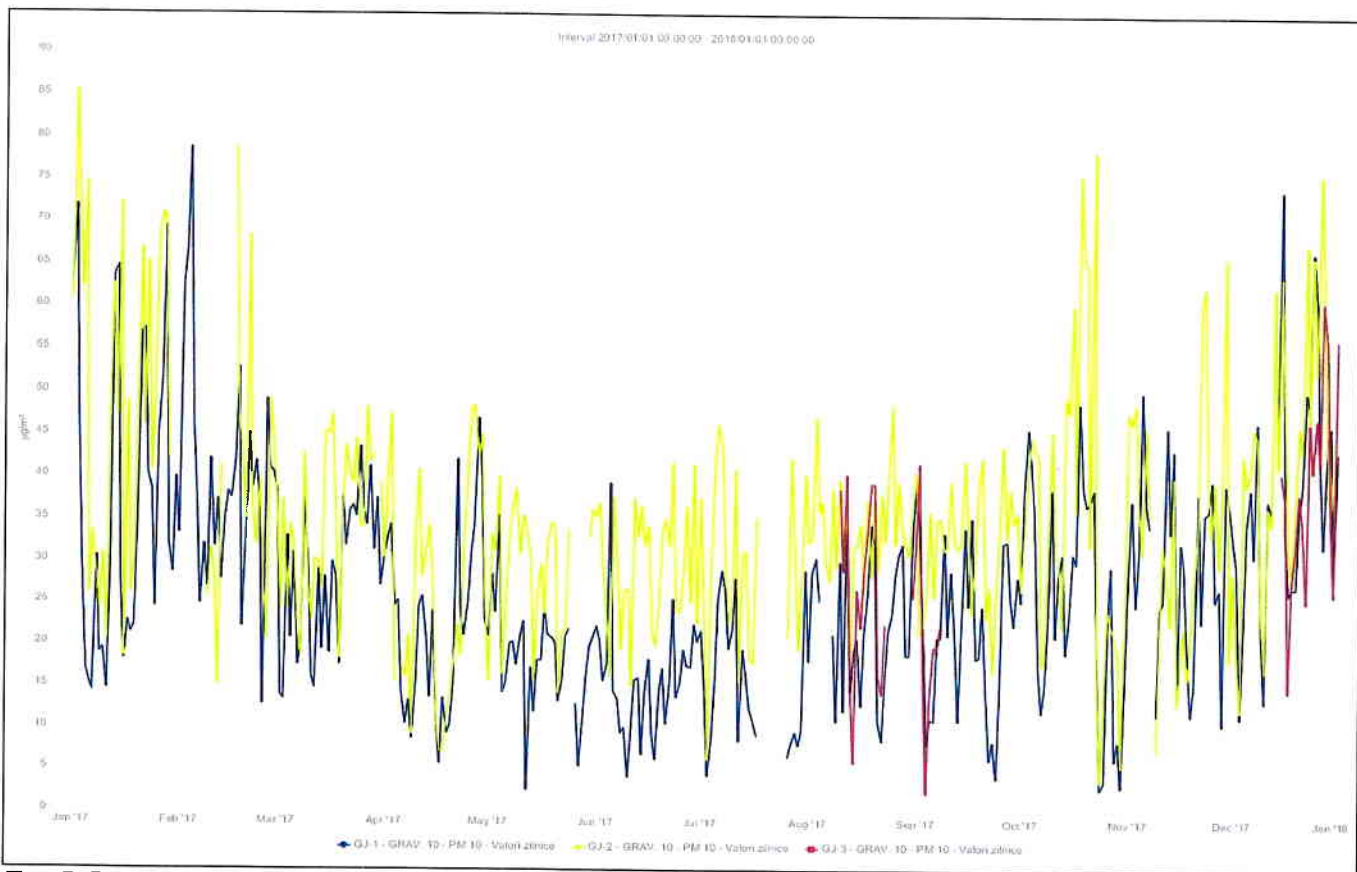
Fig. 7. PM10 gravimetric, medii zilnice, anul 2017
