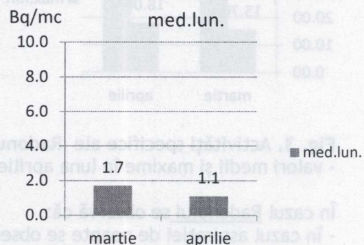
Fig. 2. Aerosoli atmosferici, activități specifice beta globale imediate - valori medii și maxime în luna aprilie, comparativ cu luna martie
