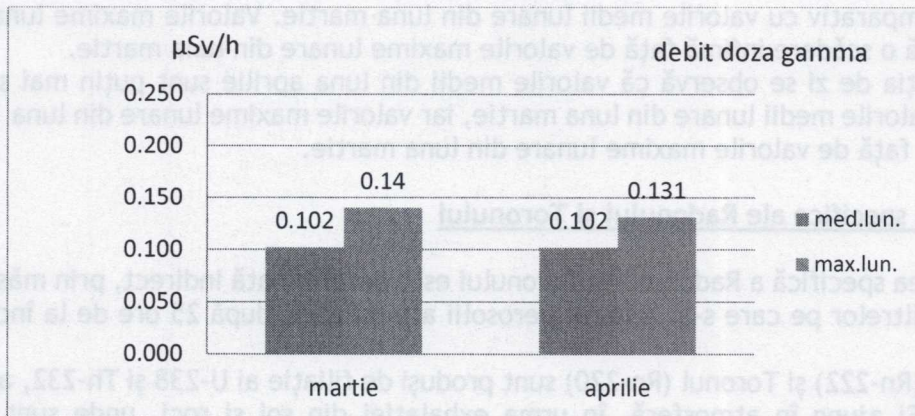
Fig. 1. Debitul dozei gama în aer ( \mu\text{Sv/h} ) - valori medii și maxime în luna aprilie comparativ cu luna martie
