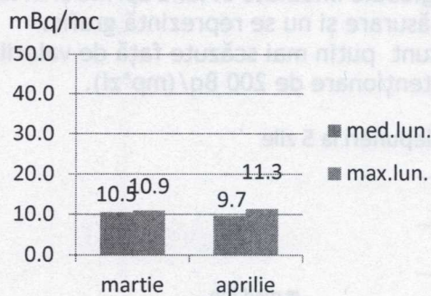
Fig. 5. Aerosoli atmosferici, activități specifice beta globale întârziate (la 5 zile) - valori medii și maxime în luna aprilie, comparativ cu luna martie
