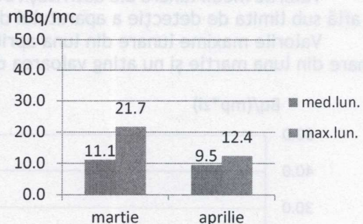
Fig. 5. Aerosoli atmosferici, activități specifice beta globale întârziate (la 5 zile) - valori medii și maxime în luna aprilie, comparativ cu luna martie
