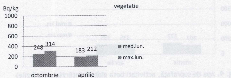
Fig. 11. Vegetație spontană, activitati beta globale întârziate (la 5 zile)
