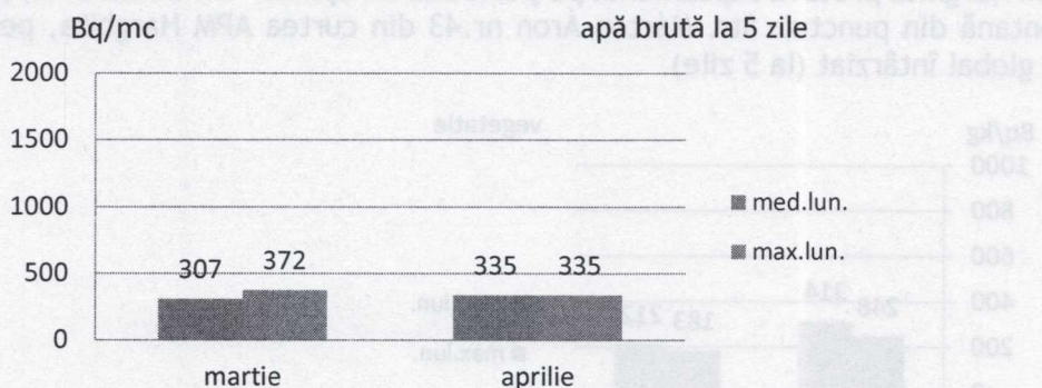
Fig. 9. Apa de suprafață, activitati beta globale întârziate (la 5 zile) - valori medii și maxime în luna aprilie, comparativ cu luna martie
