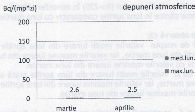
Fig. 6. Depuneri atmosferice, activitati beta globale immediate - valori medii și maxime în luna aprilie, comparativ cu luna martie
