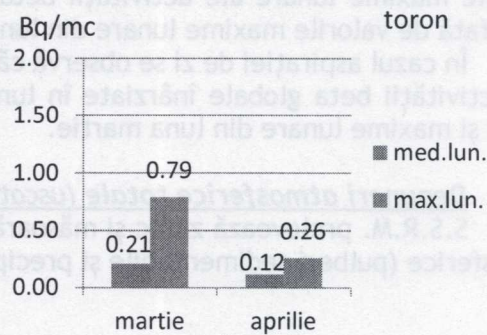
Fig. 4. Activități specifice ale Toronului (Rn-220) în atmosfera liberă medii lunare și maxime zilnice în luna aprilie comparativ cu luna martie
