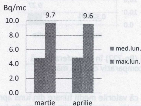
Fig. 2. Aerosoli atmosferici, activități specifice beta globale imediate - valori medii și maxime în luna aprilie, comparativ cu luna martie
