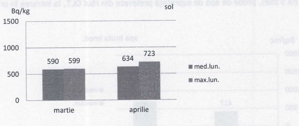
Fig. 10. Sol necultivat, activitati beta globale întârziate (la 5 zile)
