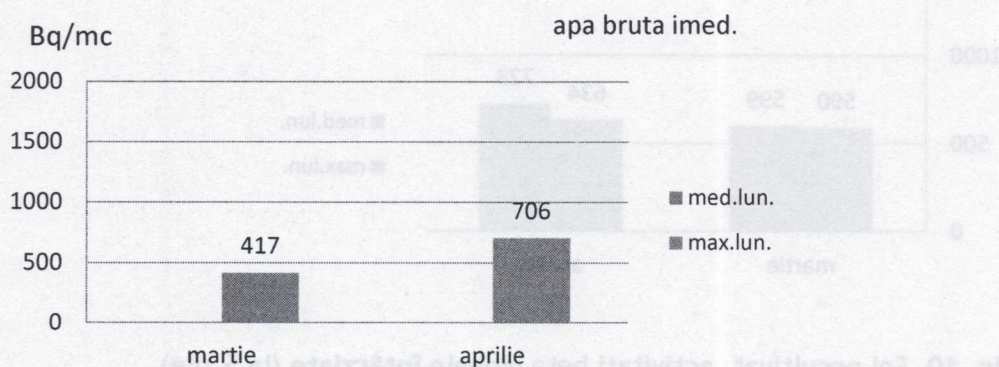
Fig. 8. Apa de suprafață, activitati beta globale imediate - valori medii și maxime în luna aprilie, comparativ cu luna martie
