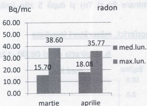
Fig. 3. Activități specifice ale Radonului (Rn-222) în atmosfera liberă - valori medii și maxime în luna aprilie, comparativ cu luna martie
