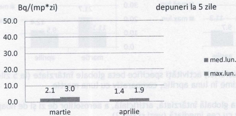
Fig. 7. Depuneri atmosferici, activități beta globale întârziate (la 5 zile) - valori medii și maxime în luna aprilie, comparativ cu luna martie
