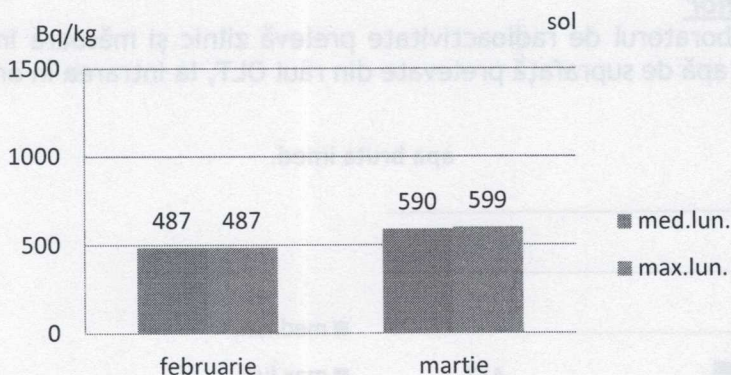
Fig. 10. Sol necultivat, activitati beta globale întârziat (la 5 zile)
