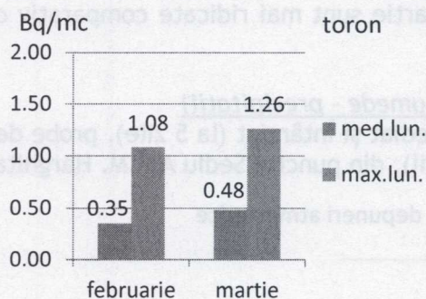
Fig. 4. Activități specifice ale Toronului (Rn-220) în atmosfera liberă medii lunare și maxime zilnice în luna martie, comparativ cu luna februarie
