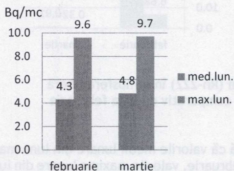
Fig. 2. Aerosoli atmosferici, activități specifice beta globale imediate - valori medii și maxime în luna martie, comparativ cu luna februarie
