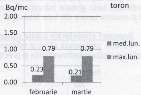
Fig. 4. Activități specifice ale Toronului (Rn-220) în atmosfera liberă medii lunare și maxime zilnice în luna martie, comparativ cu luna februarie
