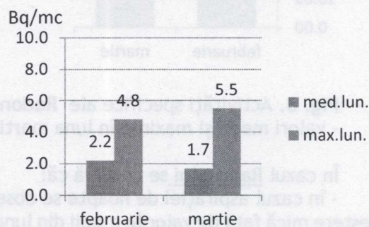
Fig. 2. Aerosoli atmosferici, activități specifice beta globale imediate - valori medii și maxime în luna martie, comparativ cu luna februarie
