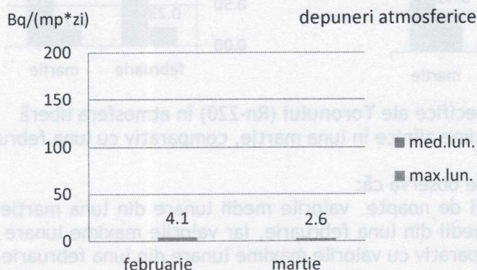
Fig. 6. Depuneri atmosferice, activitati beta globale imediate - valori medii și maxime în luna martie, comparativ cu luna februarie
