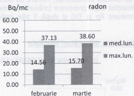
Fig. 3. Activități specifice ale Radonului (Rn-222) în atmosfera liberă - valori medii și maxime în luna martie, comparativ cu luna februarie
