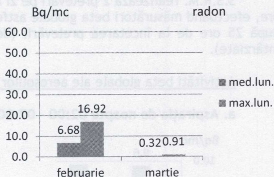
Fig. 3. Activități specifice ale Radonului (Rn-222) în atmosfera liberă - valori medii și maxime în luna martie, comparativ cu luna februarie
