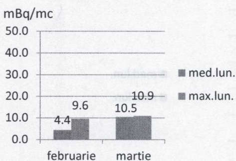
Fig. 5. Aerosoli atmosferici, activități specifice beta globale întârziate (la 5 zile) - valori medii și maxime în luna martie, comparativ cu luna februarie
