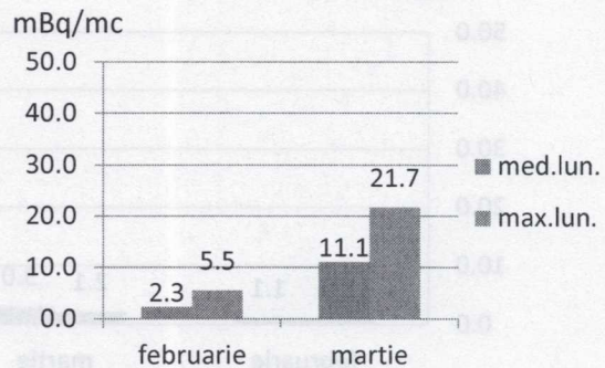
Fig. 5. Aerosoli atmosferici, activități specifice beta globale întârziate (la 5 zile) - valori medii și maxime în luna martie, comparativ cu luna februarie
