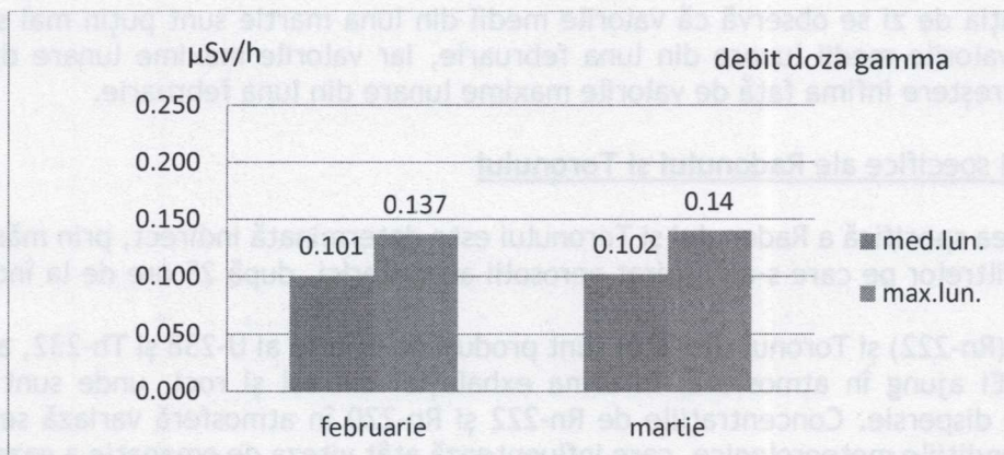
Fig. 1. Debitul dozei gama în aer ( \mu\text{Sv/h} ) - valori medii și maxime în luna martie comparativ cu luna februarie
