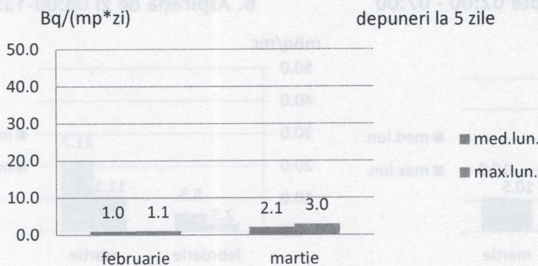
Fig. 7. Depuneri atmosferici, activități beta globale întârziate (la 5 zile) - valori medii și maxime în luna martie, comparativ cu luna februarie
