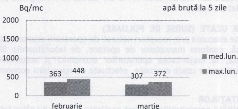
Fig. 9. Apa de suprafață, activități beta globale întârziate (la 5 zile)
