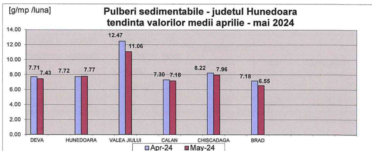
Fig. nr. 1.2.1.1. Evoluția calității pulberilor sedimentabile în perioada Aprilie 2024 - Mai 2024
