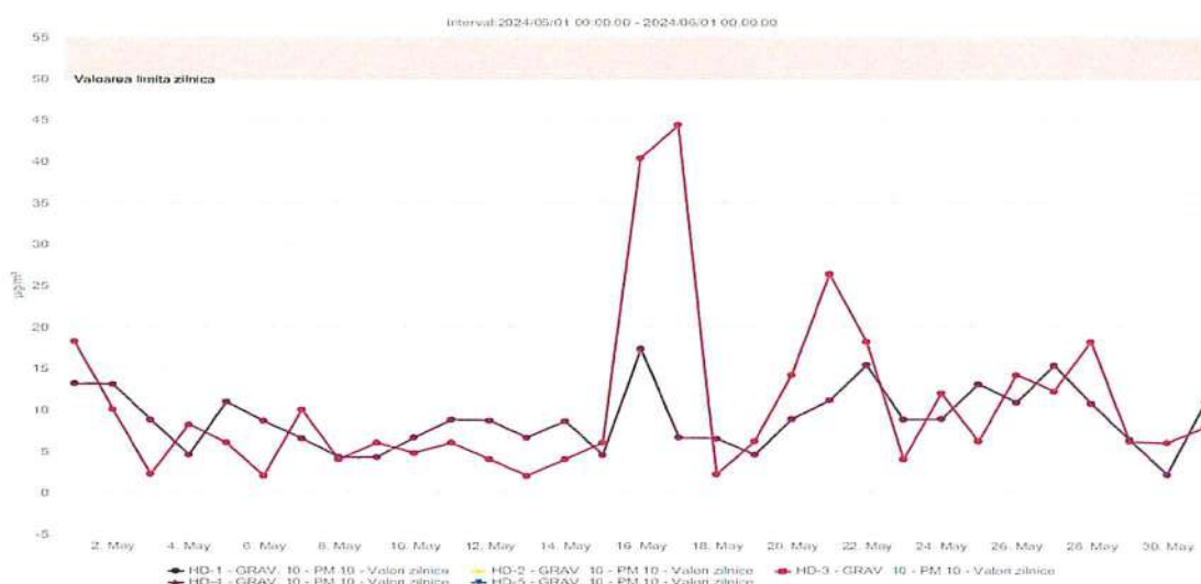
Figura nr. 1.3.8. Evoluția zilnică a valorilor de \text{PM}_{10} ( \mu\text{g}/\text{mc} ) determinat gravimetric, în luna mai 2024, la stațiile automate de monitorizare
