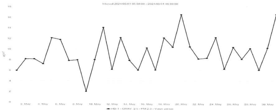
Figura nr. 1.3.8. Evoluția zilnică a valorilor de PM 2.5 (µg/mc) determinat gravimetric, în luna mai 2024, la stația automata de monitorizare HD-1
