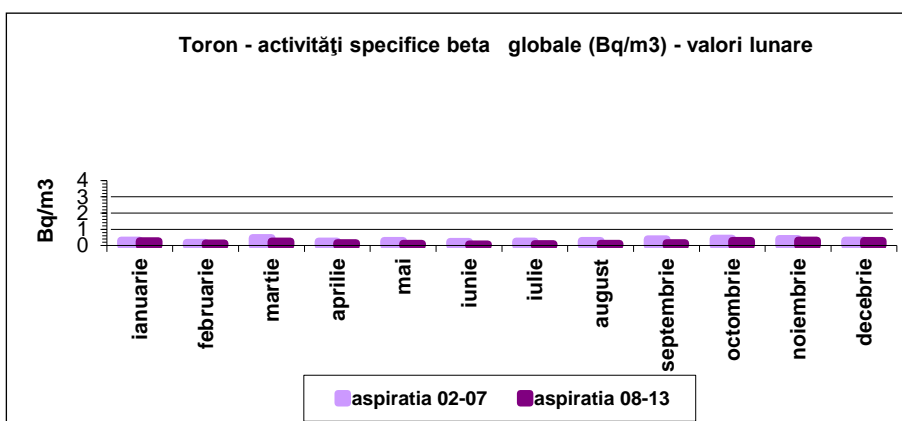
Fig. IX. 1.1.7 - Valori lunare ale activității beta globale-2023
