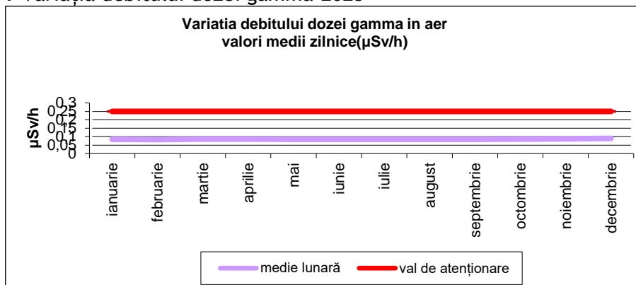
Fig.IX.1.1.1-Variația debitului dozei gamma-2023
