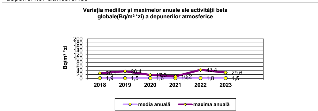
Fig.IX.1.1.10 - Variația mediilor și maximelor anuale ale activității beta globale a depunerilor atmosferice
