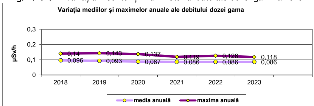
Fig.IX.1.1.2 - Variația mediilor și maximelor anuale ale dozei gamma 2018 - 2023
