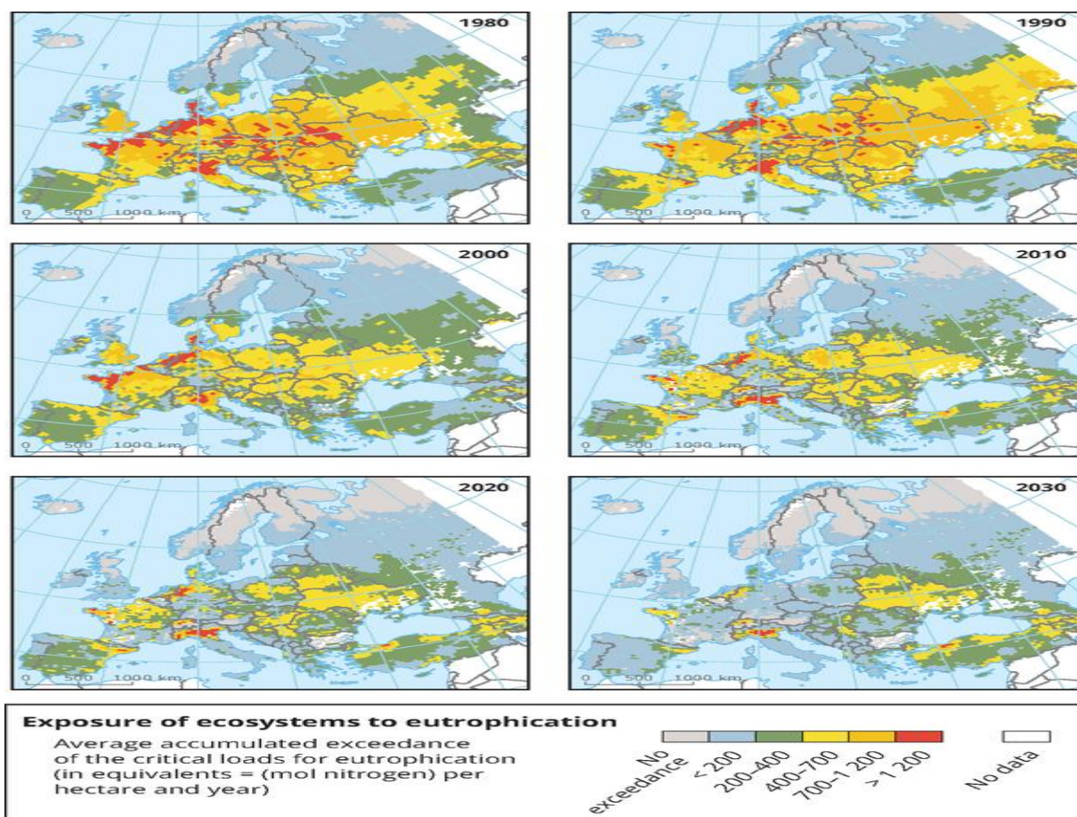
Figura I.1.2.2.2 Expunerea la eutrofizare în unele state din Europa (sursa: https://ec.europa.eu/eurostat/web/environment/environmental-indicator-catalogue )
