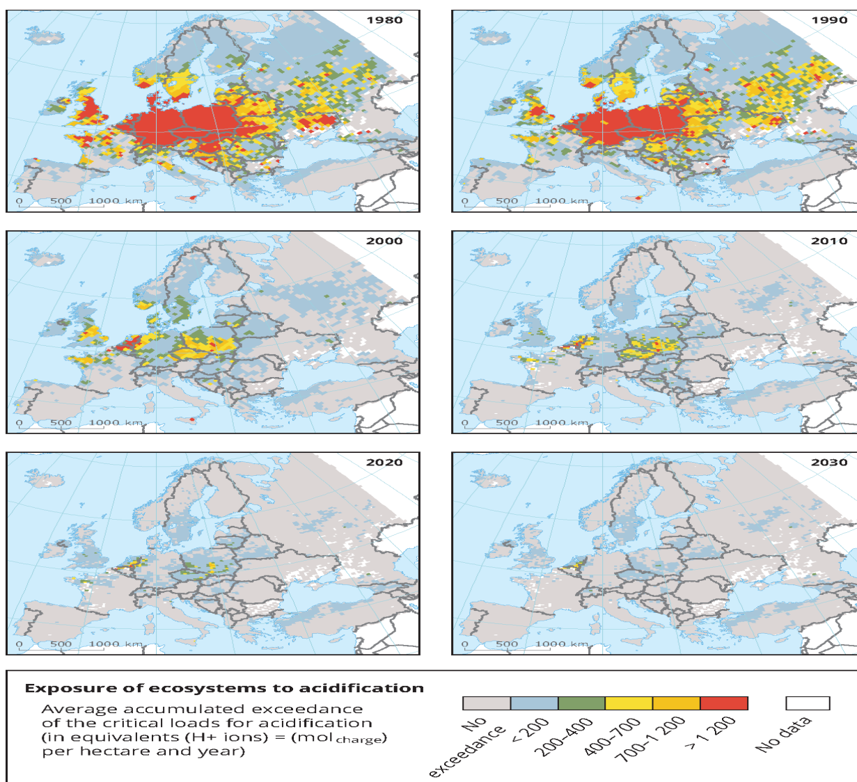
Figura I.1.2.2.1 Expunerea la acidifiere în unele state din Europa
