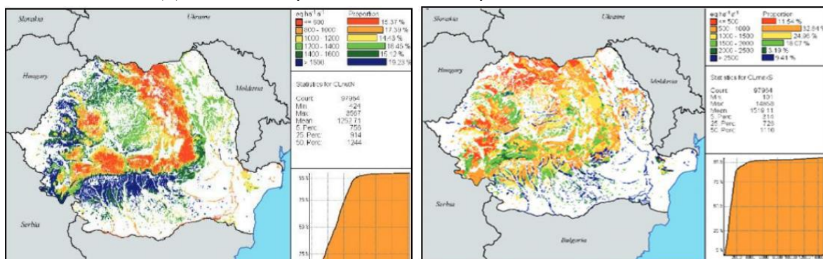
Figura I.1.2.3.1. Încărcări critice la acidifiere CL max(S) în România pentru ecosistemul păduri
