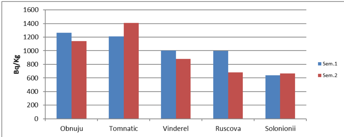
Figura IX.2.4.2. Activități \beta -globale în soluri din zona Repedea și Poienile de sub Munte în anul 2023
