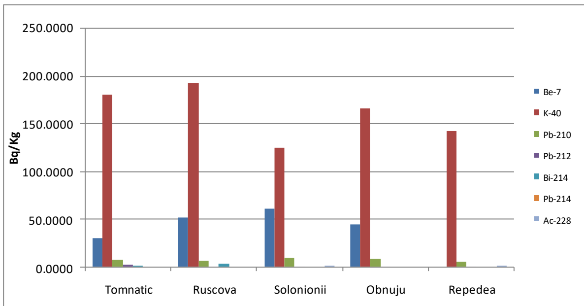
Figura IX.2.5.3. Nivelul activității radionuclizilor identificați în vegetație spontană din zona Repedeș și Poienile de sub Munte în anul 2023
