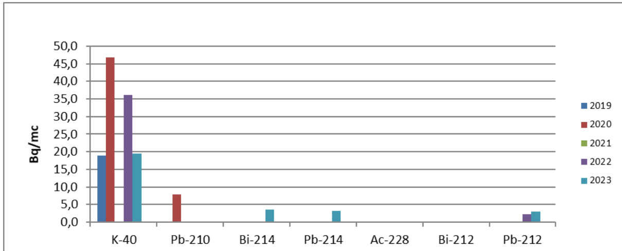
Figura IX.1.2.10. Evoluția activității celor mai frecvenți radionuclizi identificați pentru Baraj Firiza în perioada 2019 - 2023
