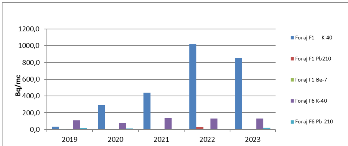
Figura IX.1.2.8. Evoluția activității celor mai frecvenți radionuclizi identificați pentru cele doua foraje în perioada 2019 - 2023
