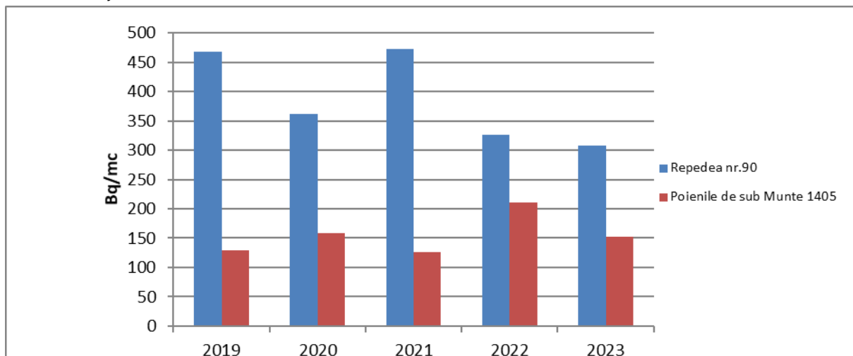
Figura IX.2.2.1. Activități \beta -globale imediate în fântânile monitorizate în zona Repedeș și Poienile de sub Munte în perioada 2019-2023
