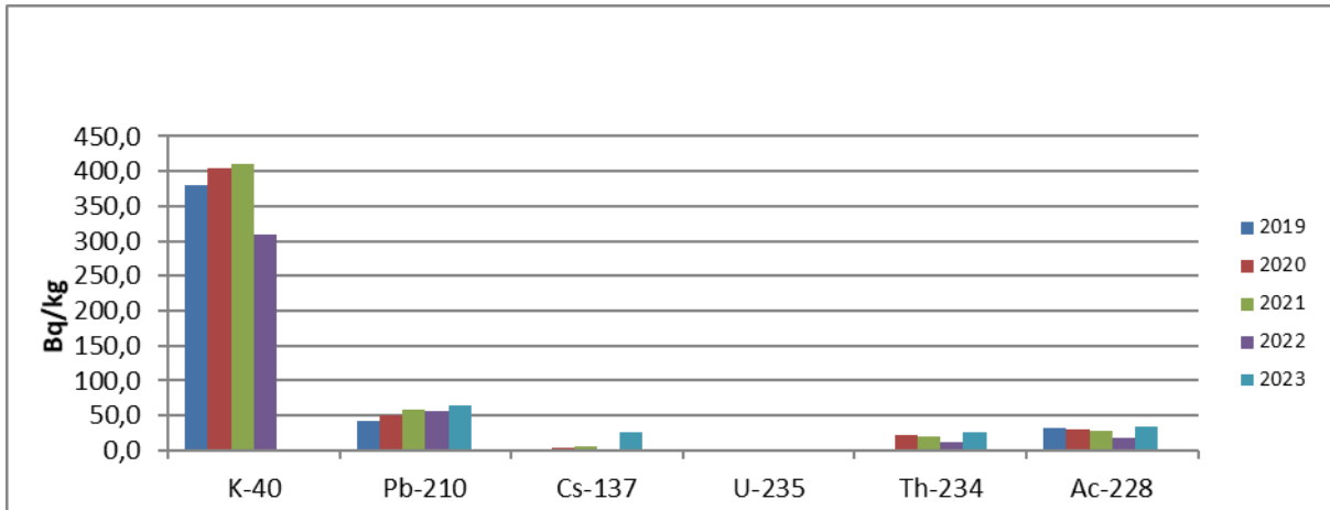
Figura IX.1.3.2. Evoluția activității celor mai frecvenți radionuclizi identificați pentru solul necultivat din Baia Mare
