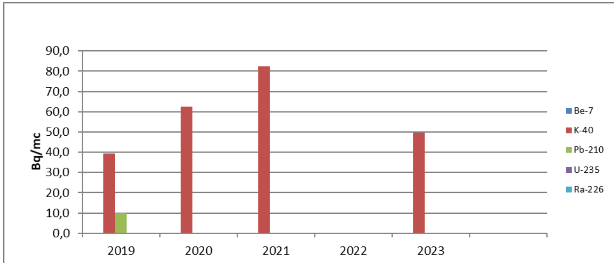
Figura IX.1.2.6. Evoluția activității celor mai frecvenți radionuclizi identificați pentru râul Tisa în perioada 2019-2023
