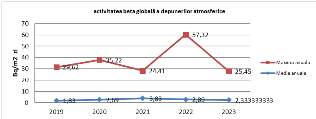
Figura IX.1.2.1. Variația mediilor și maximelor anuale ale activității beta Globale a depunerilor atmosferice totale
