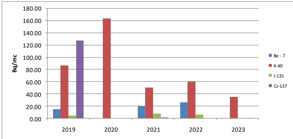
Figura IX.1.2.2. Evoluția activității celor mai frecvenți radionuclizi identificați pentru râul Săsar în perioada 2019 - 2023
