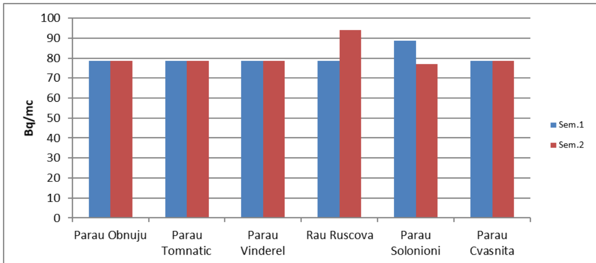
Figura IX.2.1.2. Măsurători \beta - globale pentru apa de suprafață în zona Repedeș și Poienile de sub Munte în anul 2023
