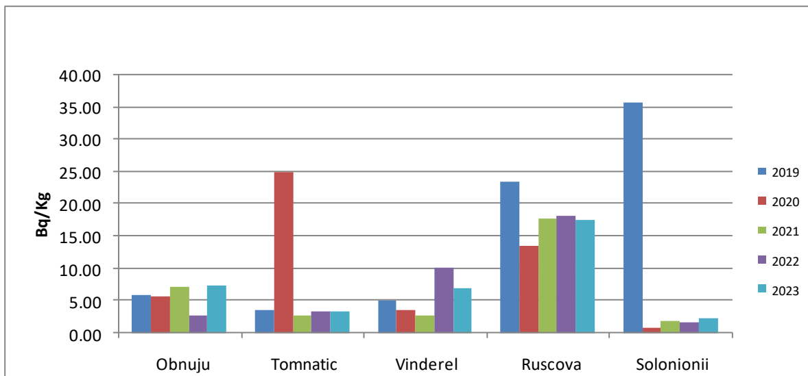
Figura IX.2.4.4. Nivelul activității Cs-137 în sol necultivat din zona Repede și Poienile de sub Munte în perioada 2019 - 2023
