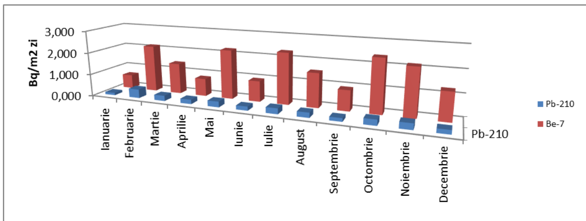
Figura IX.1.2.2. Variația activității specifice lunare a radionuclizilor naturali identificați în probele de depuneri atmosferice totale
