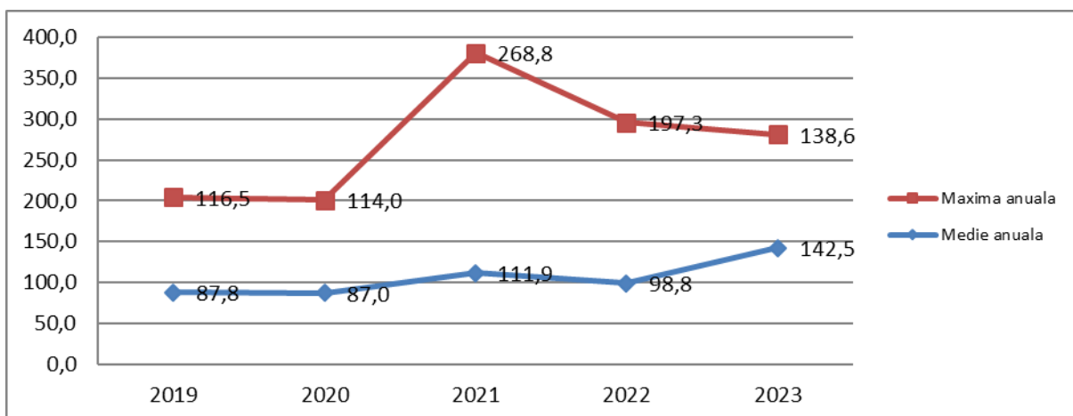
Figura IX.1.2.5. Variația mediilor și maximelor anuale ale activității beta globale a râului Tisa
