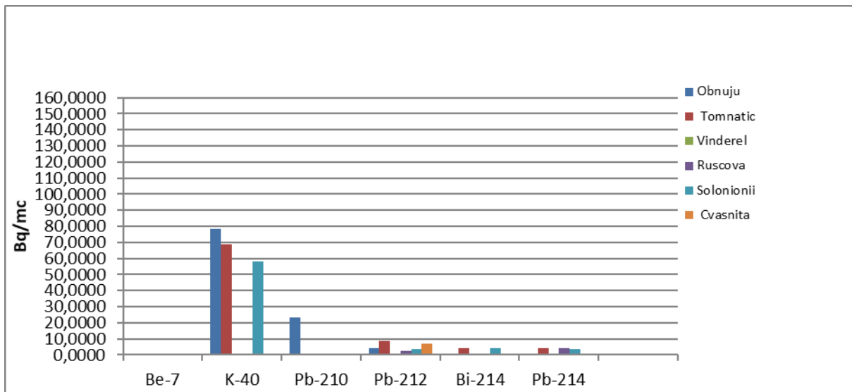
Figura IX.2.1.3. Nivelul activităților radionuclizilor identificați în apa de suprafață din zona Repedeș și Poienile de sub Munte în anul 2023
