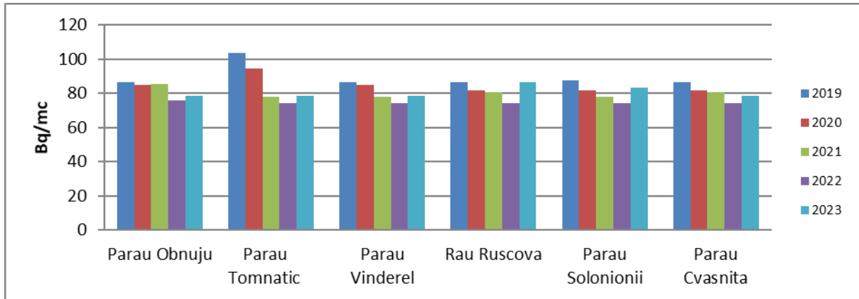
Figura IX.2.1.1. Activitatea \beta -globală pentru apa de suprafață în zona Repedeș și Poienile de sub Munte
