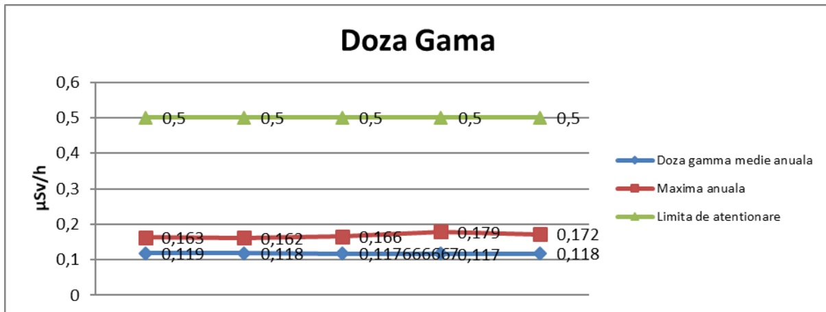
Figura IX.1.1.1.1. Variația mediilor și maximelor anuale ale debitului dozei gama
