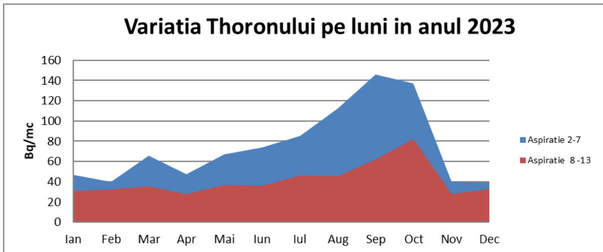
Figura IX.1.1.2.4. Variația activităților specifice medie anuală a toronului din atmosferă în funcție de variația diurnă
