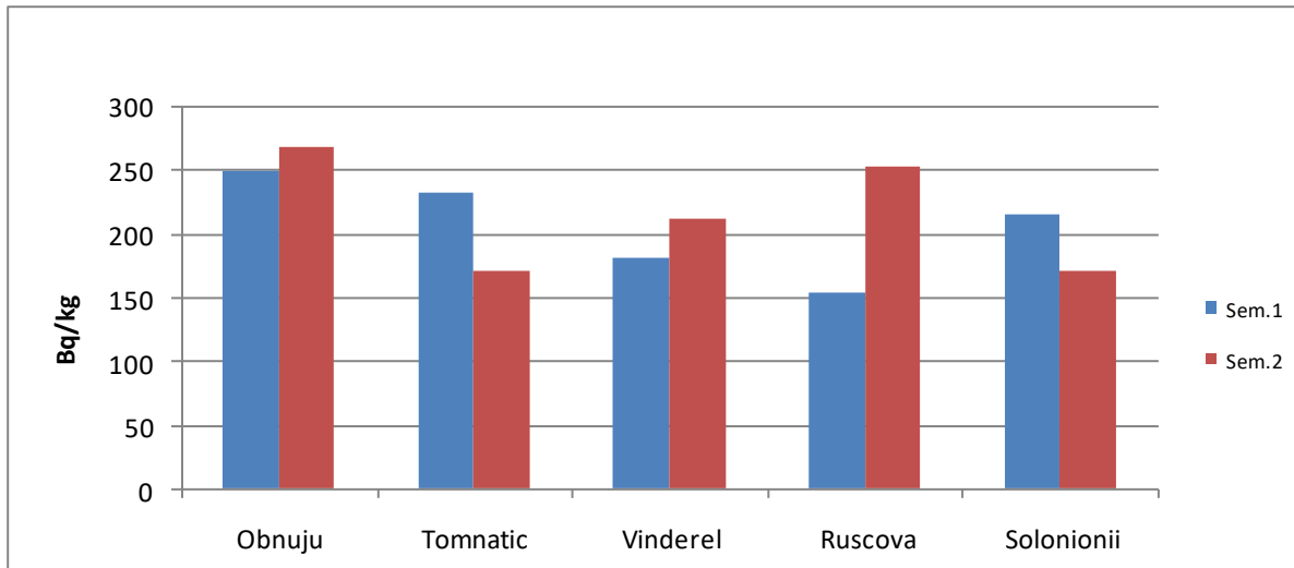
Figura IX.2.5.2. Activități \beta -globale în vegetație spontană din zona Repedeș și Poienile de sub Munte în anul 2023
