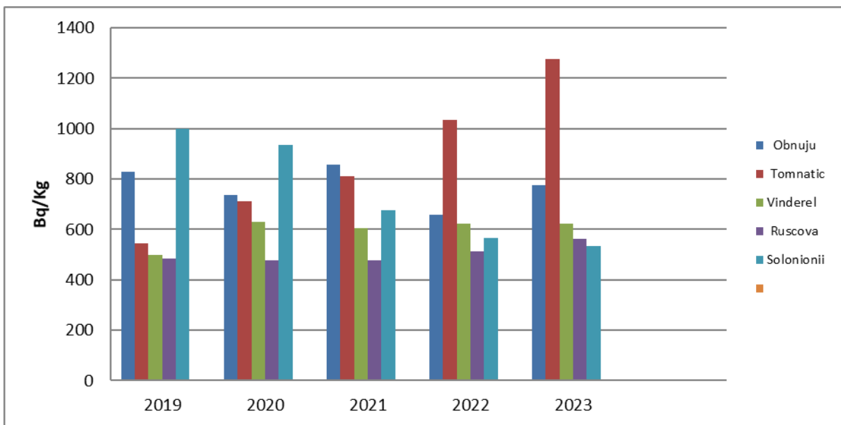
Figura IX.2.4.3. Nivelul activității K - 40 în sol necultivat din zona Repedea și Poienile de sub Munte în perioada 2019 - 2023
