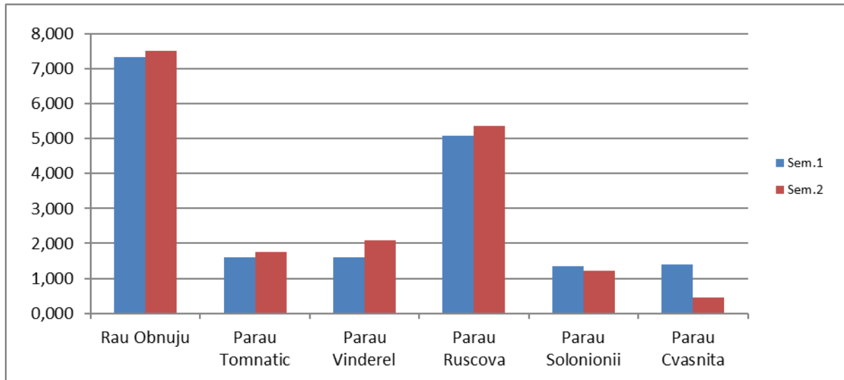
Figura IX.2.3.2. Nivelul activității Cs-137 în sedimente din zona Repedeș și Poienile de sub Munte în anul 2023
