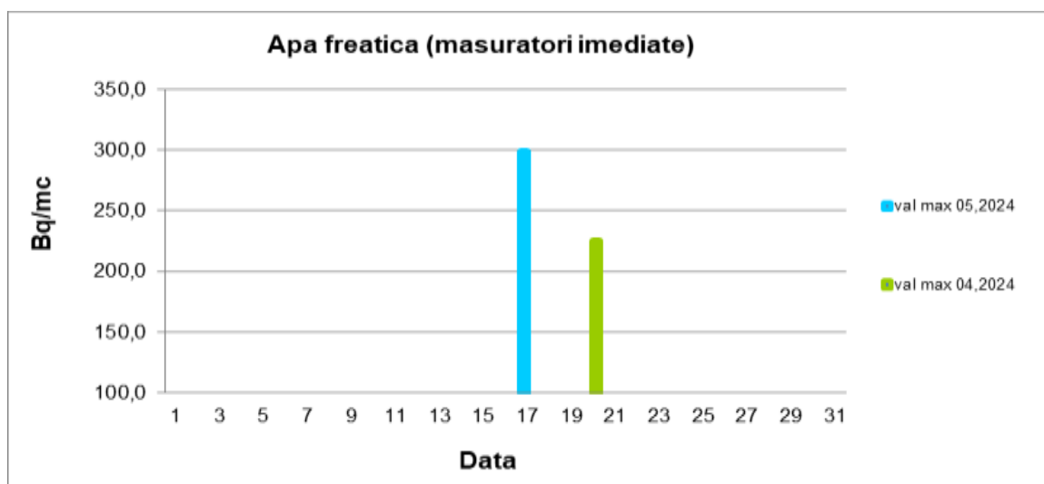
Graficul nr. 16.- apa freatică - activitate specifică beta globală
