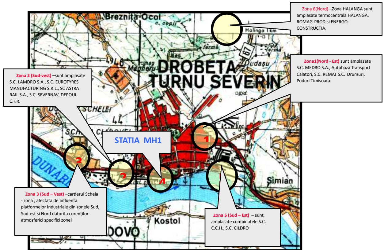
Figura nr 1-Amplasare Stație fixă automată - MH-1
