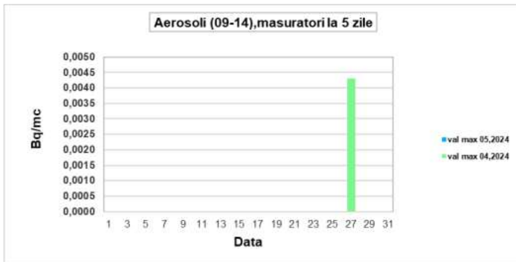
Graficul nr 11.- Aerosoli atmosferici - activitate specifică beta globală - intervalul 09-14
