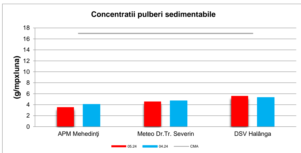
Graficul nr. 6 -Concentrațiile pulberilor sedimentabile
