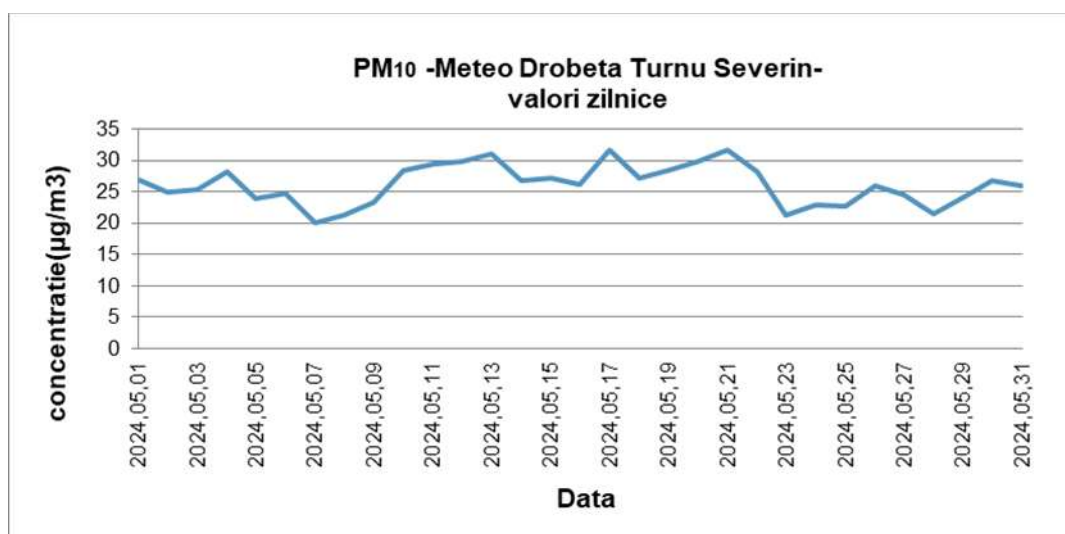
Graficul nr. 7. - Evoluția concentrațiilor medii zilnice pentru particule în suspensie (PM 10 )
