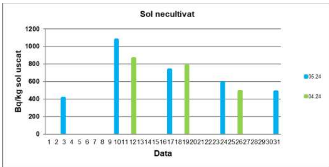
Graficul nr. 17- sol necultivat - activitate specifică beta globală
