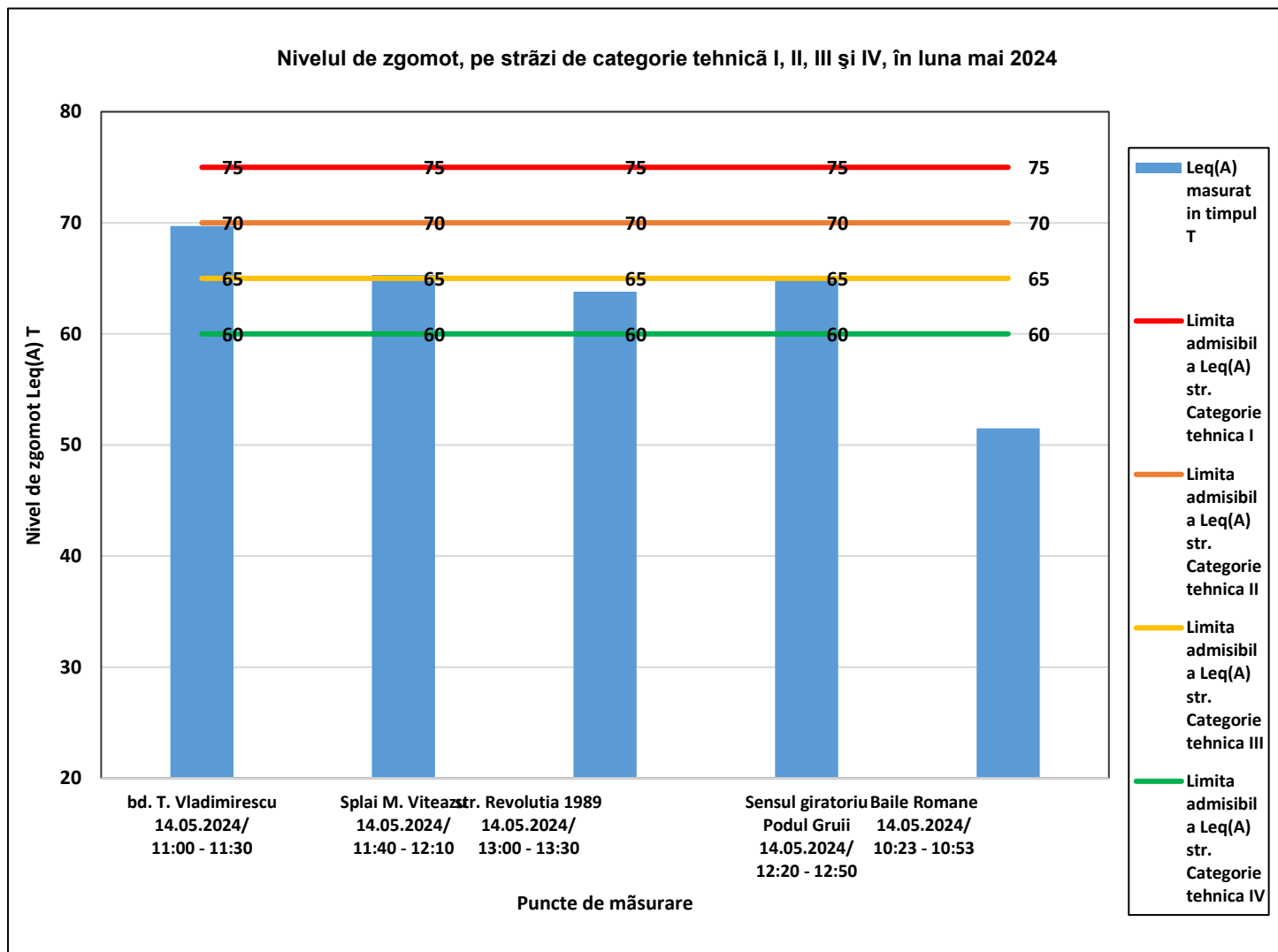
Graficul nr. 20- Nivelul de zgomot urban pe străzi de categorie tehnică I, II, III și IV, în municipiul Drobeta Turnu Severin, în luna mai 2024
