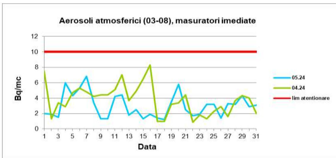
Graficul nr. 8.- Aerosoli atmosferici - activitate specifică beta globală - intervalul 03-08
