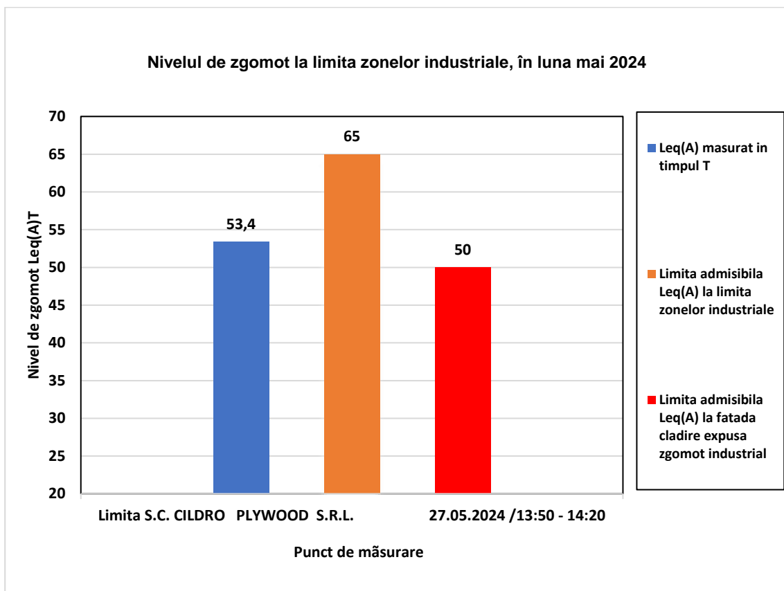
Graficul nr. 22- Nivelul de zgomot la limita zonelor industriale, din municipiul Drobeta Turnu Severin, în luna mai 2024
