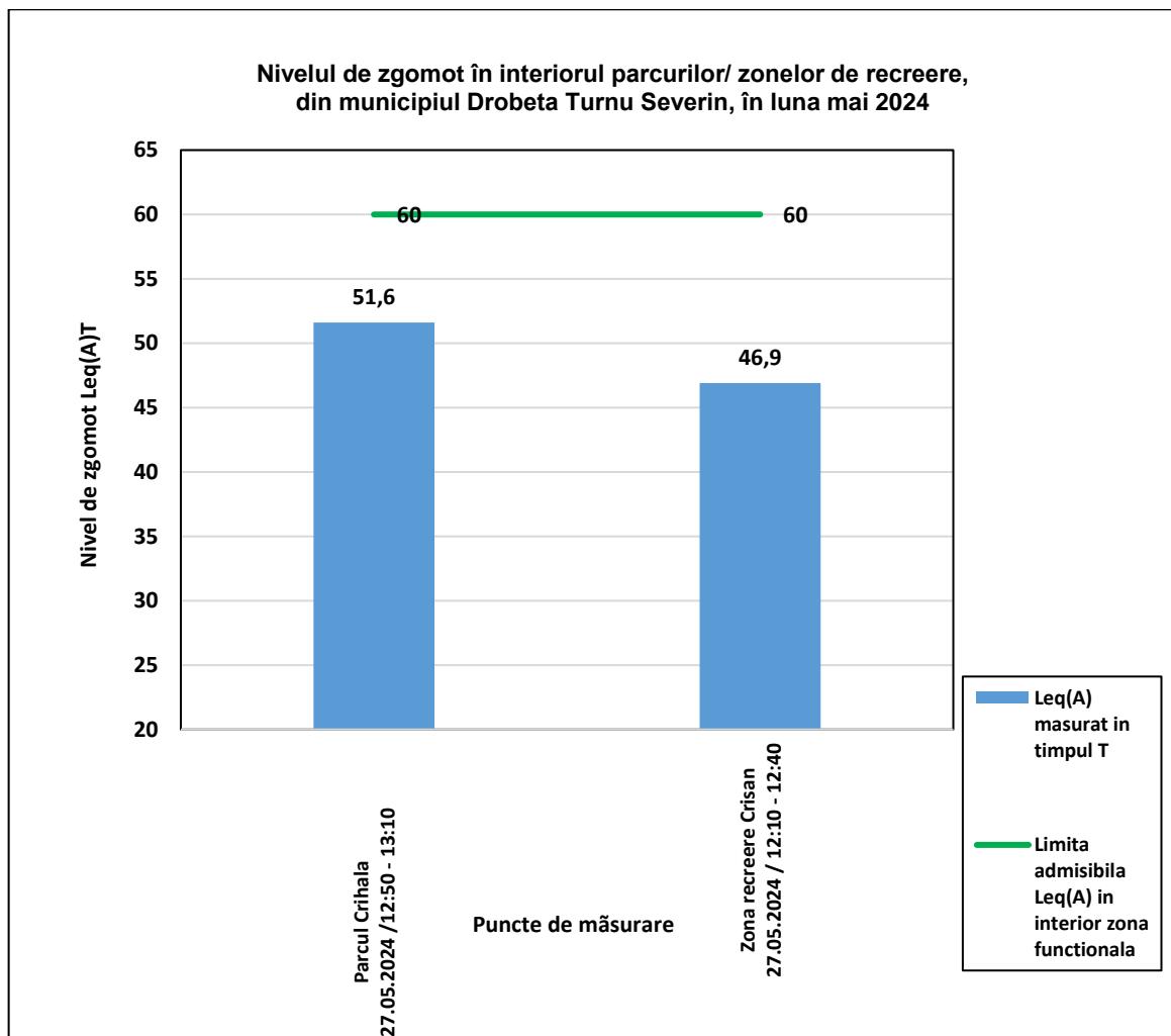
Graficul nr. 21- Nivel de zgomot în interiorul parcurilor / zonelor de recreere, de pe raza municipiului Drobeta Turnu Severin, în luna mai 2024
