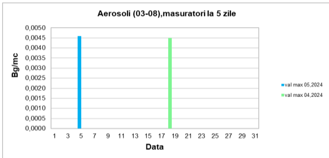
Graficul nr. 10.- Aerosoli atmosferici - activitate specifică beta globală - intervalul 03-08
