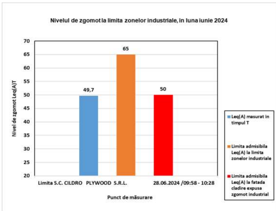
Graficul nr. 20- Nivelul de zgomot la limita zonelor industriale, din municipiul Drobeta Turnu Severin, în luna iunie 2024
