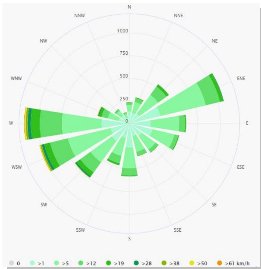
Figura 5– Roza vântului în zona amplasamentului
