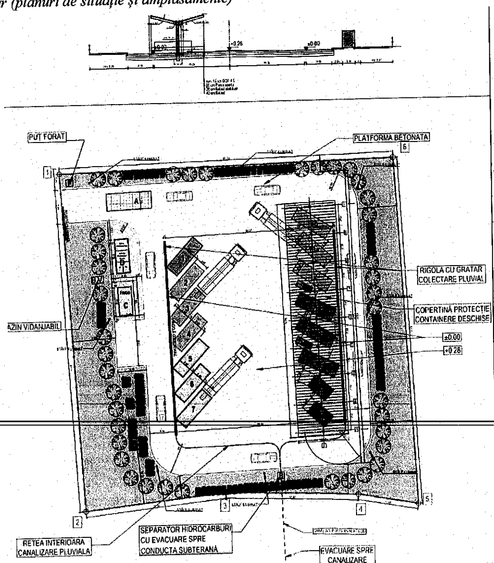
Plan de situație al amplasamentului
