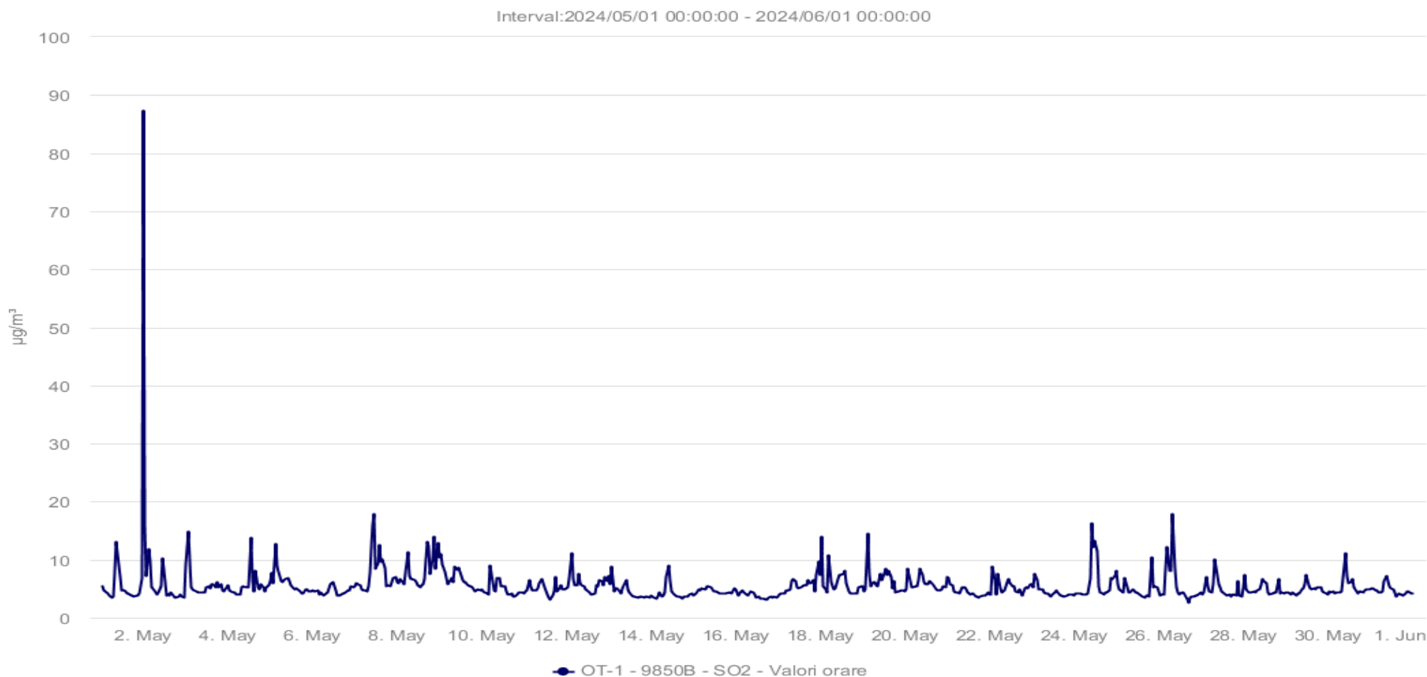
Fig. 1.5. Evoluție valori medii orare SO 2 la stația automata OT1 din județul Olt - luna MAI 2024.
