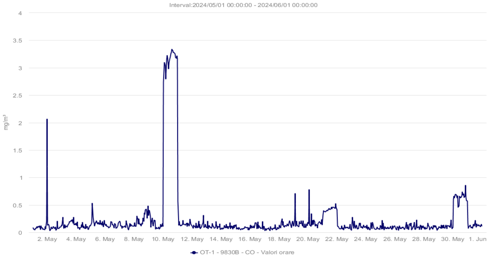
Fig. 1.6 Evoluție valori medii orare pentru CO - luna MAI 2024
