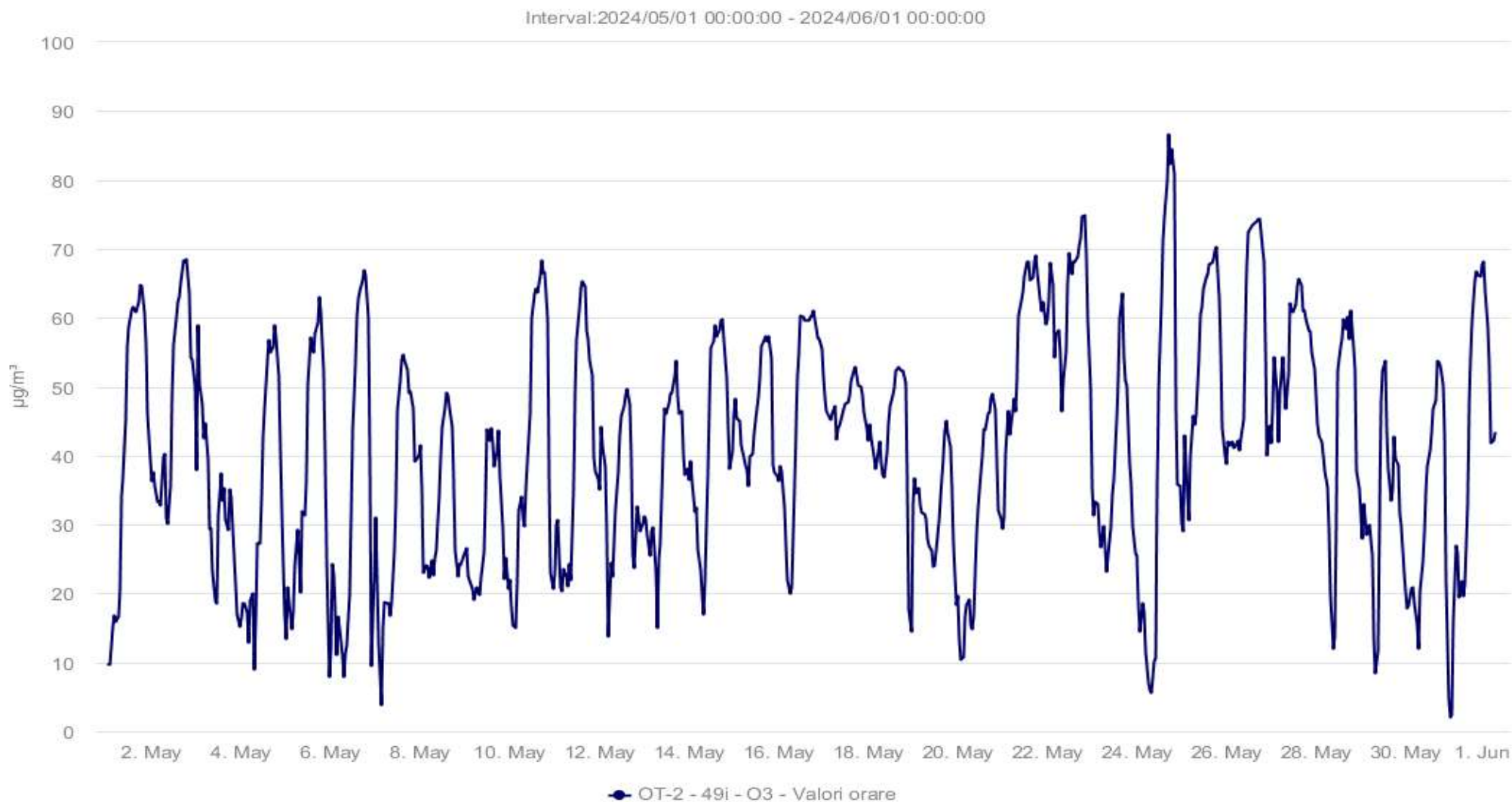
Fig. 1.7. Evoluție valori medii orare pentru O_3 - luna MAI 2024
