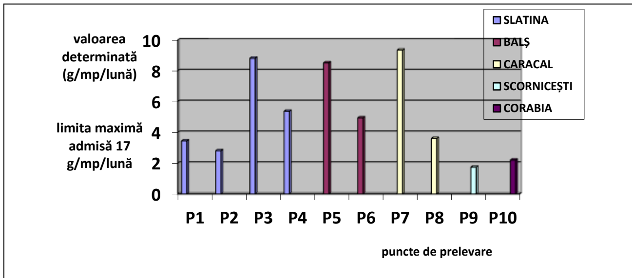
Fig. 1.9. Valori determinate pulberi sedimentabile
