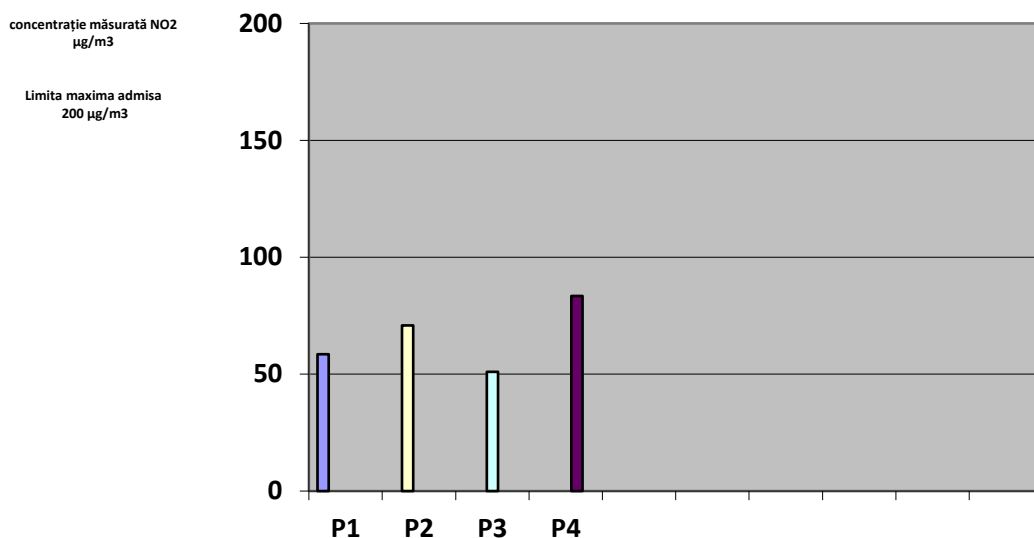
Fig. 1.8. Valori concentrații măsurate NO 2
