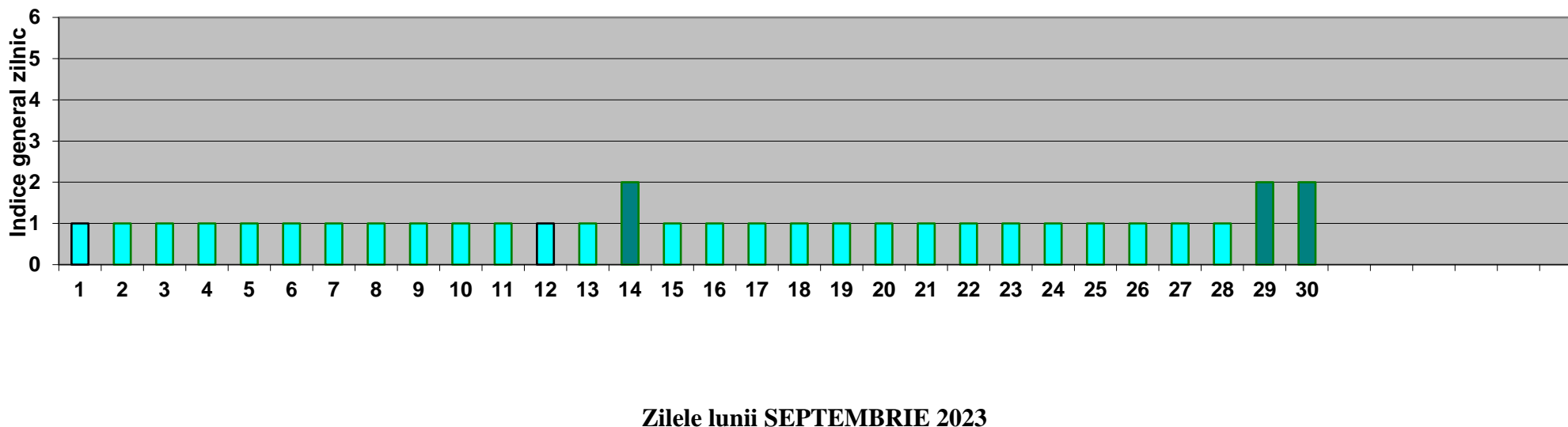
Fig.1.2. Evoluția indicelui general de calitate a aerului în luna SEPTEMBRIE 2023 la stația OT-1 (Slatina, Aleea Grădiște F.N.)
