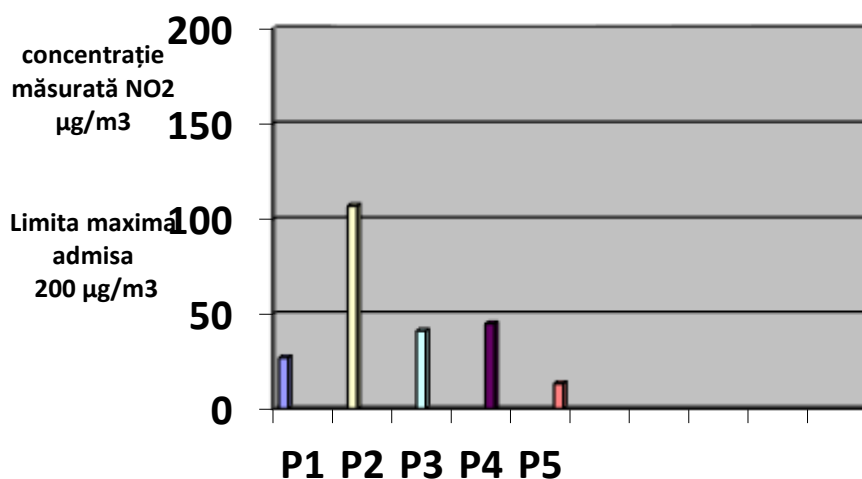
Fig. 1.7. Valori concentrației măsurate NO 2
