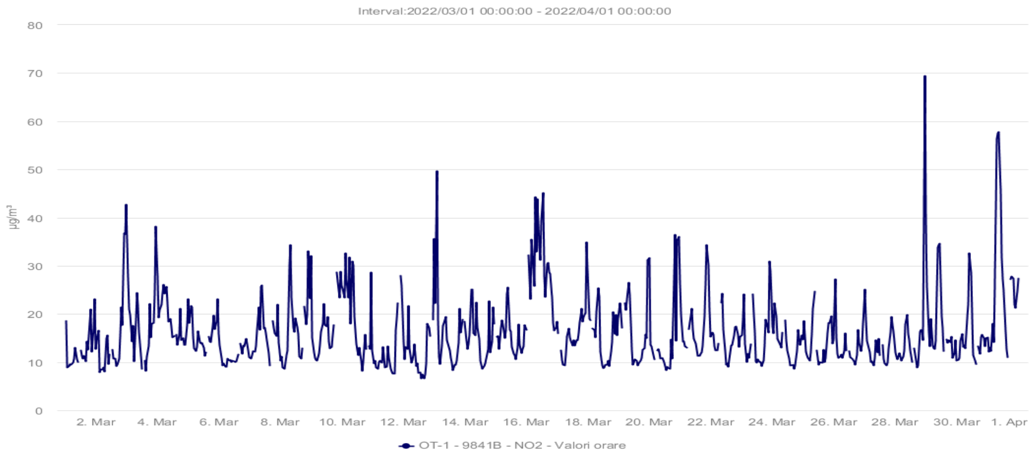
Fig. 1.5 Evoluție valori medii orare NO 2 la stația automată din județul Olt – luna MARTIE 2022
