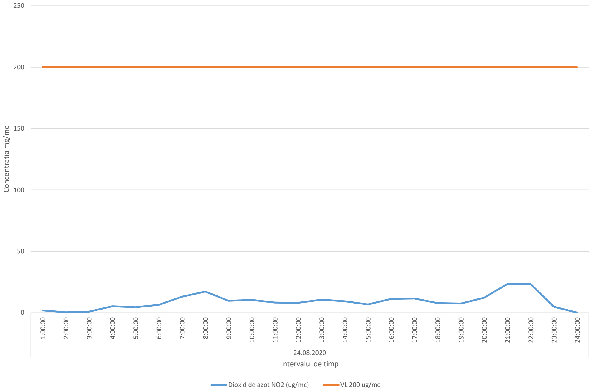
Variatia mediilor orare ale indicatorului NO2 in data de 24.08.2020
