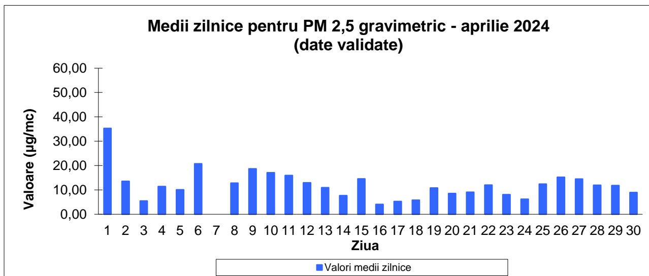
Fig 1.8 Mediile zilnice pentru indicatorul PM2,5
