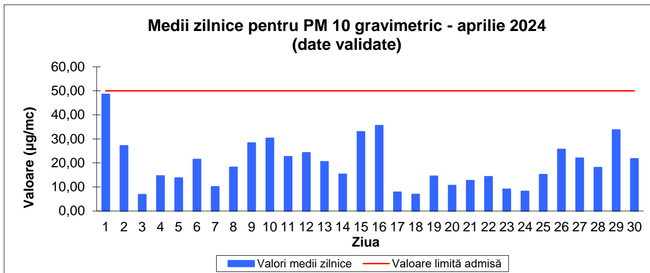
Fig 1.7 Mediile zilnice pentru indicatorul PM10
