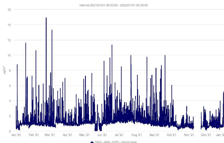
Fig. 5 Evoluția H 2 S în anul 2021 (concentrații medii orare)
