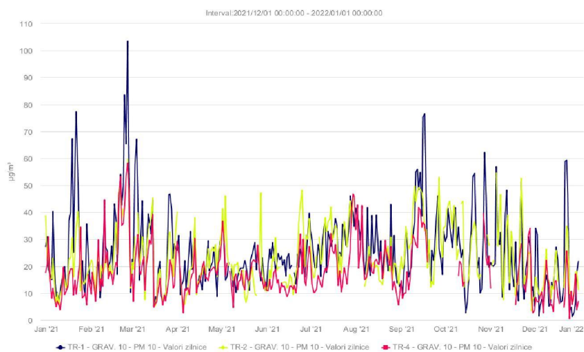
Fig. 8 Evoluția PM 10 în anul 2021 (concentrații medii zilnice)
