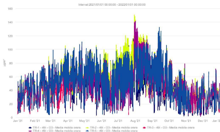
Fig. 4 Evoluția O 3 în anul 2021 (concentrații medii mobile)
