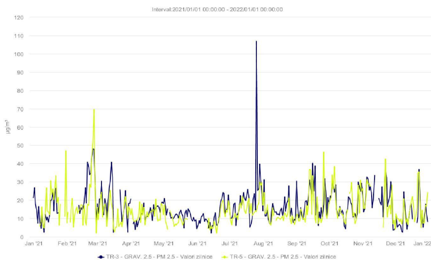
Fig. 9 Evoluția PM 2.5 în anul 2021 (concentrații medii zilnice)
