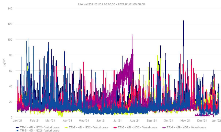
Fig. 2 Evoluția NO 2 în anul 2021 (concentrații medii orare)
