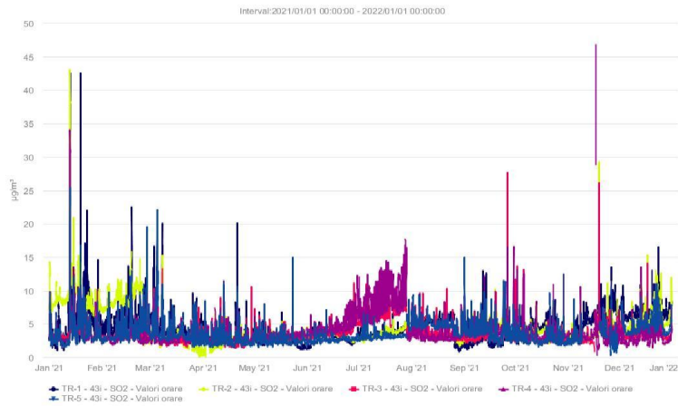
Fig. 1 Evoluția SO 2 în anul 2021 (concentrații medii orare)
