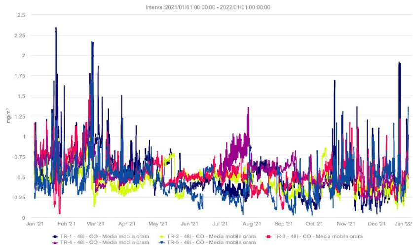
Fig. 3 Evoluția CO în anul 2021 (concentrații medii mobile)
