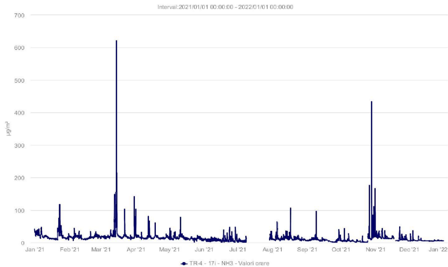
Fig. 7 Evoluția NH 3 în anul 2021 (concentrații medii orare)
