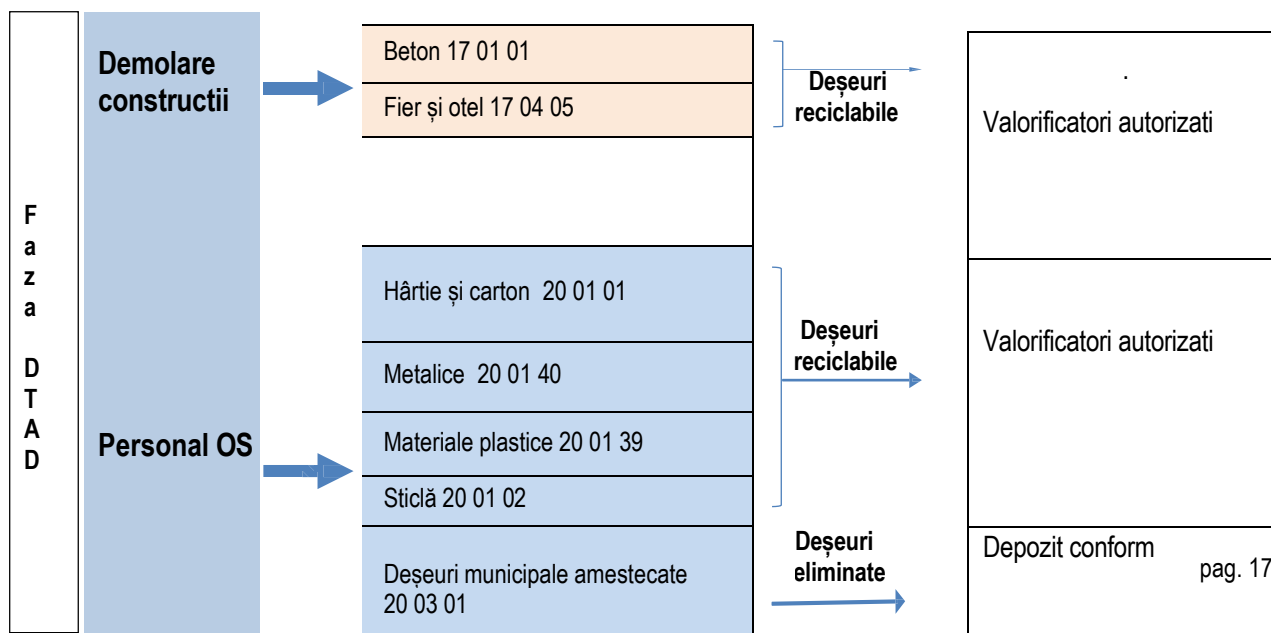
Figura VI-1: Schema flux a deșeurilor pe perioada de execuție a proiectului
