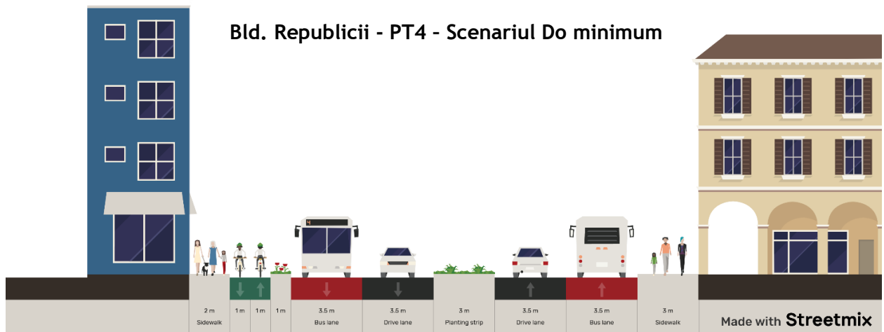
Figura nr. 71 Profil transversal tip 4 - Scenariul Do minimum (pana in 2028) Sectoare limitate de strada de la M. Kogălniceanu pana la Str. M. Eminescu (sursa streetmix.net)
