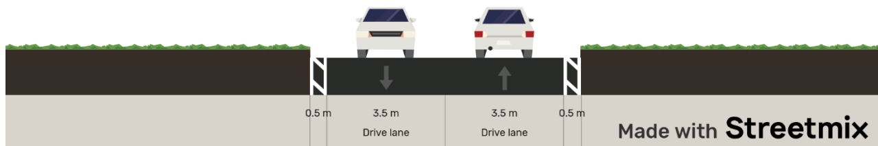
Figura nr. 61 Profil transversal tip 1 - anul de baza (2023) Sector de strada de la Park&Ride Nord pana la I.R.B. (sursa streetmix.net)
