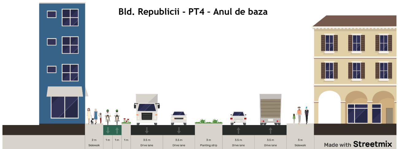
Figura nr. 70 Profil transversal tip 4 - anul de baza (2023) Sectoare limitate de strada de la M. Kogălniceanu pana la Str. M. Eminescu (sursa streetmix.net)
