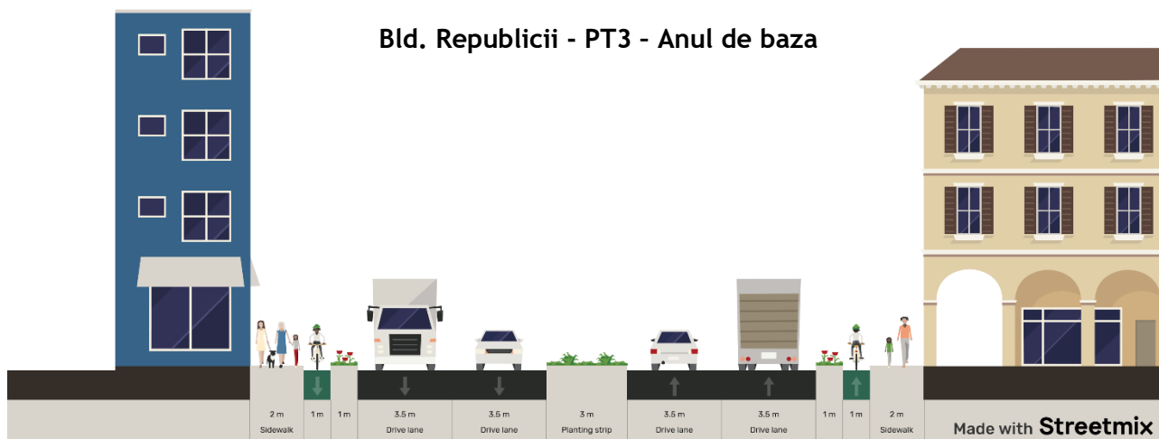
Figura nr. 67 Profil transversal tip 3 - anul de baza (2023) Sector strada de la str. M. Kogălniceanu pana la Str. M. Eminescu (sursa streetmix.net)
