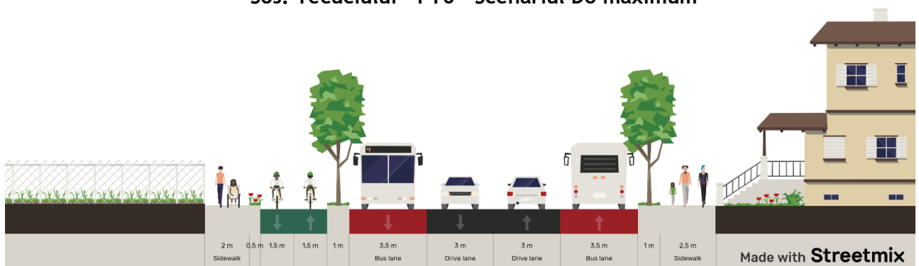
Figura nr. 78 Profil transversal tip 6 - Scenariul Do maximum (pana in 2038) Sector strada de la Park&Ride Sud pana la Autobaza (Petrom) (sursa streetmix.net)
