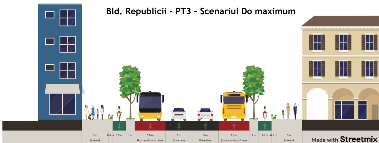
Figura nr. 69 Profil transversal tip 3 - Scenariul Do maximum (până în 2038) Sector strada de la str. M. Kogălniceanu pana la Str. M. Eminescu (sursa streetmix.net)
