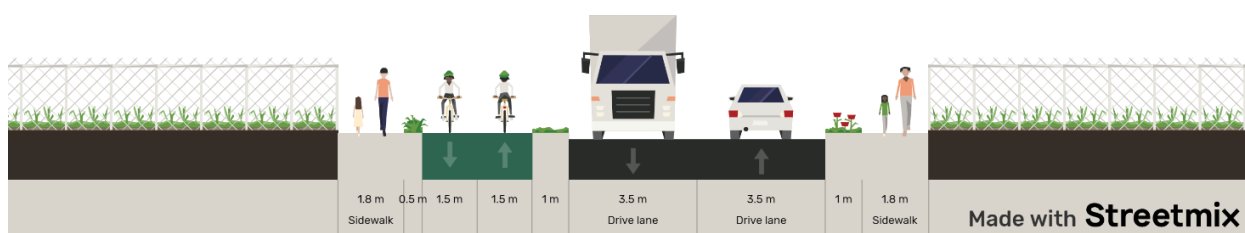
Figura nr. 62 Profil transversal tip 1 - Scenariul Do minimum (pana in 2028) Sector de strada de la Park&Ride Nord pana la I.R.B (sursa streetmix.net)
