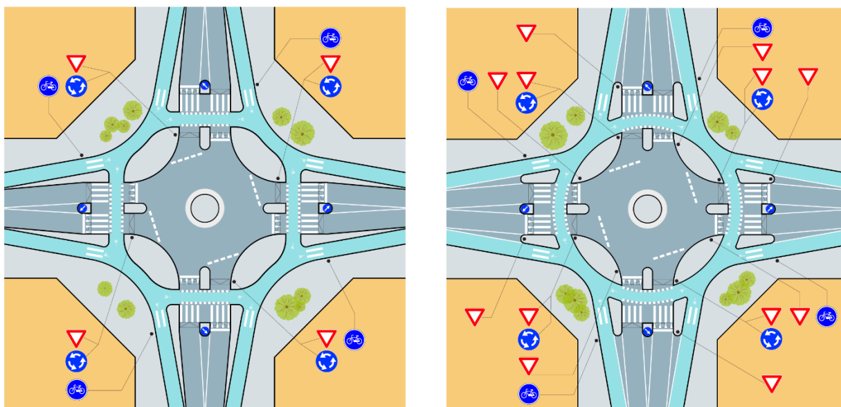
Figura nr. 92 Model amenajare intersecție giratorie conform Ghid metodologic de reglementare a proiectării, execuției, utilizării și mentenanței lucrărilor de infrastructură pentru biciclete, întocmit de OPTAR ( https://optar.ro/ ; https://www.mdlna.ro/pages/proiecteindesfasurare )
