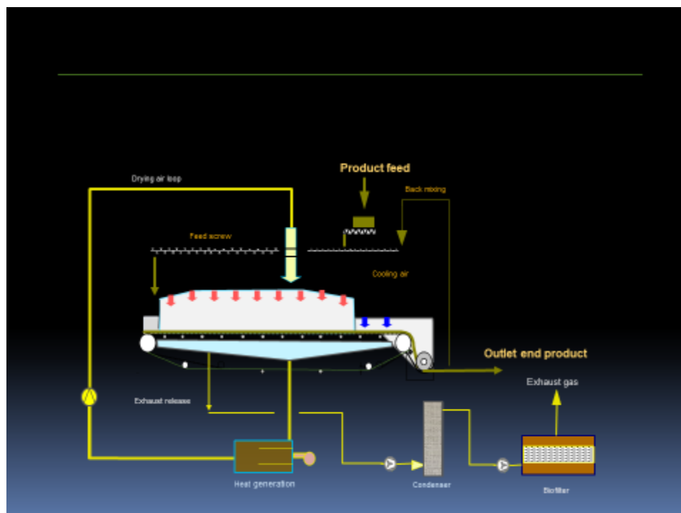
Figura 1: Diagrama de flux a instalației de uscarea
