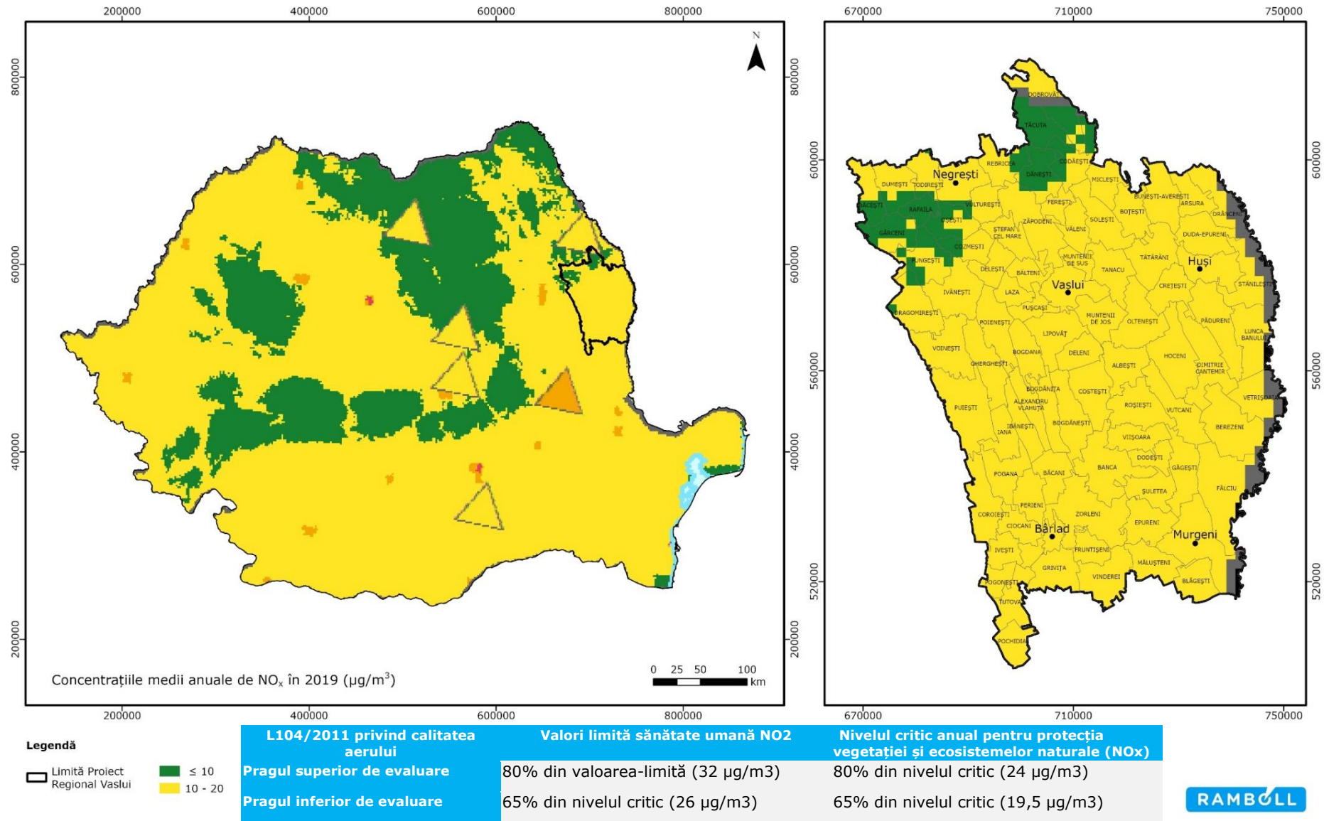
Figura 43: Calitatea aerului în zona de amplasare a proiectului, concentrații medii anuale NO x (2019)
