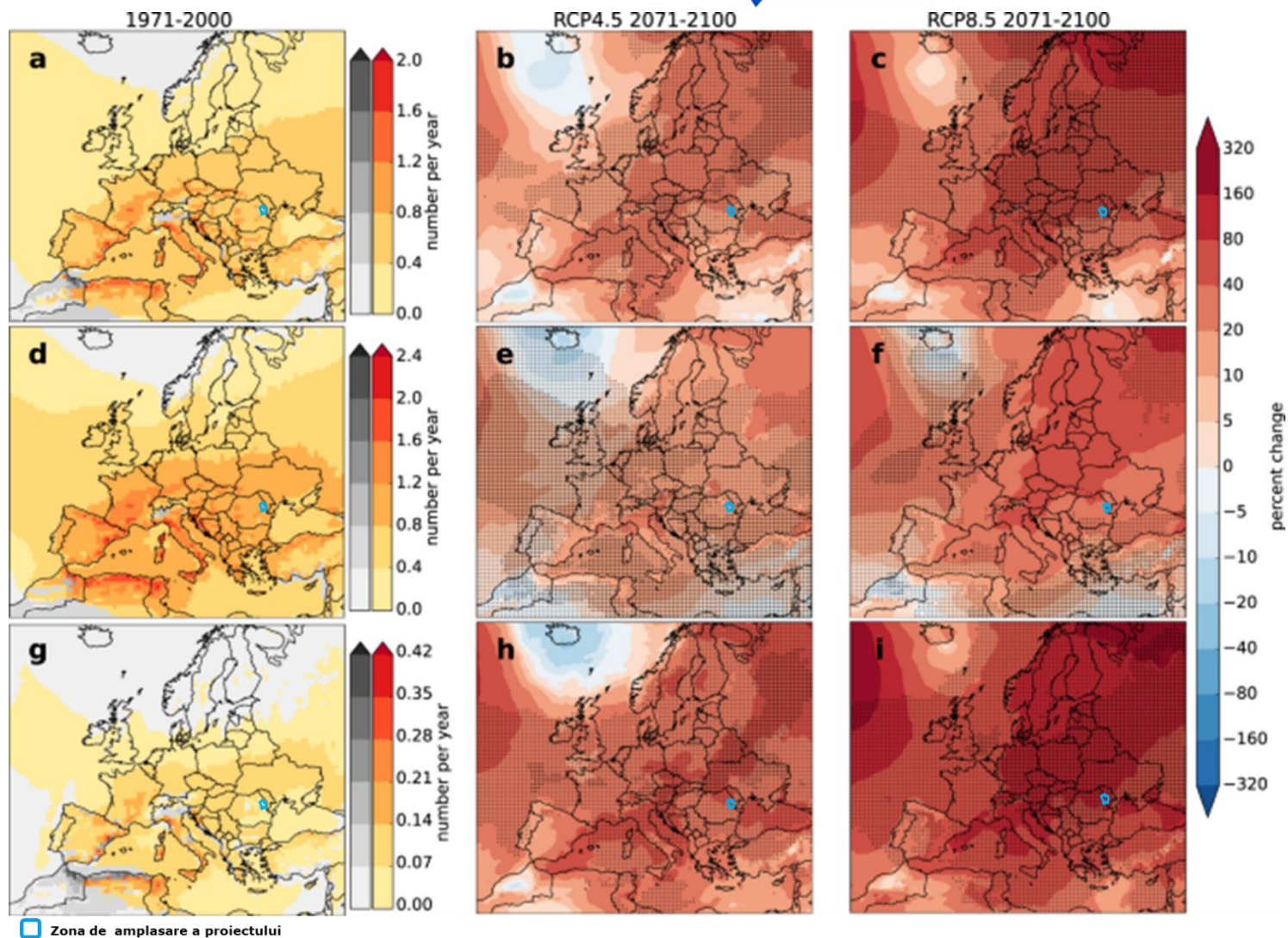
Figură 40: Perioade anuale simulate de 6 ore pentru grindină A-C \geq 2 cm, rafale de vânt D-F \geq 25 m/s și grindină G-I \geq 5 cm într-o perioadă istorică (1971-2000) și procentul de schimbare la sfârșitul secolului (2071-2100) în scenariile b RCP4.5 și c RCP8.5. Tendințele din b, c sunt numite (foarte) robuste atunci când modificarea este mai mare decât (de două ori) abaterea standard inițială a ansamblului de modele. Modificările (foarte) robuste sunt indicate prin puncte negre (mari).
