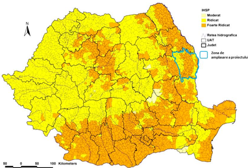
Figura 60: Harta de hazard la seceta pedologică (IHSP) 34
