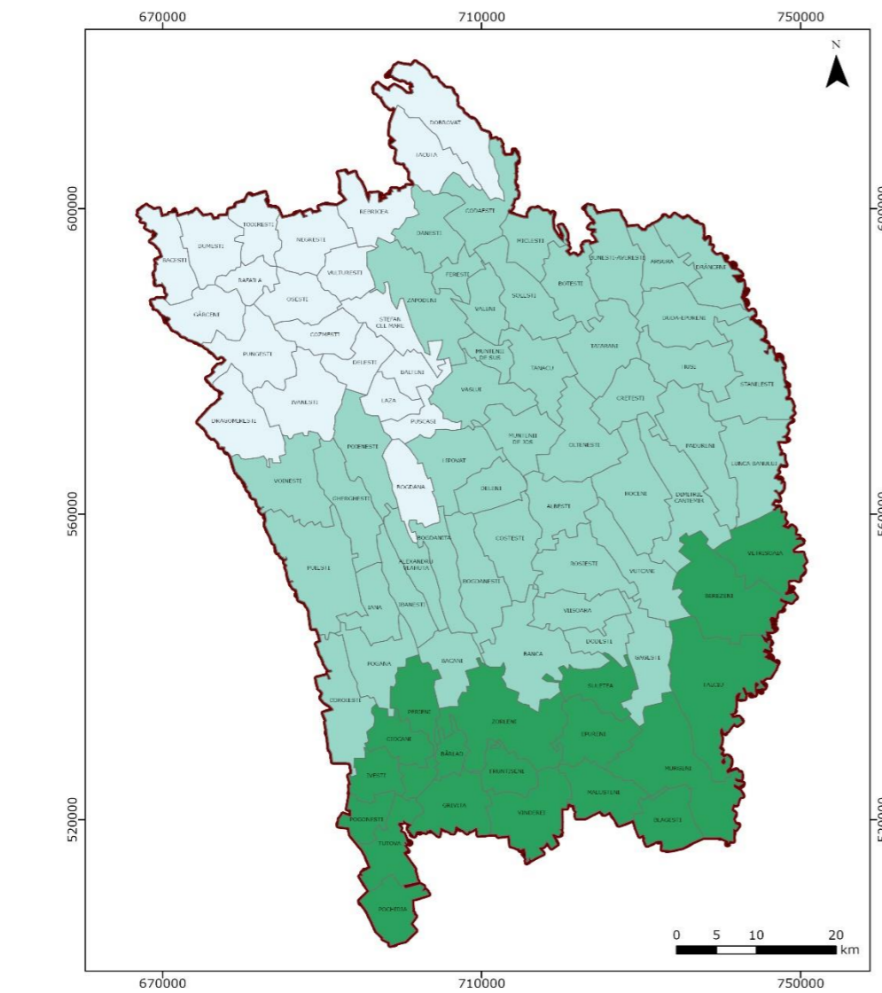
Viteza medie a vântului scenariul RCP4.5 perioada 2041-2070 (m/s)
