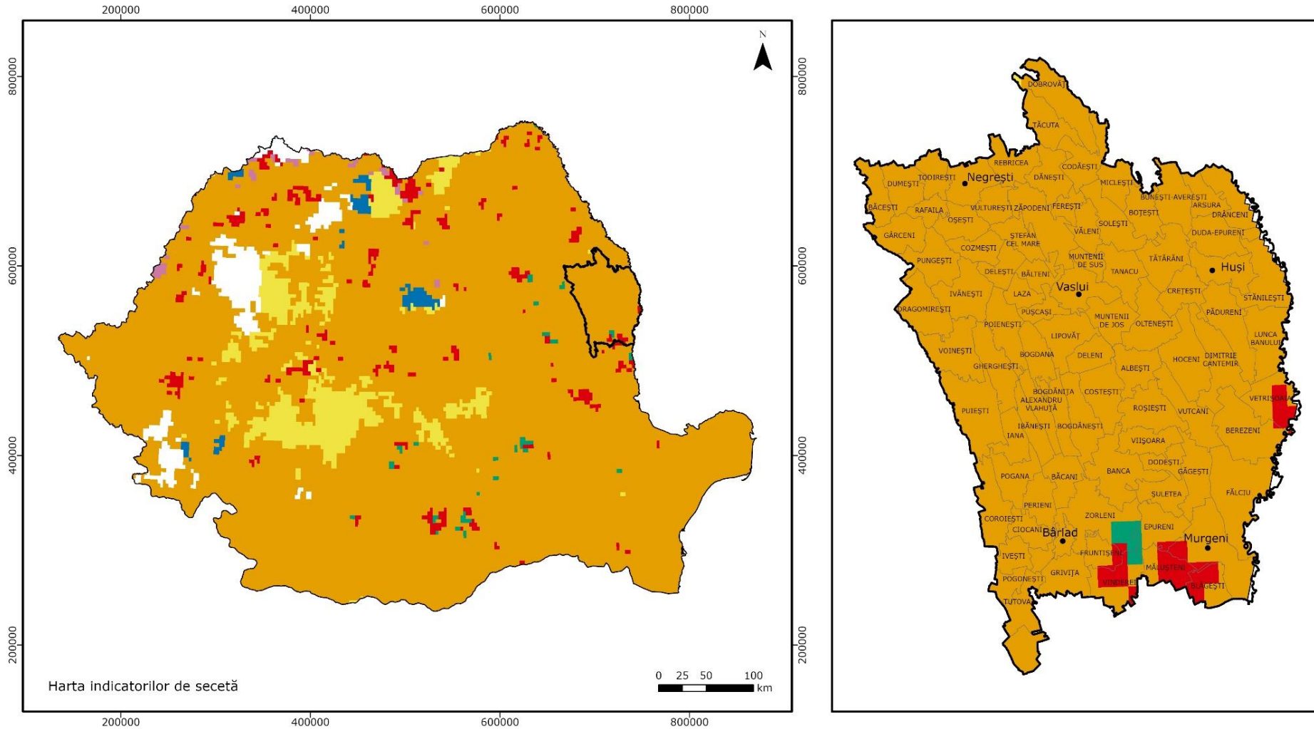
Figura 66: Indicatori de secetă (sursa : EDO, situația indicatorilor de seceta noiembrie 2023)
