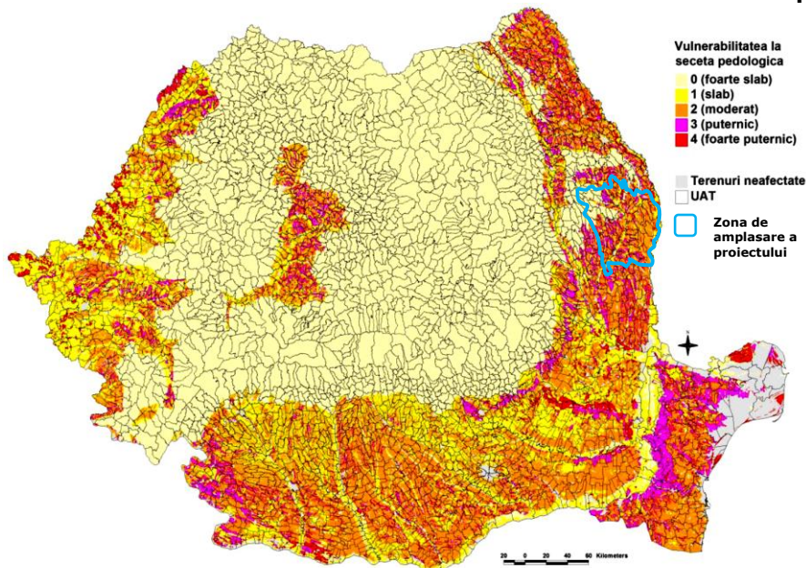
Figura 61: Harta vulnerabilității solurilor la seceta pedologică 35
