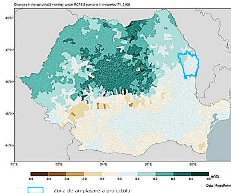
Figura 71: Schimbarea medie a valorii medii a Indicelui Standardizat de Precipitații (SPI), RCP8.5, 2071-2100
