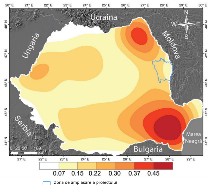
Figura 36b: Distribuția spațială a tornadelor în România raportate între 1990–2013 (tornade per 105 km 2 / an) Sursa: Buletinul Societății Meteorologie Române, anul III, nr.1, martie 2015, Antonescu și Bell (2015),
