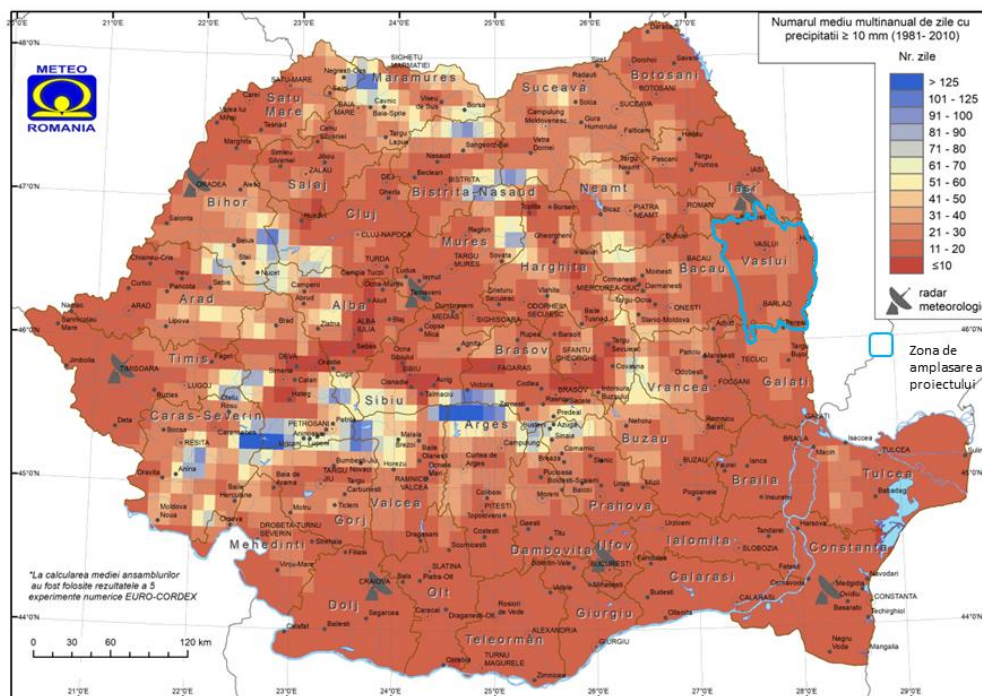
Figura 48: Distribuția spațială a frecvenței medii multianuale a zilelor cu precipitații abundente (mai mari sau egale cu 10 mm) în România (1981-2010)
