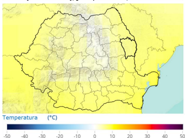
Figură 26: Temperatura minimă medie sezonieră (1991-2020) 19
