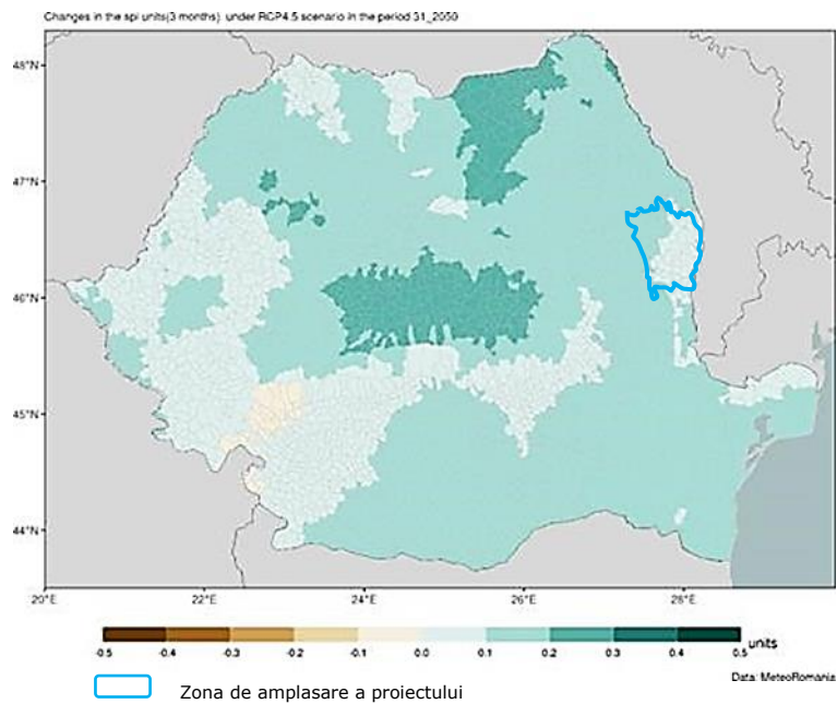
Figura 72: Schimbarea medie a valorii medii a Indicelui Standardizat de Precipitații (SPI), RCP4.5, 2031-2050
