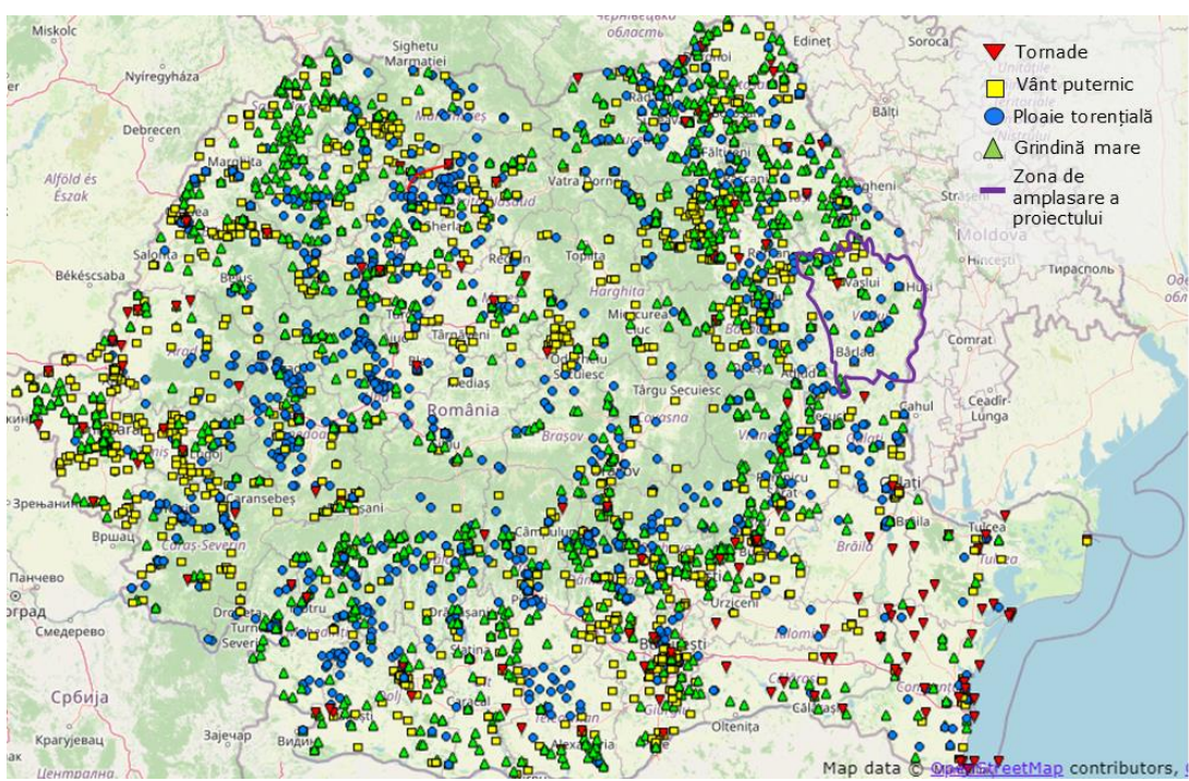
Figura 37a: Situația furtunilor convective severe raportate în România (1980-martie 2024) Sursa: European Severe Weather Database, 2024
