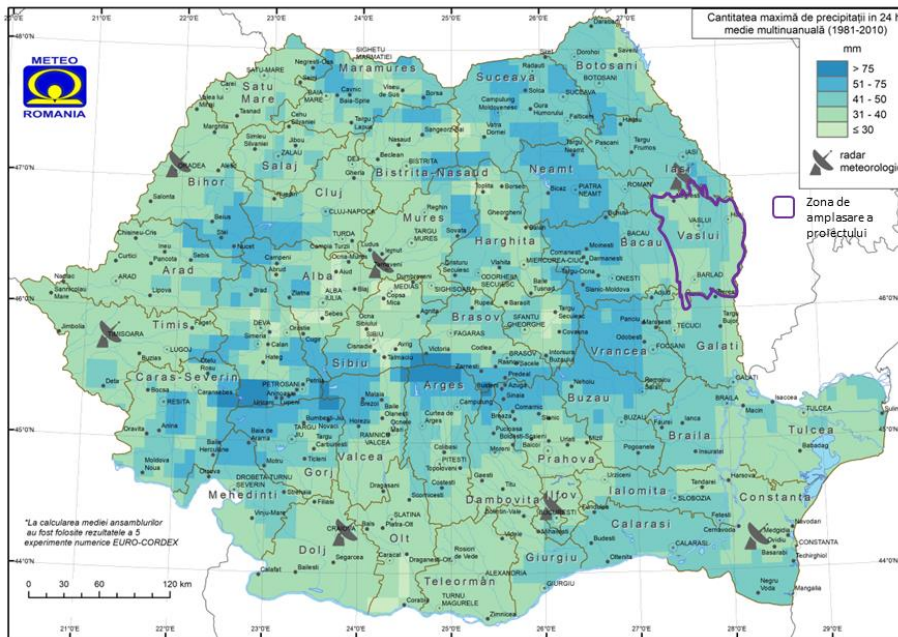
Figura 49: Distribuția teritorială a cantităților maxime de precipitații în 24 de ore medii multianuale în România (1981-2010) sursa: Agenția Național Meteorologică, proiect Ramboll
