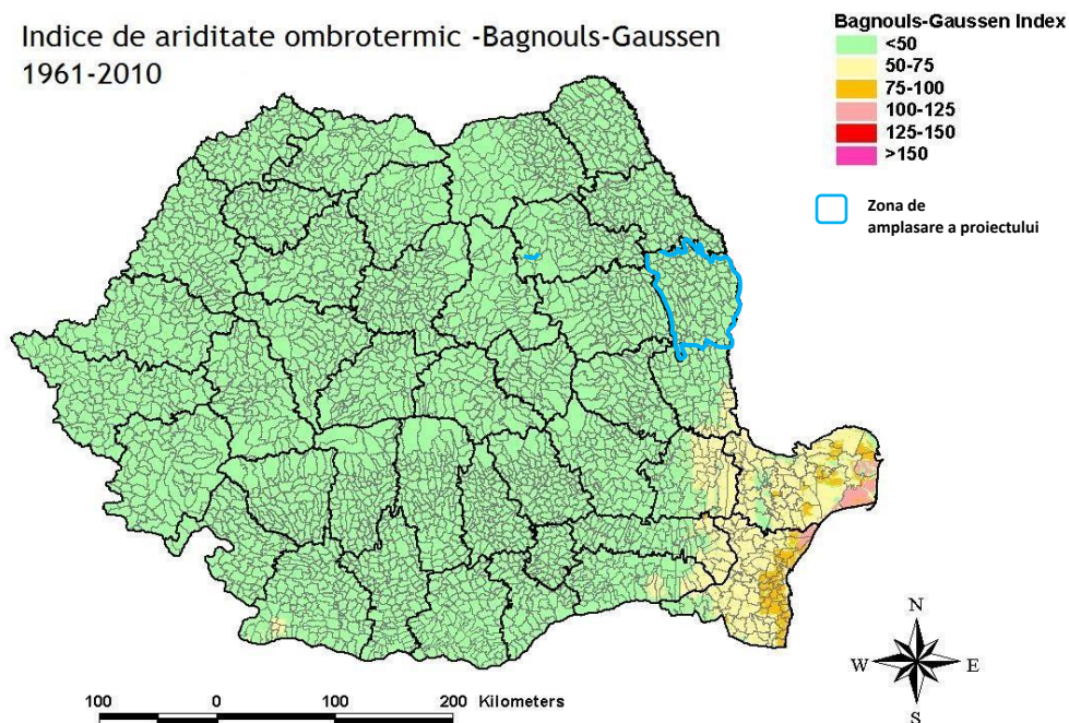
Figura 65: Evaluării zonelor sensibile la deșertificare (1961-2010)
