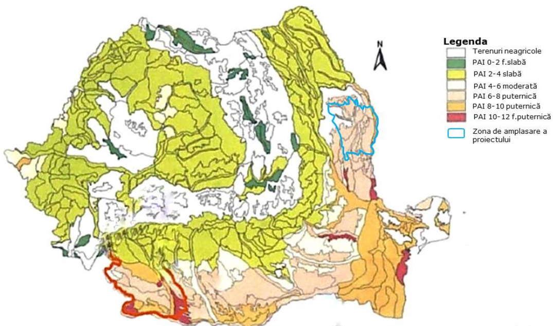
Figura 62: Zone cu risc diferit la seceta, caracterizate prin indici PAI, funcție de sol, relief și apele subterane (sursa: INHGA)
