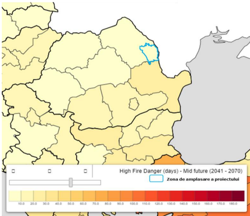
Figura 80: Zile cu risc mare de incendiu în România, Regiunea Nord-Est, zona de amplasare a proiectului, RCP 4.5 (2041-2070) Sursa: Copernicus Climate Change Service (C3S)
