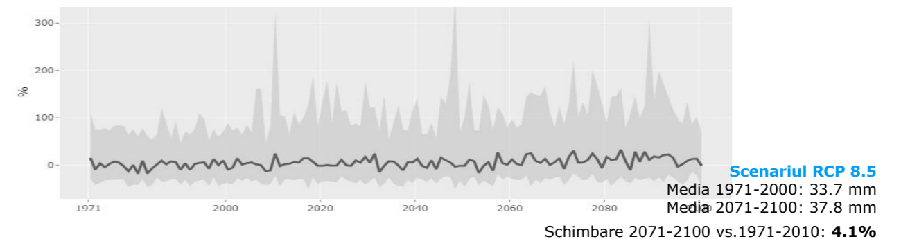
Figura 53: Cantități precipitații maxime 24h - scenariul RCP8.5 (2071-2100)
