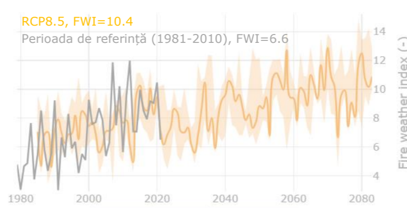
Figura 77: Indicele Meteo de Incendiu (FWI) în România, Regiunea Nord-Est, zona de amplasare a proiectului, RCP 8.5 (2071-2083)
