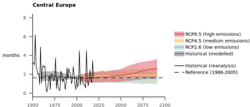
Figura 70: Modificarea preconizată a duratei secetelor meteorologice pentru Europa Centrală 41
