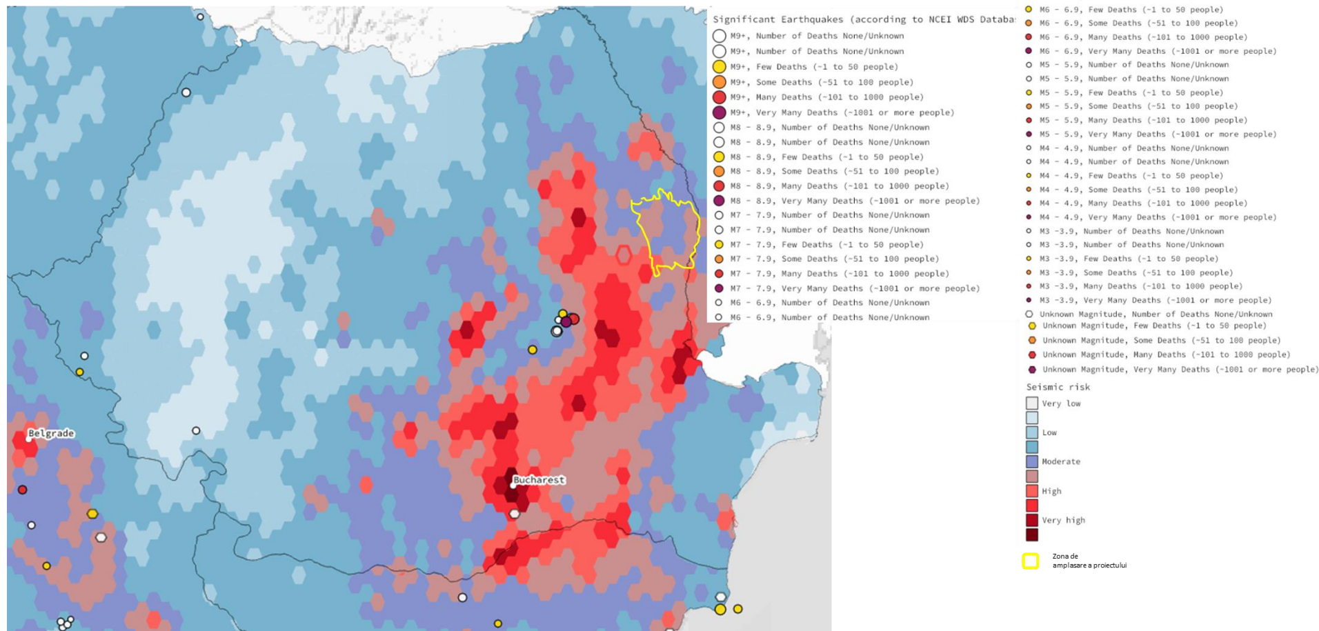
Figura 87: Harta de indicelui european de risc seismic
