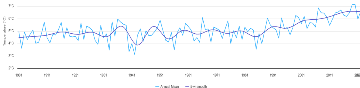
Figură 27: Evoluția temperaturii minime anuale județul Vaslui (1991-2020) 20
