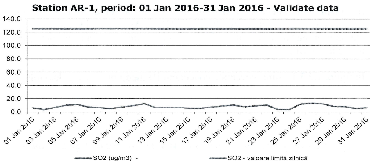
Fig. 1.2.1.2. Concentrațiile medii zilnice ale poluantului SO 2
