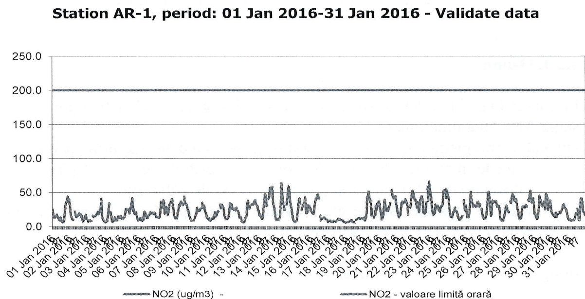
Fig.1.2.2.1. Concentrațiile medii orare ale poluantului NO 2
