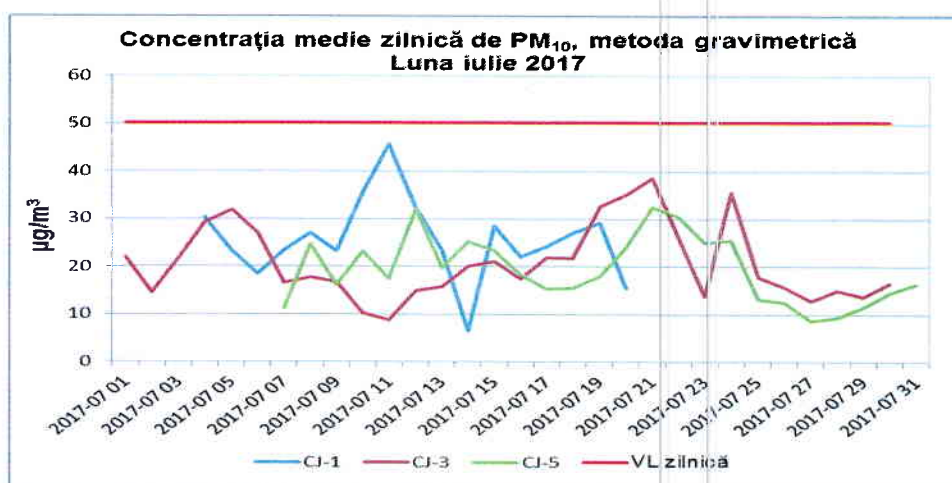
Figura 1.2.5.1. Evoluția mediilor zilnice de PM 10 , în luna iulie 2017
