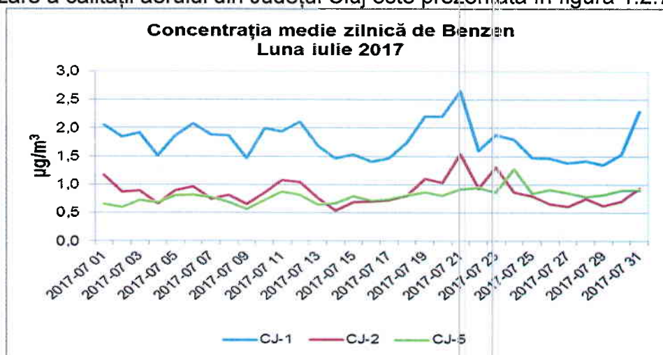
Figura 1.2.7.1. Evoluția mediilor zilnice de benzen, în luna iulie 2017
