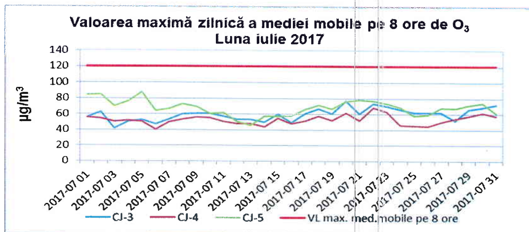
Figura 1.2.3.1. Evoluția maximelor zilnice ale mediilor mobile pe 8 ore de \text{O}_3 , în luna iulie 2017
