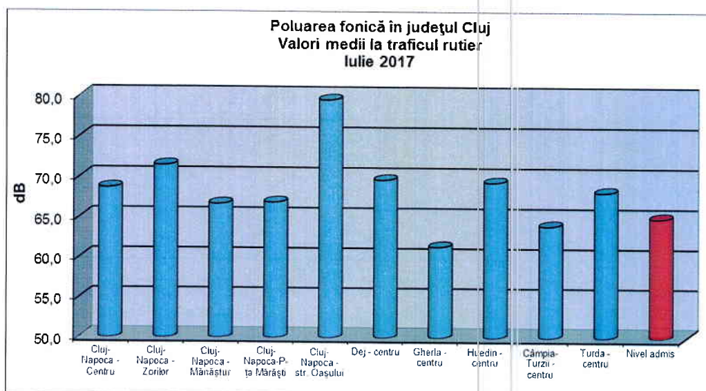
Figura 4.1. Rezultatele monitorizării nivelului de zgomot
