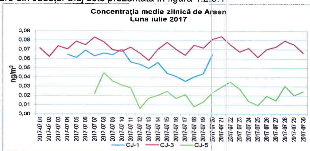
Figura 1.2.6.1. Evoluția mediilor zilnice de As, în luna iulie 2017
