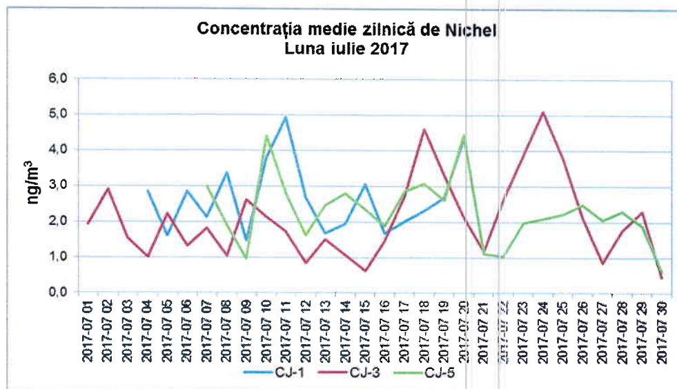
Figura 1.2.6.3. Evoluția mediilor zilnice de Ni, în luna iulie 2017
