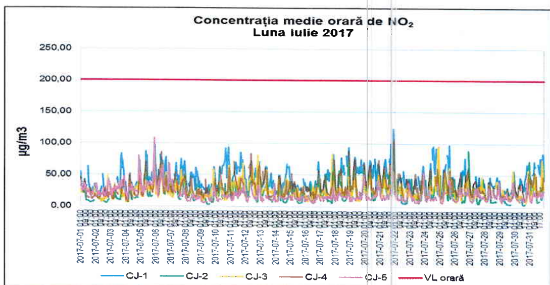
Figura 1.2.2.1. Evoluția mediilor orare de NO 2 în luna iulie 2017
