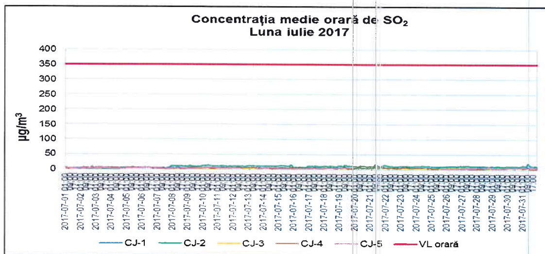
Figura 1.2.1.1. Evoluția mediilor orare de SO 2 în luna iulie 2017
