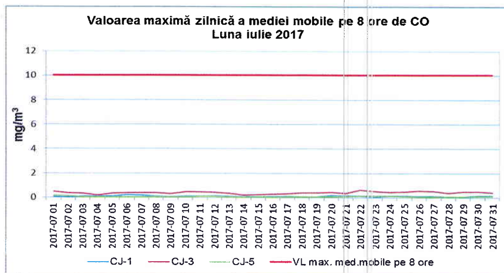
Figura 1.2.4.1. Evoluția maximelor zilnice ale mediilor mobile pe 8 ore de CO, în luna iulie 2017
