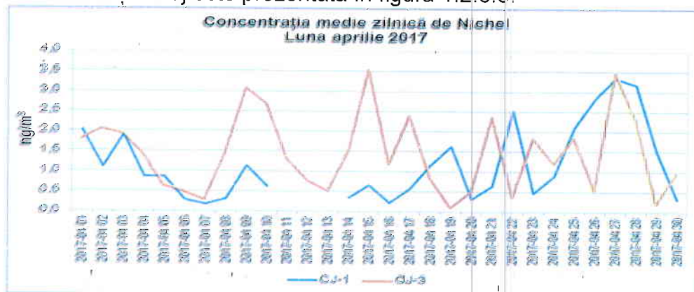
Figura 1.2.6.3. Evoluția mediilor zilnice de Ni, în luna aprilie 2017
