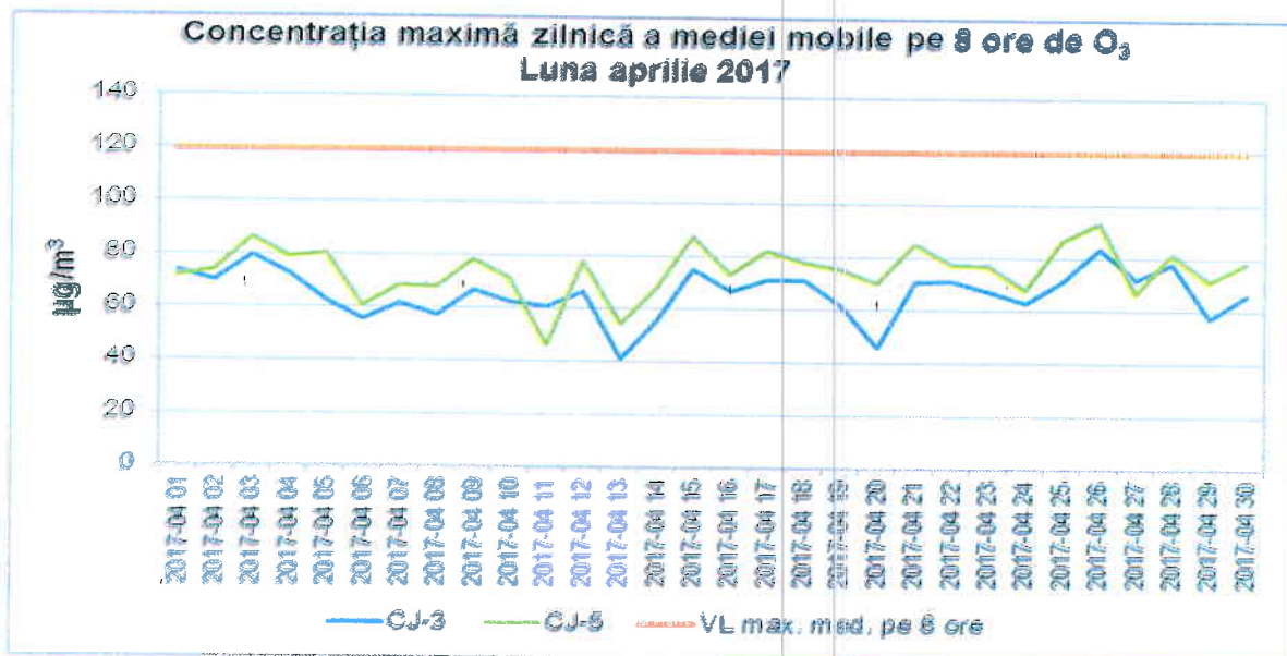
Figura 1.2.3.1. Evoluția maximelor zilnice ale mediilor mobile pe 8 ore de \text{O}_3 , în luna aprilie 2017
