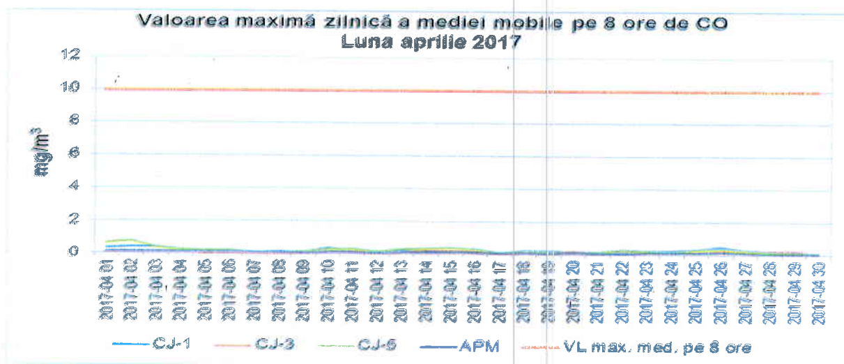
Figura 1.2.4.1. Evoluția maximelor zilnice ale mediilor mobile pe 8 ore de CO, în luna aprilie 2017
