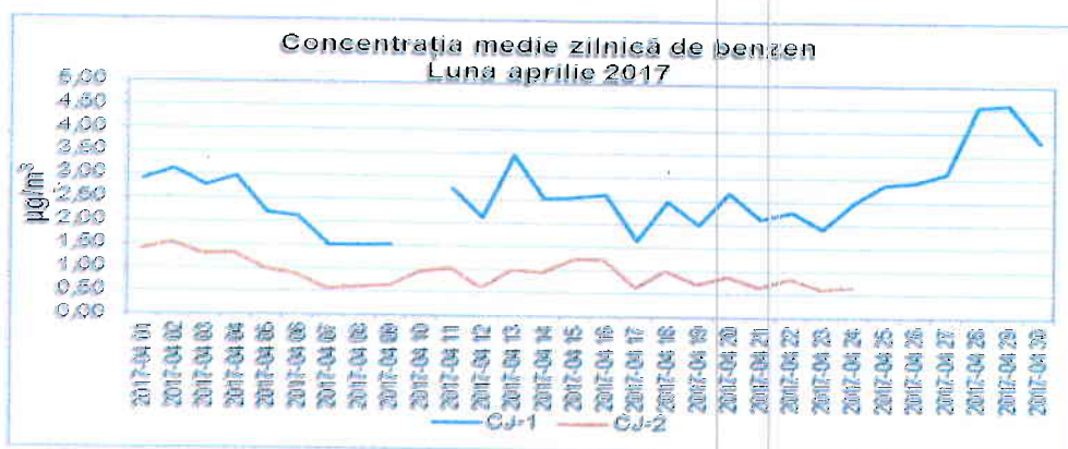
Figura 1.2.7.1. Evoluția mediilor zilnice de benzen, în luna aprilie 2017
