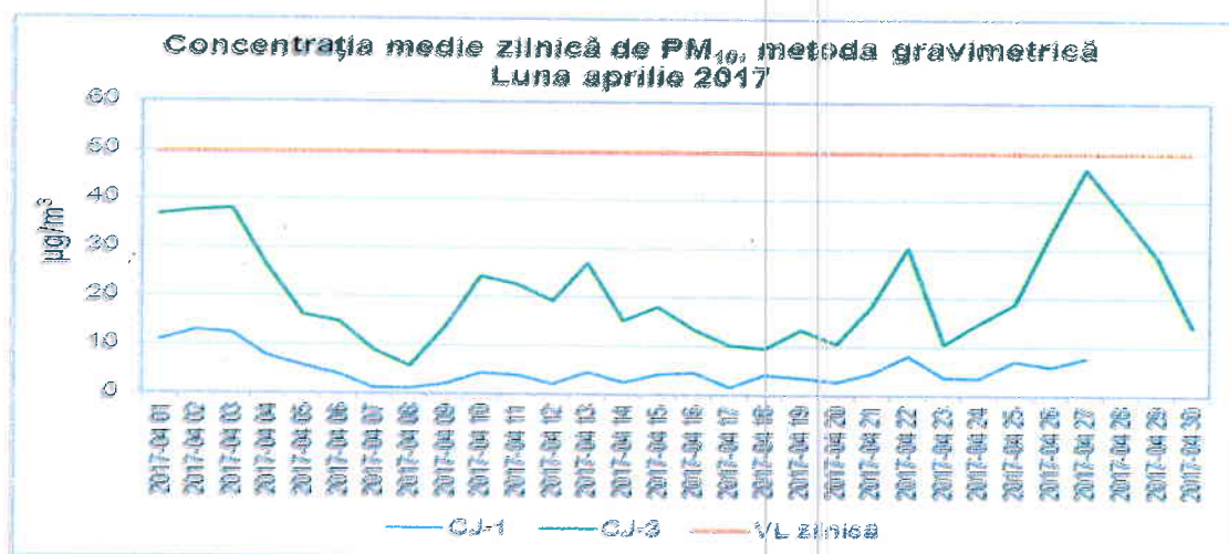
Figura 1.2.5.1. Evoluția mediilor zilnice de PM 10 , în luna aprilie 2017
