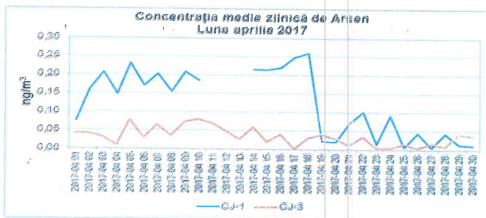
Figura 1.2.6.1. Evoluția mediilor zilnice de As, în luna aprilie 2017
