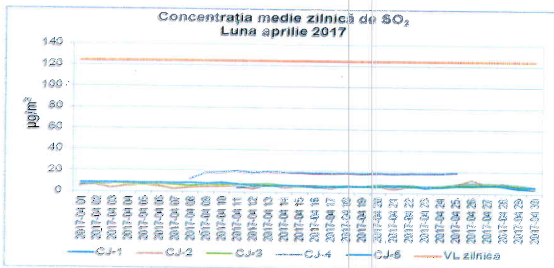
Figura 1.2.1.1. Evoluția mediilor orare de SO 2 în luna aprilie 2017
