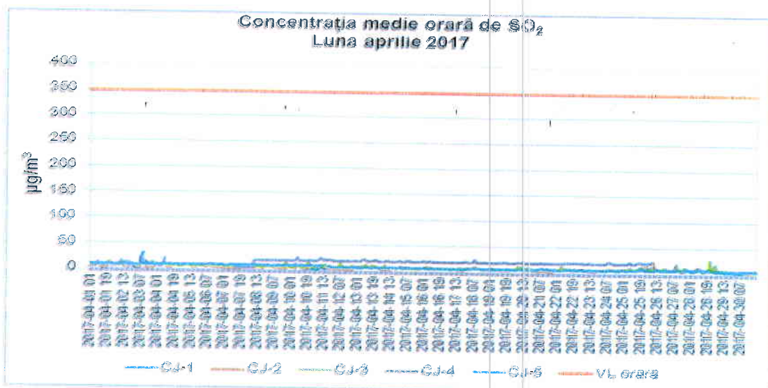
Figura 1.2.1.1. Evoluția mediilor zilnice de SO 2 în luna aprilie 2017
