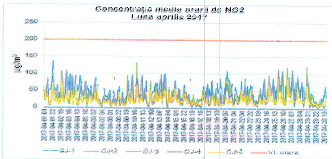
Figura 1.2.2.1. Evoluția mediilor orare de NO 2 în luna aprilie 2017
