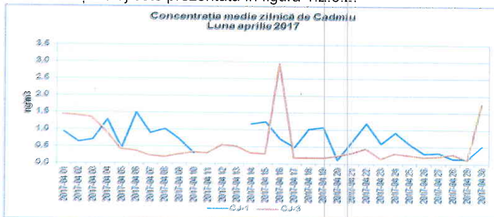
Figura 1.2.6.2. Evoluția mediilor zilnice de Cd, în luna aprilie 2017
