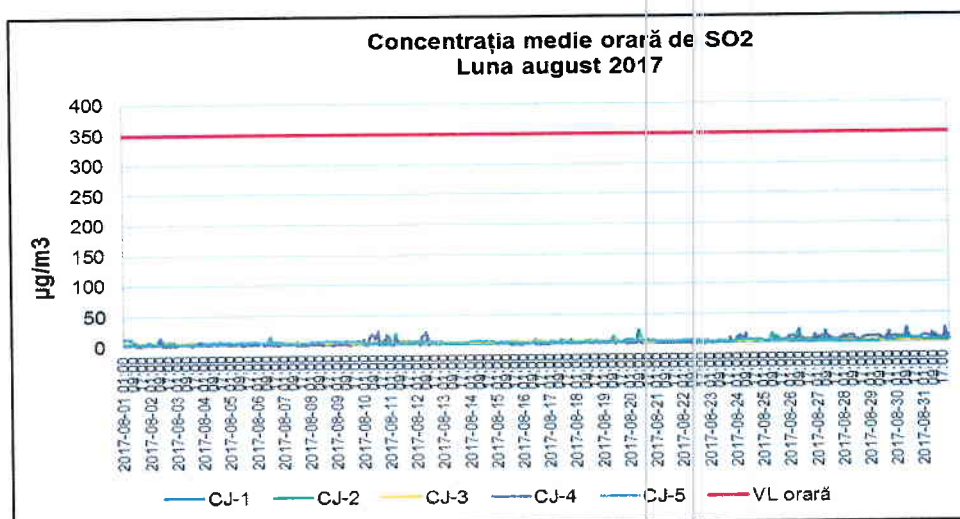
Figura 1.2.1.1. Evoluția mediilor orare de SO 2 în luna august 2017
