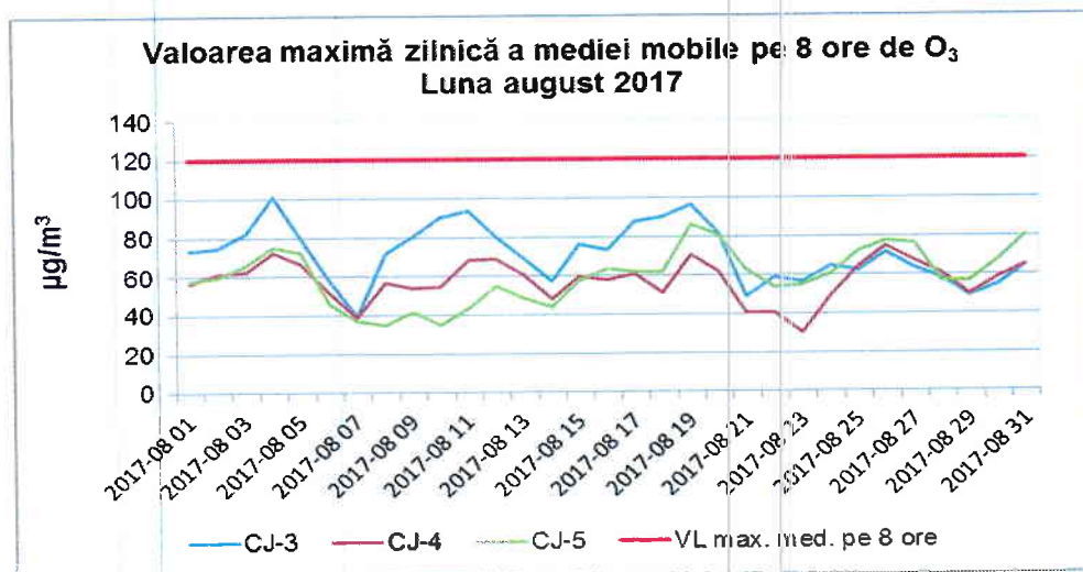
Figura 1.2.3.1. Evoluția maximelor zilnice ale mediilor mobile pe 8 ore de \text{O}_3 , în luna august 2017
