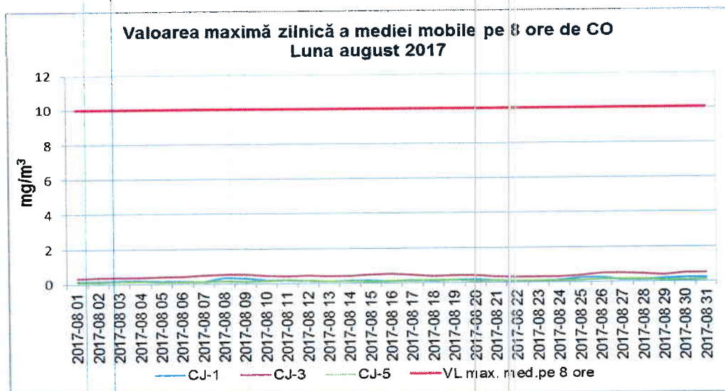
Figura 1.2.4.1. Evoluția maximelor zilnice ale mediilor mobile pe 8 ore de CO, în luna august 2017
