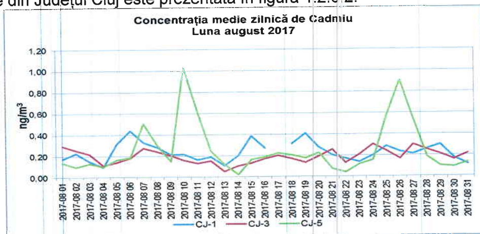
Figura 1.2.6.2. Evoluția mediilor zilnice de Cd, în luna august 2017
