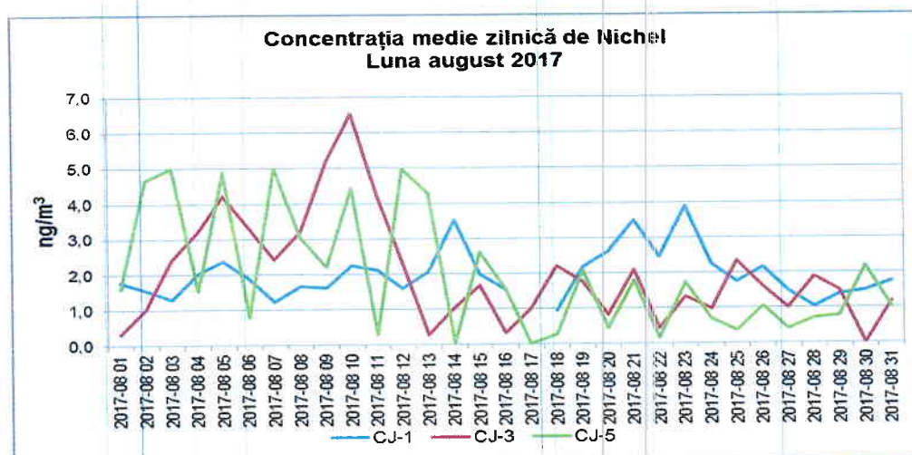
Figura 1.2.6.3. Evoluția mediilor zilnice de Ni, în luna august 2017
