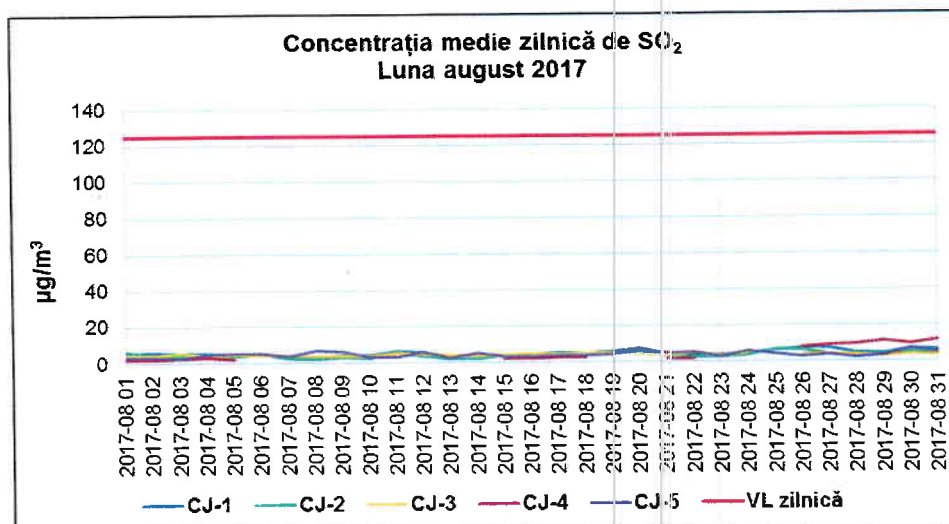
Figura 1.2.1.1. Evoluția mediilor zilnice de SO 2 în luna august 2017
