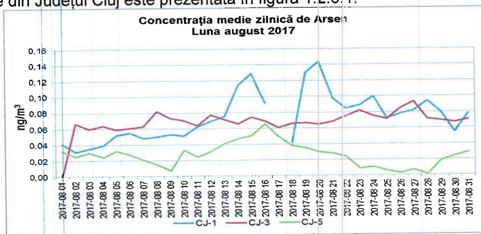
Figura 1.2.6.1. Evoluția mediilor zilnice de As, în luna august 2017
