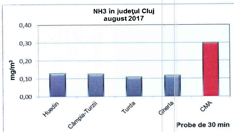
Figura 1.1.1. Rezultatele monitorizării amoniacului
