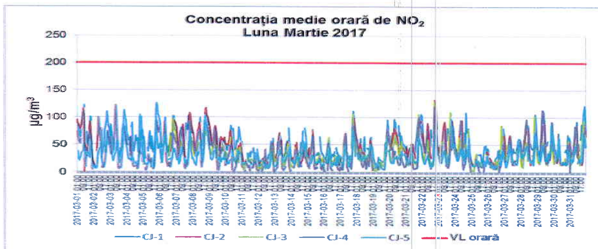
Figura 1.2.2.1. Evoluția mediilor orare de NO 2 în luna martie 2017
