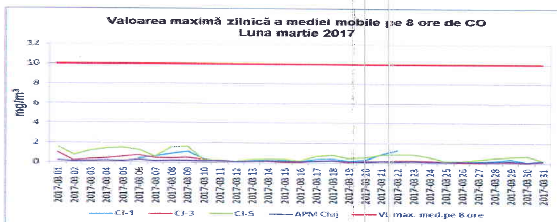
Figura 1.2.4.1. Evoluția maximelor zilnice ale mediilor mobile pe 8 ore de CO, în luna martie 2017
