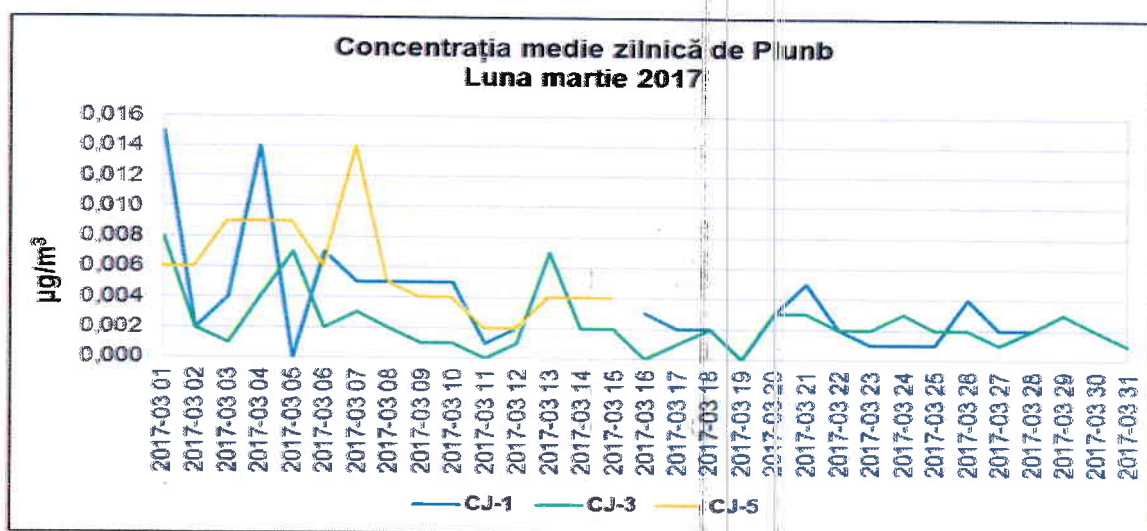
Figura 1.2.6.4. Evoluția mediilor zilnice de Pb, în luna martie 2017
