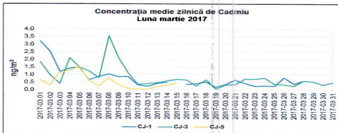
Figura 1.2.6.2. Evoluția mediilor zilnice de Cd, în luna martie 2017
