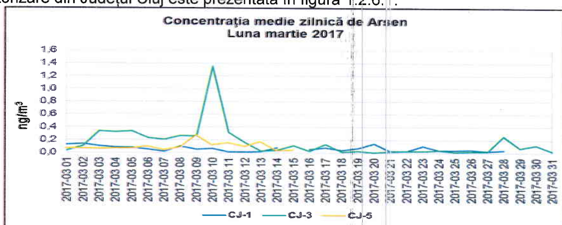
Figura 1.2.6.1. Evoluția mediilor zilnice de As, în luna martie 2017
