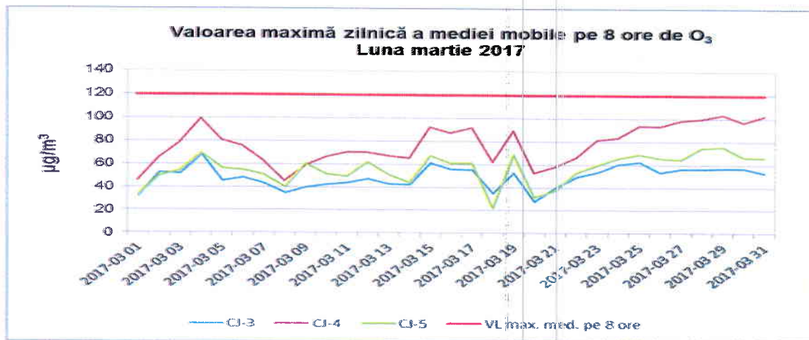
Figura 1.2.3.1. Evoluția maximelor zilnice ale mediilor mobile pe 8 ore de \text{O}_3 , în luna martie 2017
