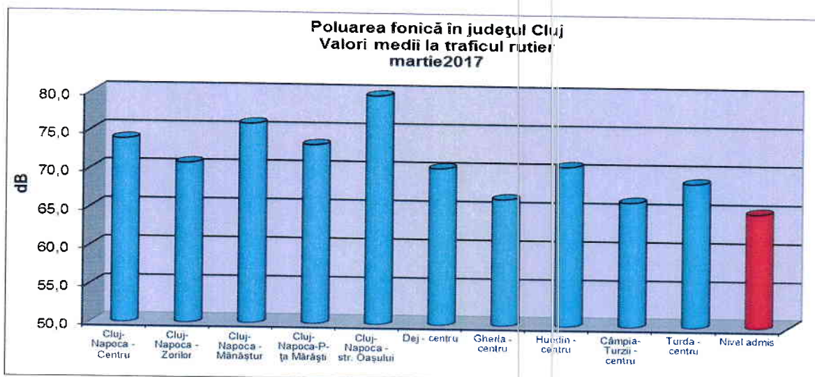
Figura 4.1. Rezultatele monitorizării nivelului de zgomot
