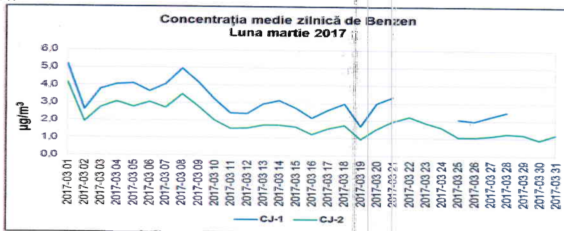
Figura 1.2.7.1. Evoluția mediilor zilnice de benzen, în luna martie 2017
