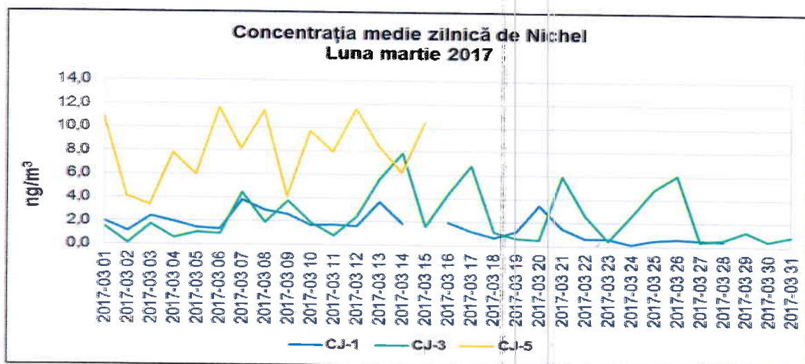
Figura 1.2.6.3. Evoluția mediilor zilnice de Ni, în luna martie 2017
