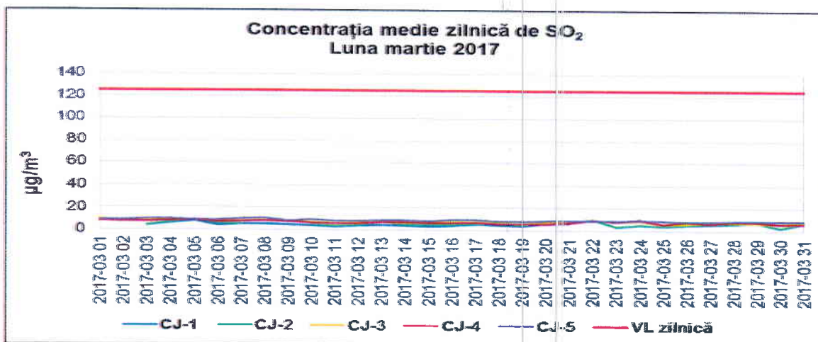
Figura 1.2.1.1. Evoluția mediilor zilnice de SO 2 în luna martie 2017
