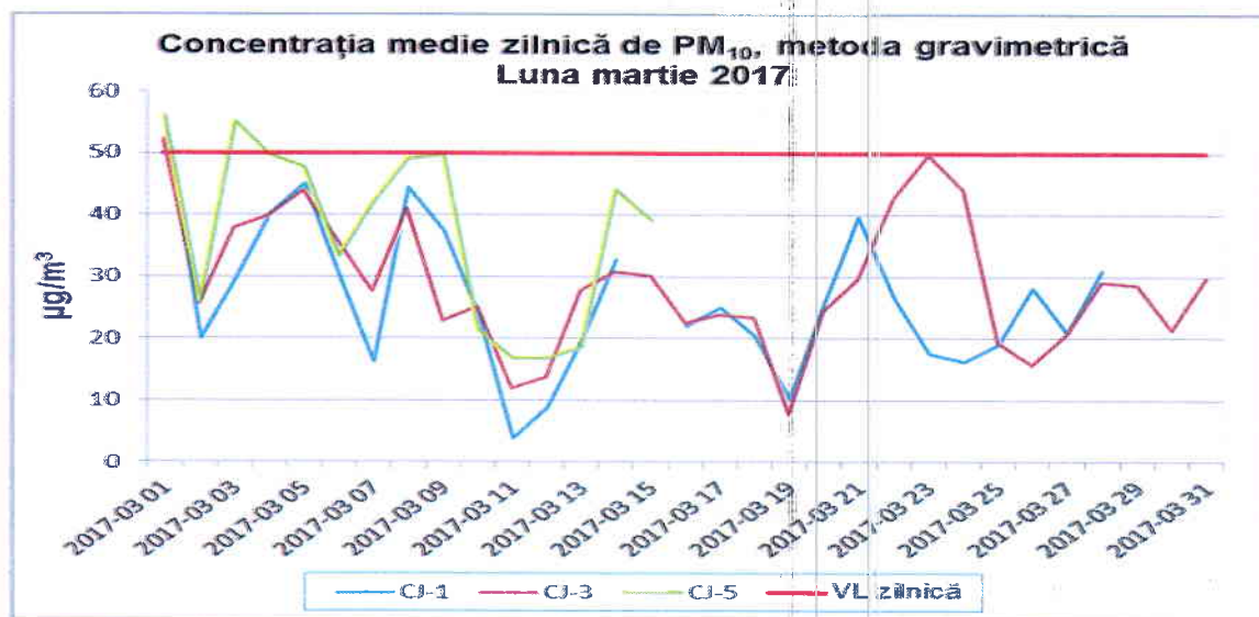
Figura 1.2.5.1. Evoluția mediilor zilnice de PM 10 , în luna martie 2017
