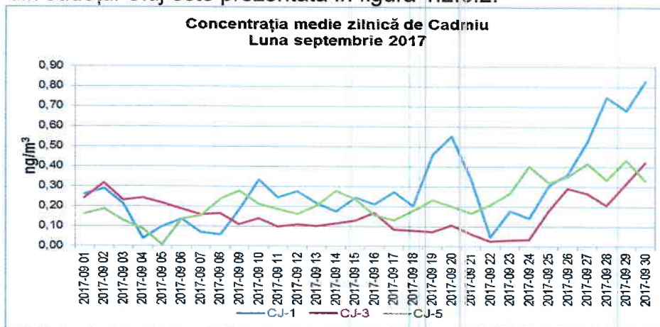
Figura 1.2.6.2. Evoluția mediilor zilnice de Cd, în luna septembrie 2017
