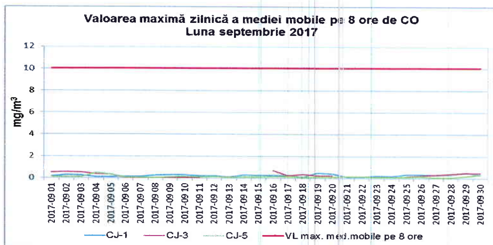
Figura 1.2.4.1. Evoluția maximelor zilnice ale mediilor mobile pe 8 ore de CO, în luna septembrie 2017
