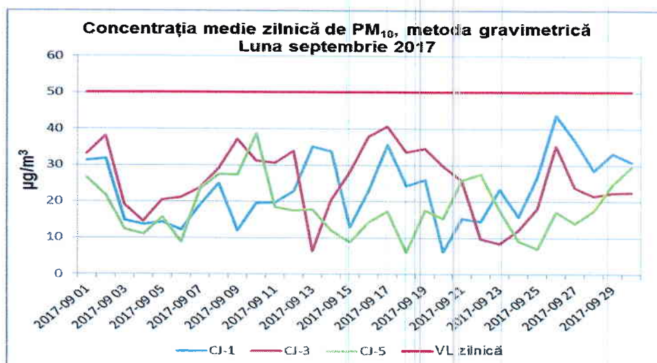
Figura 1.2.5.1. Evoluția mediilor zilnice de PM 10 , în luna septembrie 2017
