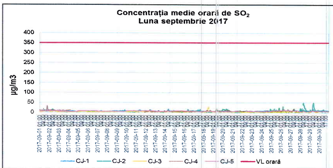
Figura 1.2.1.1. Evoluția mediilor orare de SO 2 în luna septembrie 2017
