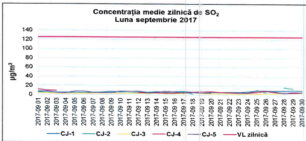
Figura 1.2.1.1. Evoluția mediilor zilnice de SO 2 în luna septembrie 2017
