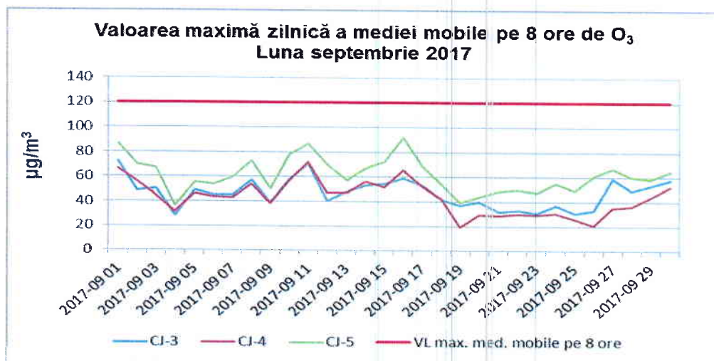
Figura 1.2.3.1. Evoluția maximelor zilnice ale mediilor mobile pe 8 ore de O 3 , în luna septembrie 2017
