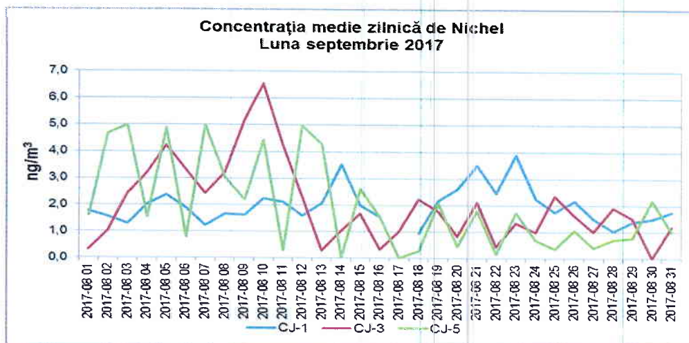
Figura 1.2.6.3. Evoluția mediilor zilnice de Ni, în luna septembrie 2017
