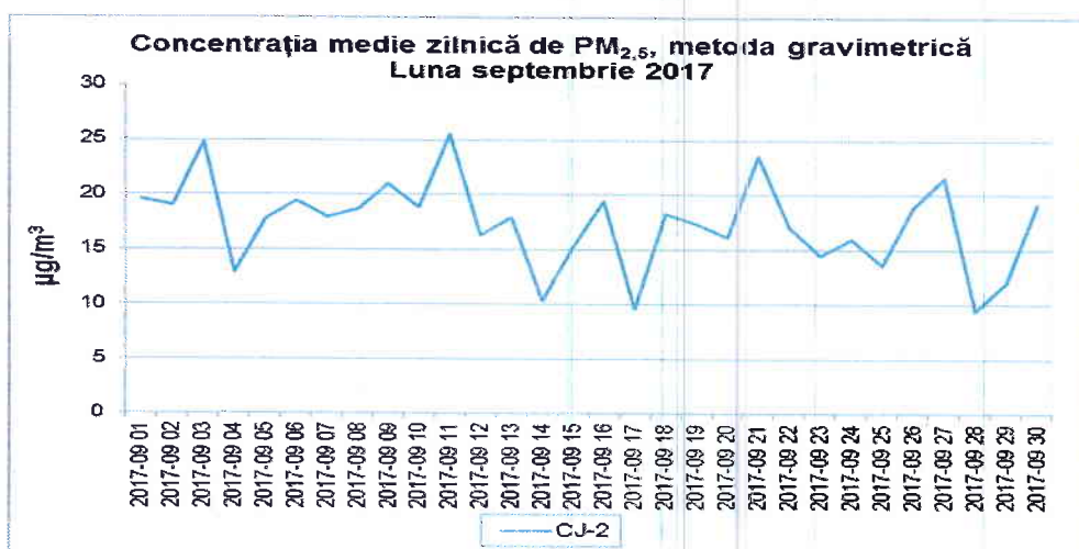
Figura 1.2.5.2. Evoluția mediilor zilnice de PM 10 , în luna septembrie 2017
