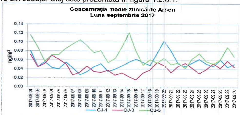
Figura 1.2.6.1. Evoluția mediilor zilnice de As, în luna septembrie 2017
