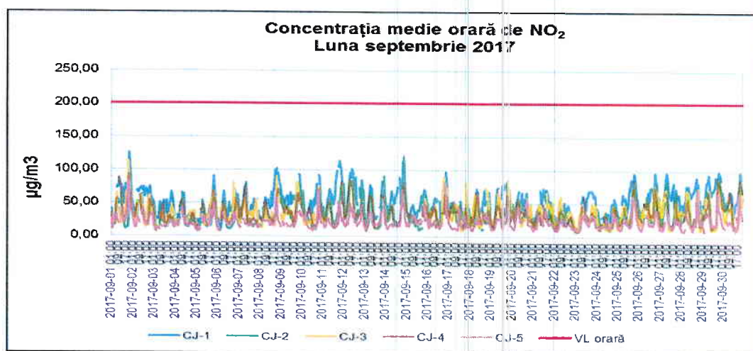
Figura 1.2.2.1. Evoluția mediilor orare de NO 2 în luna septembrie 2017
