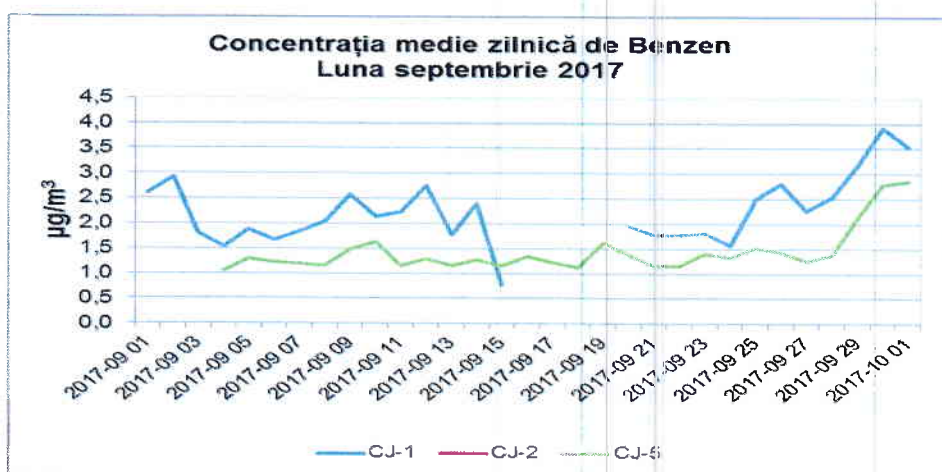
Figura 1.2.7.1. Evoluția mediilor zilnice de benzen, în luna septembrie 2017
