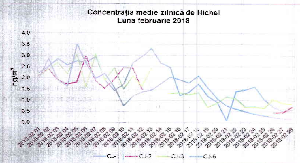
Figura 1.2.6.3. Evoluția mediilor zilnice de Ni, în luna februarie 2018
