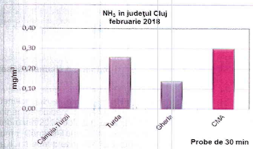
Figura 1.1.1. Rezultatele monitorizării amoniacului
