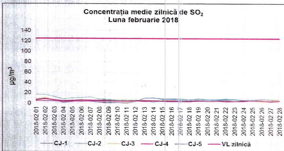
Figura 1.2.1.1. Evoluția mediilor zilnice de SO 2 în luna februarie 2018
