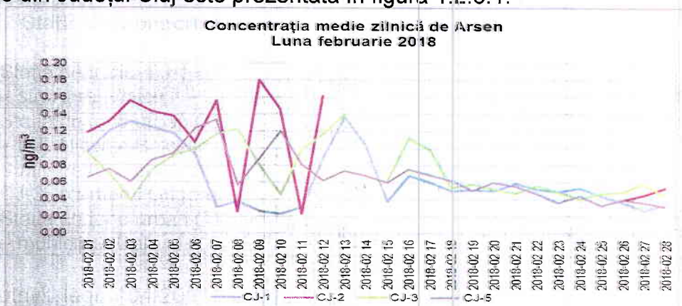
Figura 1.2.6.1. Evoluția mediilor zilnice de As, în luna februarie 2018
