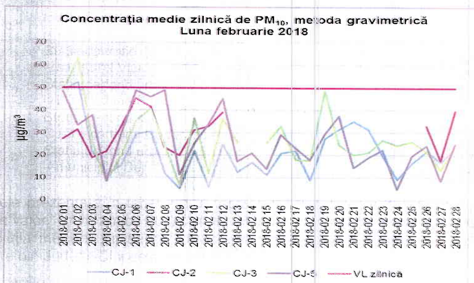
Figura 1.2.5.1. Evoluția mediilor zilnice de PM 10 , în luna februarie 2018
