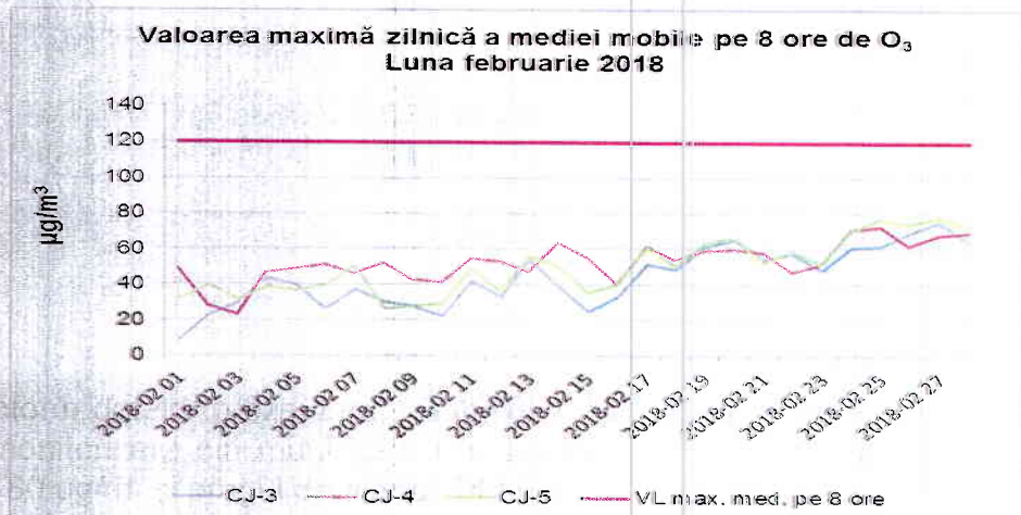
Figura 1.2.3.1. Evoluția maximelor zilnice ale mediilor mobile pe 8 ore de \text{O}_3 , în luna februarie 2018
