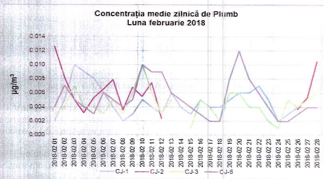
Figura 1.2.6.4. Evoluția mediilor zilnice de Pb, în luna februarie 2018
