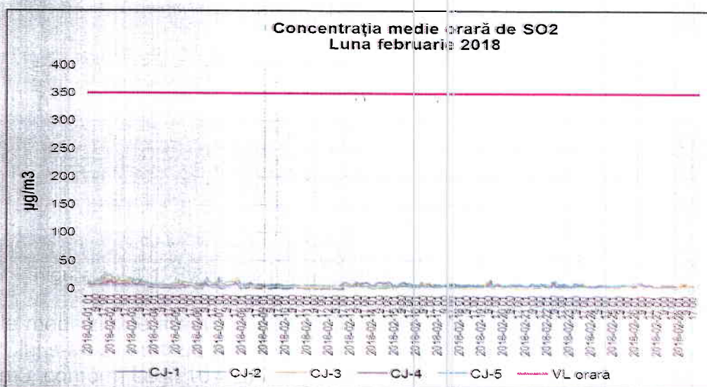
Figura 1.2.1.1. Evoluția mediilor orare de SO 2 în luna februarie 2018
