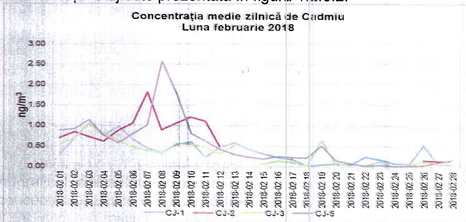
Figura 1.2.6.2. Evoluția mediilor zilnice de Cd, în luna februarie 2018
