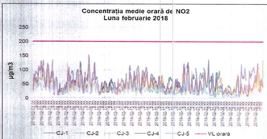
Figura 1.2.2.1. Evoluția mediilor orare de NO 2 în luna februarie 2018
