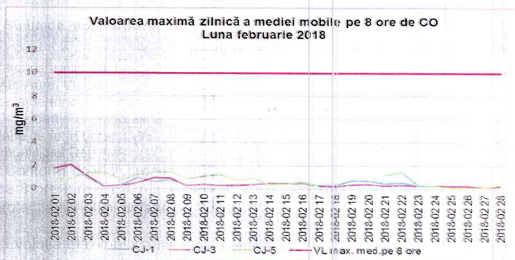
Figura 1.2.4.1. Evoluția maximelor zilnice ale mediilor mobile pe 8 ore de CO, în luna februarie 2018
