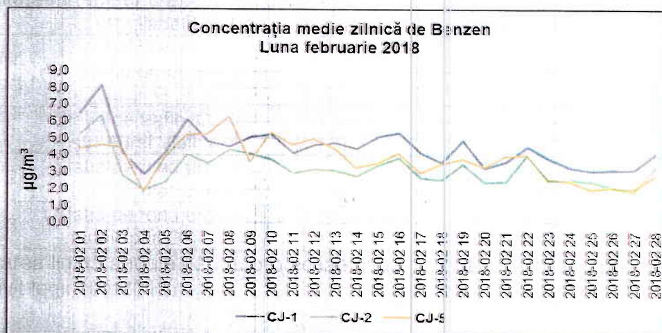
Figura 1.2.7.1. Evoluția mediilor zilnice de benzen, în luna februarie 2018
