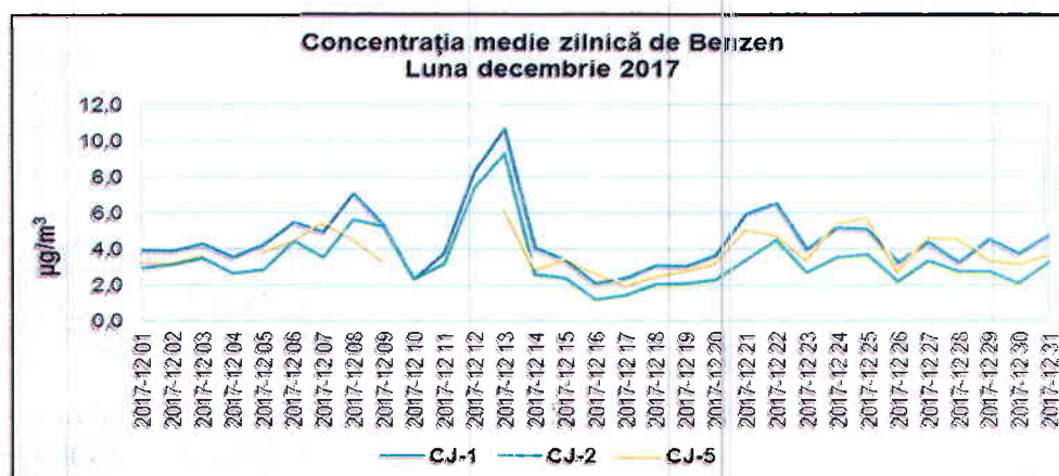
Figura 1.2.7.1. Evoluția mediilor zilnice de benzen, în luna decembrie 2017
