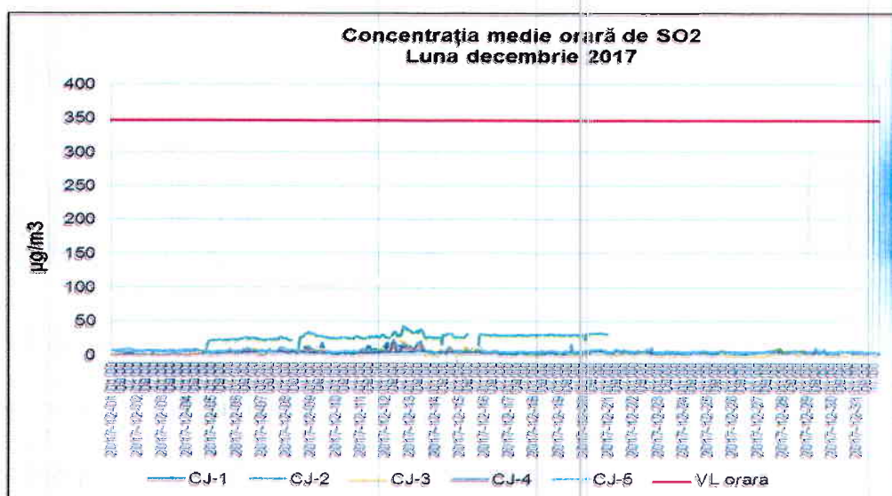
Figura 1.2.1.1. Evoluția mediilor orare de SO 2 în luna decembrie 2017
