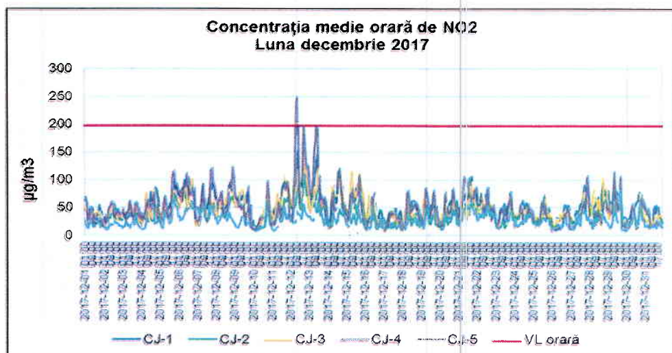
Figura 1.2.2.1. Evoluția mediilor orare de NO 2 în luna decembrie 2017
