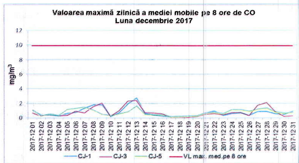
Figura 1.2.4.1. Evoluția maximelor zilnice ale mediilor mobile pe 8 ore de CO, în luna decembrie 2017
