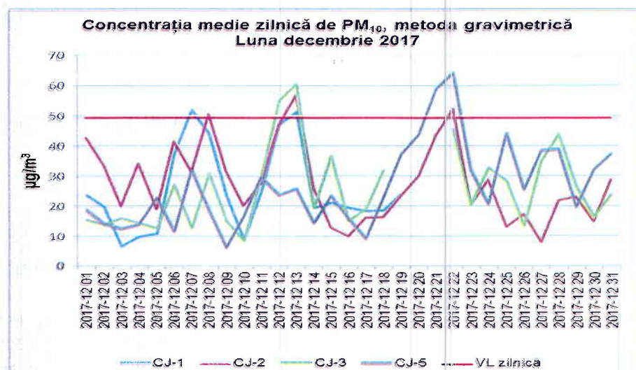
Figura 1.2.5.1. Evoluția mediilor zilnice de PM 10 , în luna decembrie 2017
