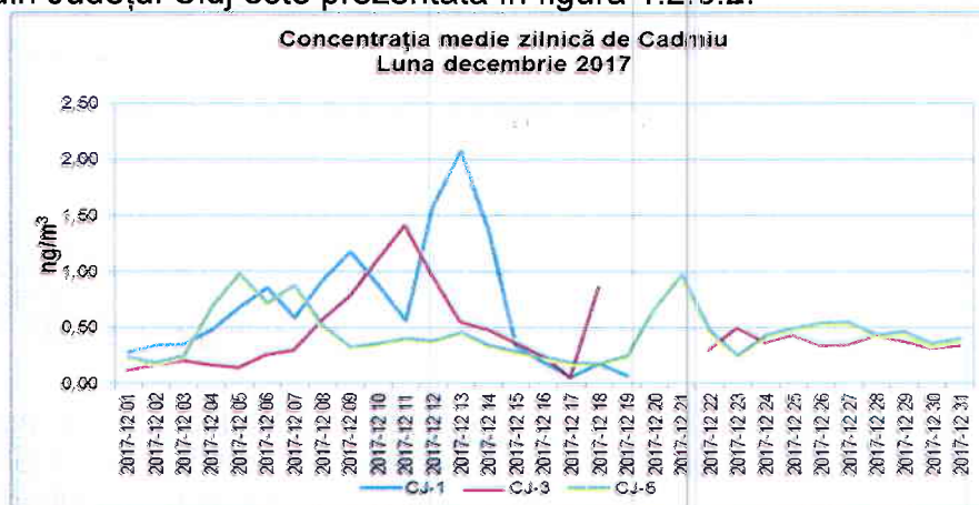
Figura 1.2.6.2. Evoluția mediilor zilnice de Cd, în luna decembrie 2017
