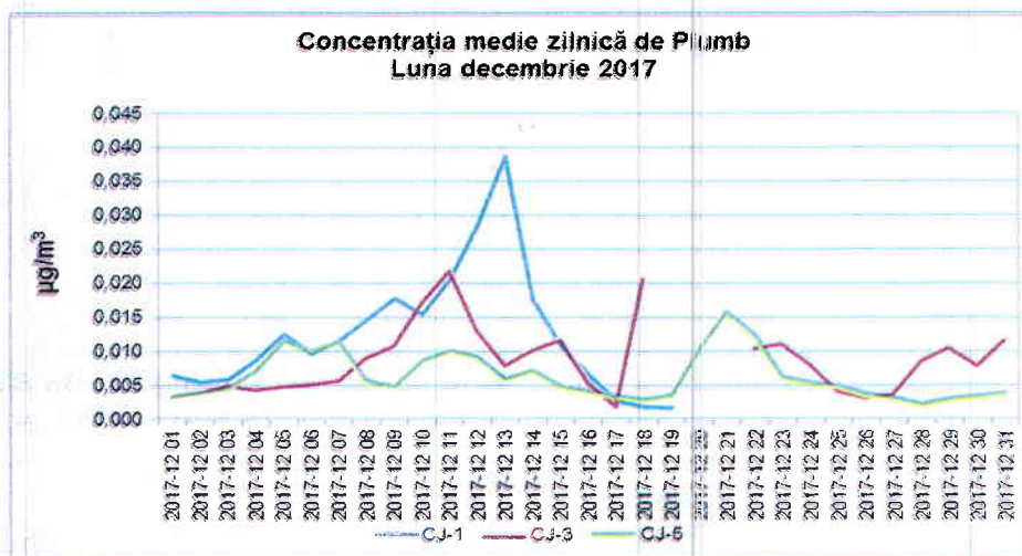
Figura 1.2.6.4. Evoluția mediilor zilnice de Pb, în luna decembrie 2017
