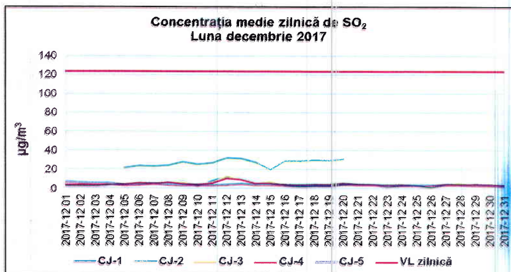
Figura 1.2.1.1. Evoluția mediilor zilnice de SO 2 în luna decembrie 2017
