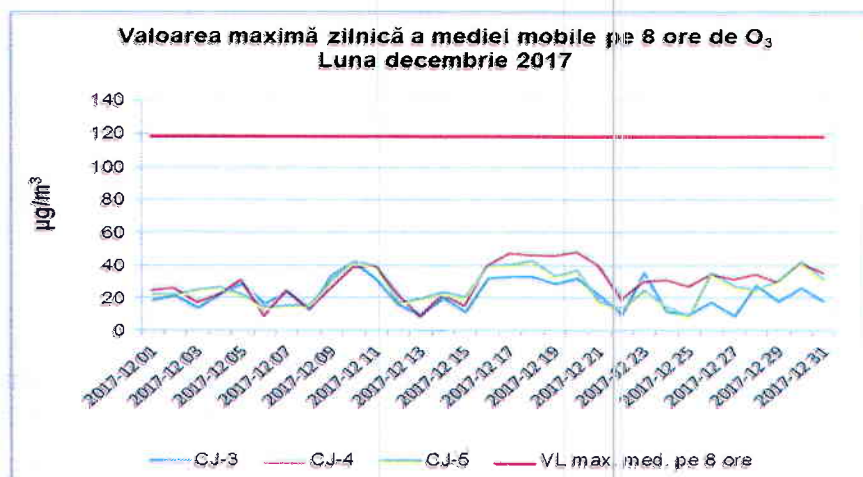
Figura 1.2.3.1. Evoluția maximelor zilnice ale mediilor mobile pe 8 ore de \text{O}_3 , în luna decembrie 2017
