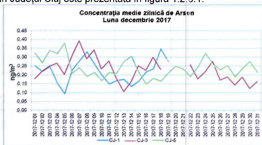
Figura 1.2.6.1. Evoluția mediilor zilnice de As, în luna decembrie 2017
