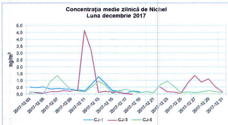
Figura 1.2.6.3. Evoluția mediilor zilnice de Ni, în luna decembrie 2017
