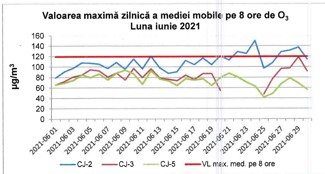
Figura 1.2.3.1. Evoluția maximelor zilnice ale mediilor mobile pe 8 ore de \text{O}_3 , în județul Cluj, în luna iunie 2021
