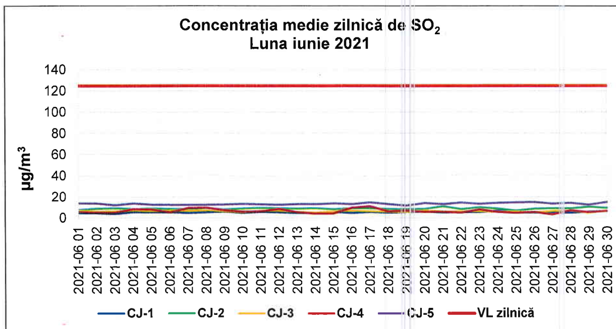
Figura 1.2.1.1. Evoluția concentrației medii zilnice de SO 2 În județul Cluj în luna iunie 2021
