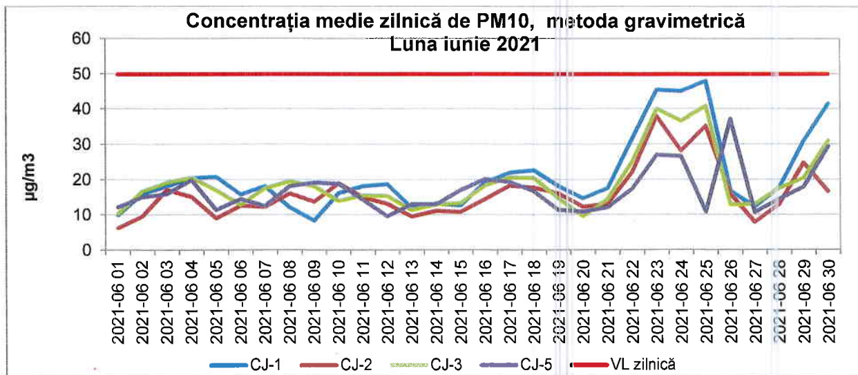
Figura 1.2.5.1. Evoluția concentrației medii zilnice de \text{PM}_{10} , în județul Cluj, în luna iunie 2021
