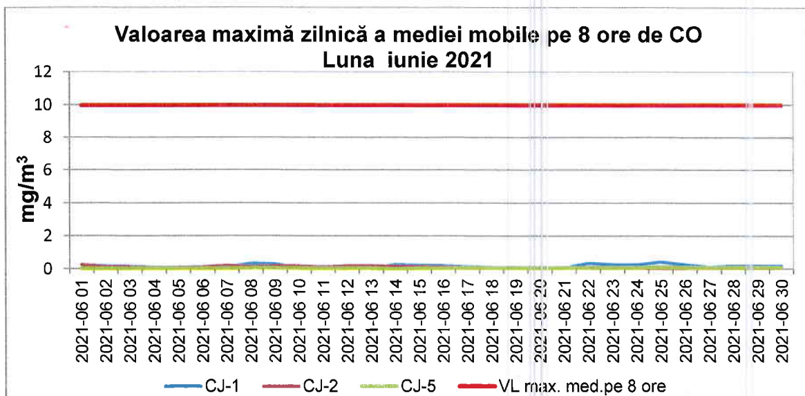
Figura 1.2.4.1. Evoluția concentrațiilor maxime zilnice a mediilor mobile pe 8 ore de CO, în județul Cluj, în luna iunie 2021
