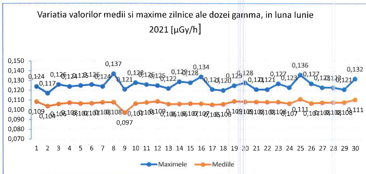
Figura nr. 3.1.1 Variația valorilor medii și maxime zilnice ale debitului dozei gamma în luna iunie 2021
