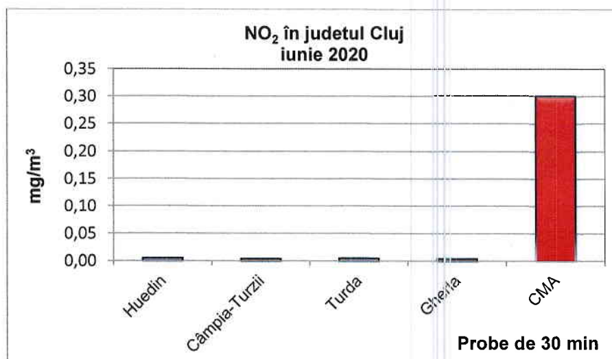
Figura 1.1.2. Evoluția concentrației de dioxid de azot în județul Cluj în luna iunie 2021
