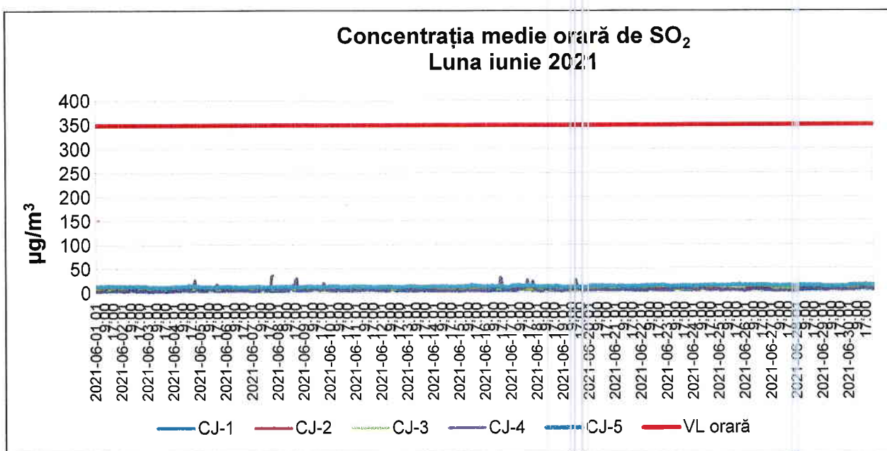
Figura 1.2.1.2. Evoluția concentrației medii orare de SO 2 În județul Cluj în luna iunie 2021
