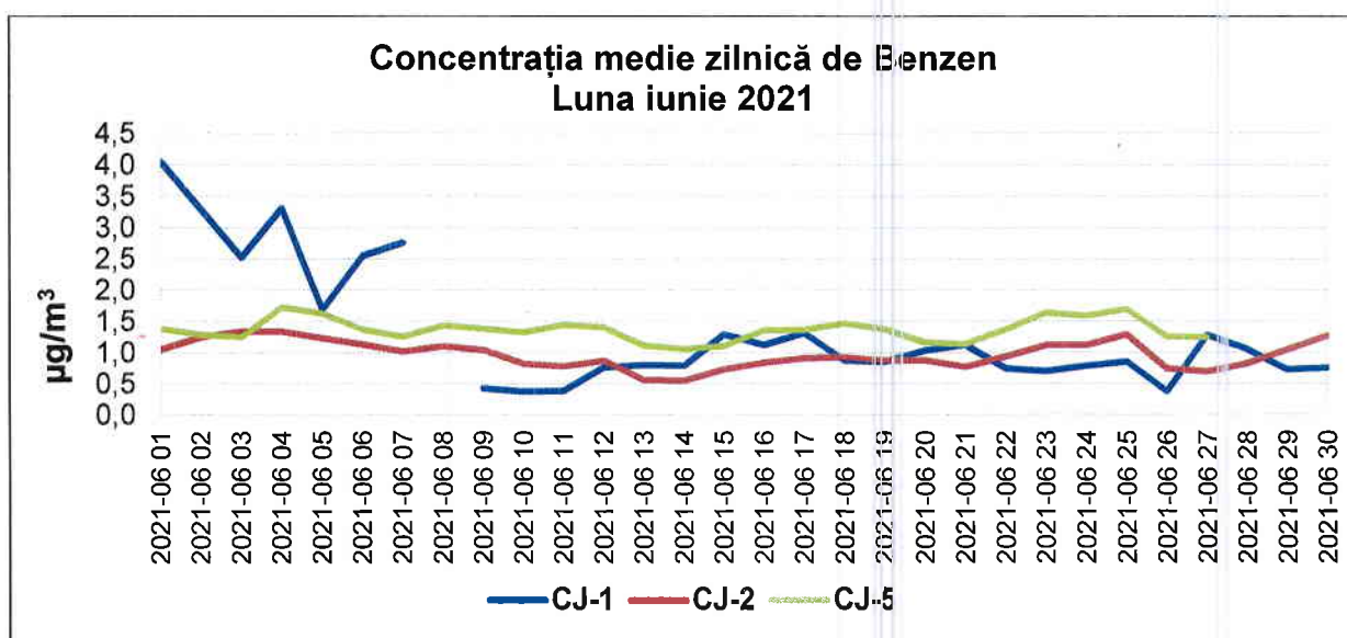
Figura 1.2.7.1. Evoluția concentrației medii zilnice de benzen în județul Cluj, în luna iunie 2021
