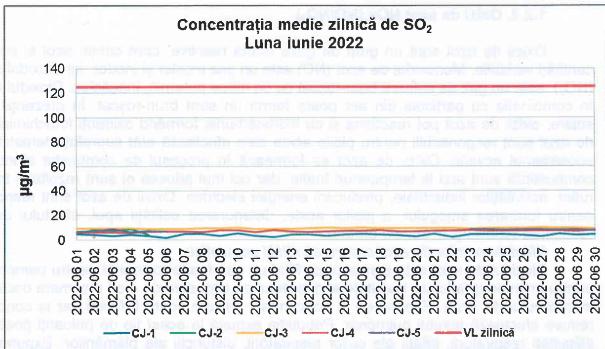
Figura 1.2.1.1. Evoluția concentrației medii zilnice de SO 2 în județul Cluj în luna iunie 2022
