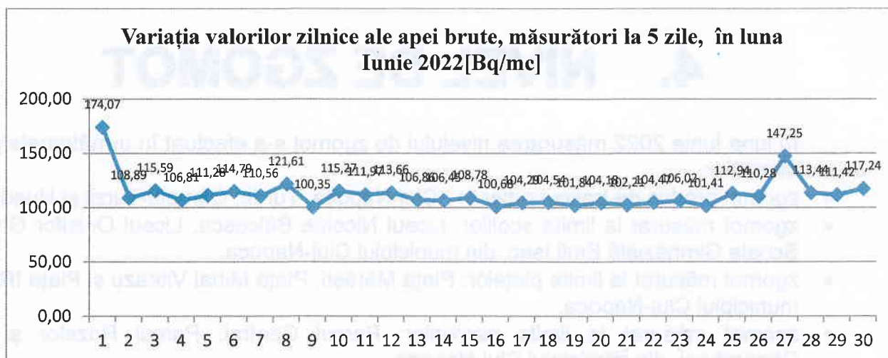
Figura nr. 3.4.1.2.1 Variația valorilor zilnice ale apei brute, măsurări la 5 zile, luna Iunie 2022
