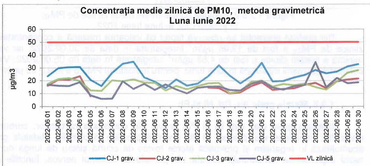
Figura 1.2.5.1. Evoluția concentrației medii zilnice de \text{PM}_{10} , în județul Cluj, în luna Iunie 2022
