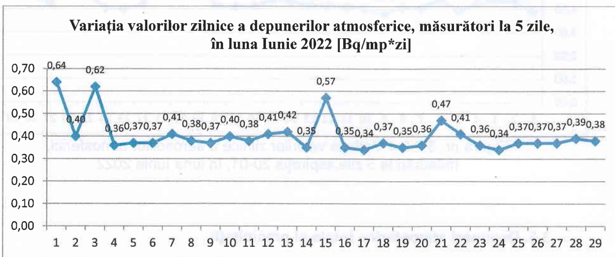
Figura nr. 3.3.2.1 Variația valorilor zilnice a depunerilor atmosferice, măsurări la 5 zile, luna Iunie 2022 [Bq/mp*zi]
