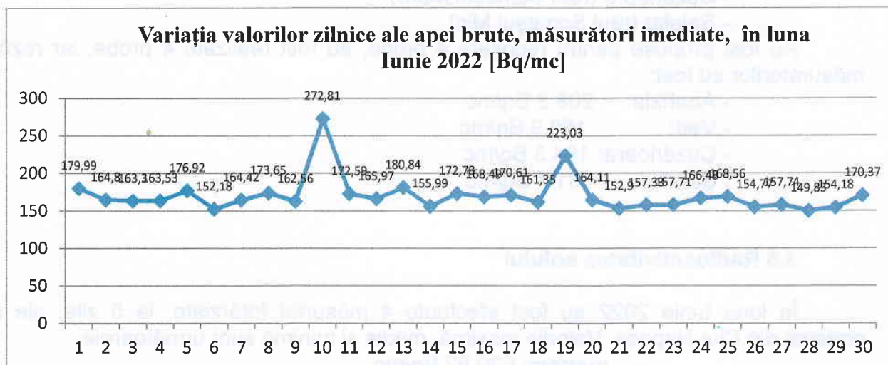
Figura nr. 3.4.1.1.1 Variația valorilor zilnice ale apei brute, măsurări imediate, luna Iunie 2022
