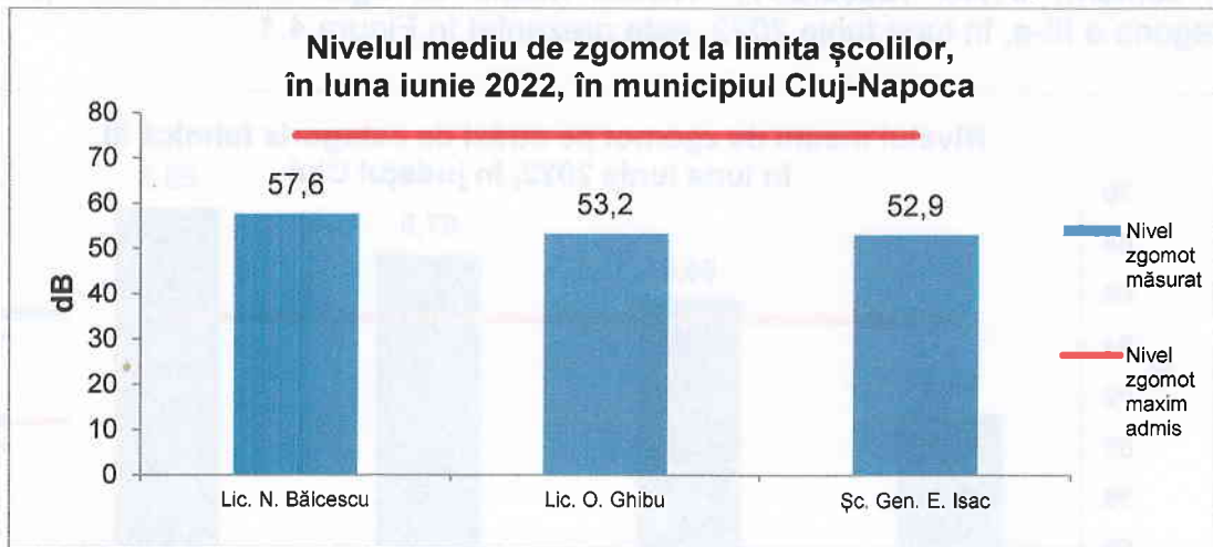
Figura 4.3. Nivelul de zgomot la limita școlilor, în luna iunie 2022
