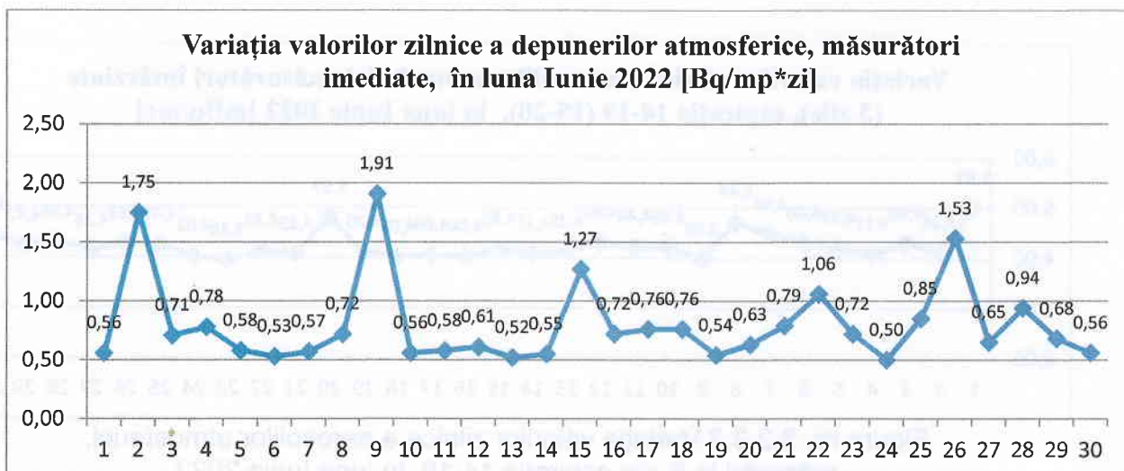
Figura nr. 3.3.1.1 Variația valorilor zilnice a depunerilor atmosferice, măsurări imediate, luna Iunie 2022 [Bq/mp*zi]
