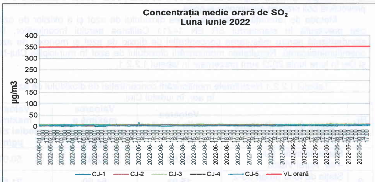
Figura 1.2.1.2. Evoluția concentrației medii orare de SO 2 în județul Cluj în luna iunie 2022
