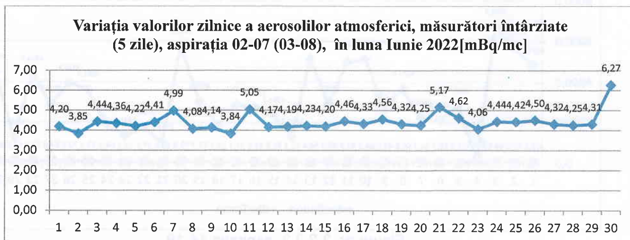
Figura nr. 3.2.3.1 Variația valorilor zilnice a aerosolilor atmosferici, măsurări la 5 zile, aspirația 03-08, în luna Iunie 2022
