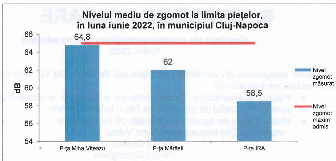
Figura 4.5. Nivelul de zgomot la limita piețelor, în luna Iunie 2022
