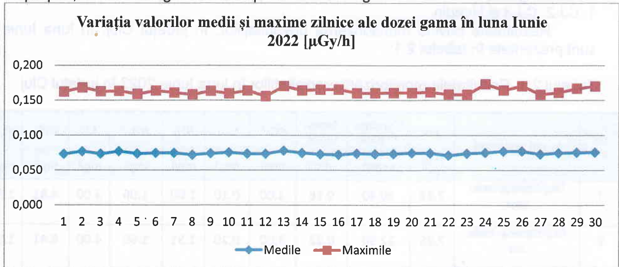
Figura nr. 3.1.1 Variația valorilor medii și maxime zilnice ale debitului dozei gamma în luna Iunie 2022
