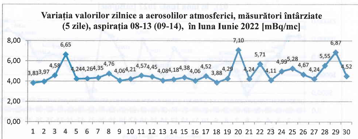
Figura nr. 3.2.3.2 Variația valorilor zilnice a aerosolilor atmosferici, măsurări la 5 zile, aspirația 08-13, în luna Iunie 2022
