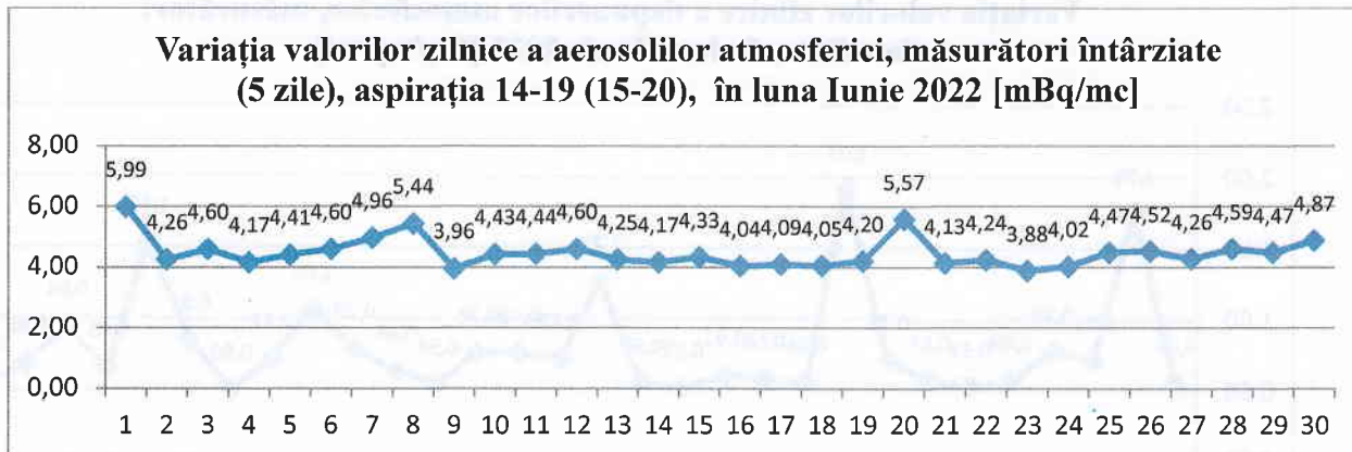
Figura nr. 3.2.3.3 Variația valorilor zilnice a aerosolilor atmosferici, măsurări la 5 zile, aspirația 14-19, în luna Iunie 2022
