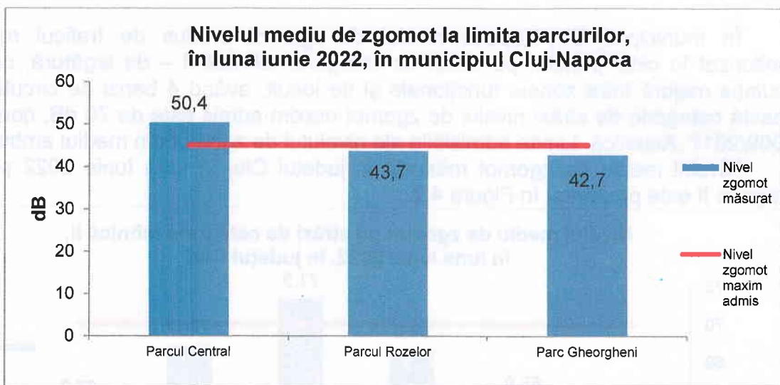
Figura 4.4. Nivelul de zgomot la limita parcurilor, în luna iunie 2022
