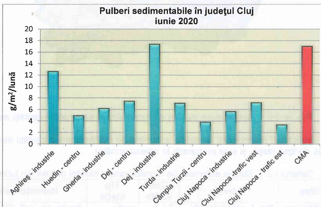
Figura 1.1.4. Evoluția concentrației de pulveri sedimentabile în județul Cluj în luna iunie 2022
