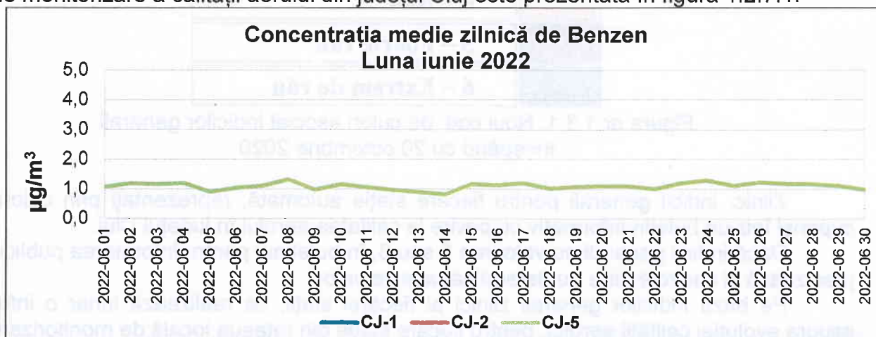
Figura 1.2.7.1. Evoluția concentrației medii de zilnice de benzen în județul Cluj, în luna Iunie 2022
