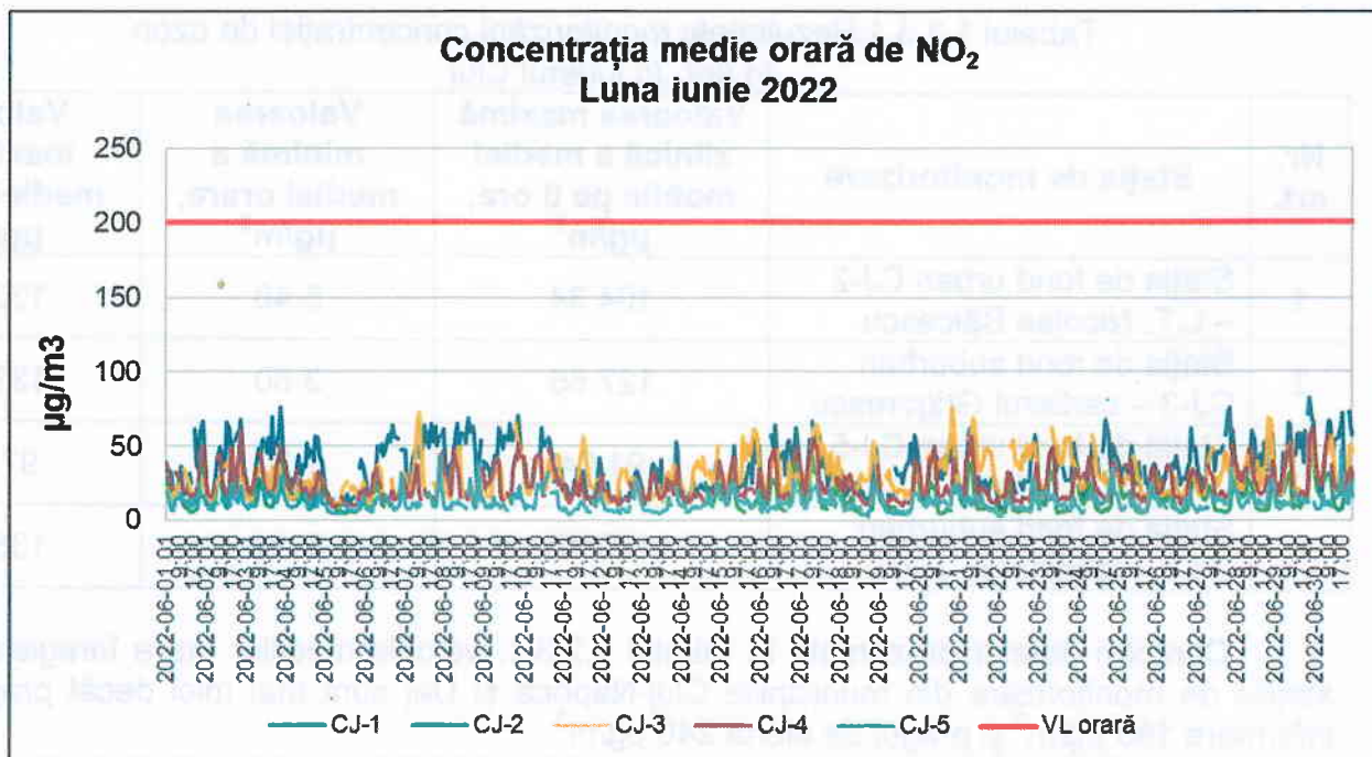
Figura 1.2.2.1. Evoluția concentrațiilor medii orare de \text{NO}_2 în județul Cluj în luna Iunie 2022
