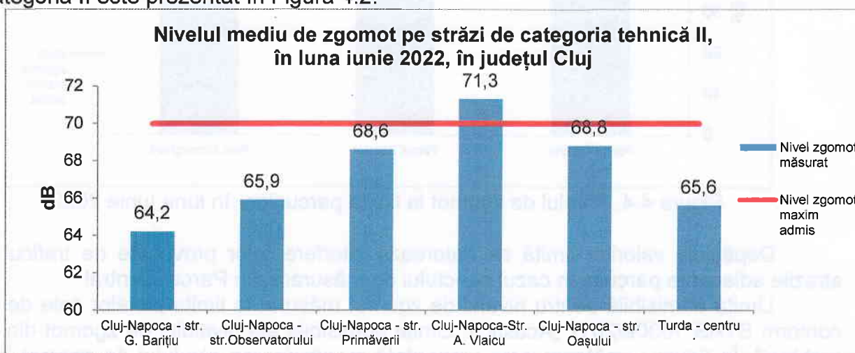
Figura 4.2. Nivelul de zgomot urban pe străzi de categoria II, în județul Cluj, în luna iunie 2022
