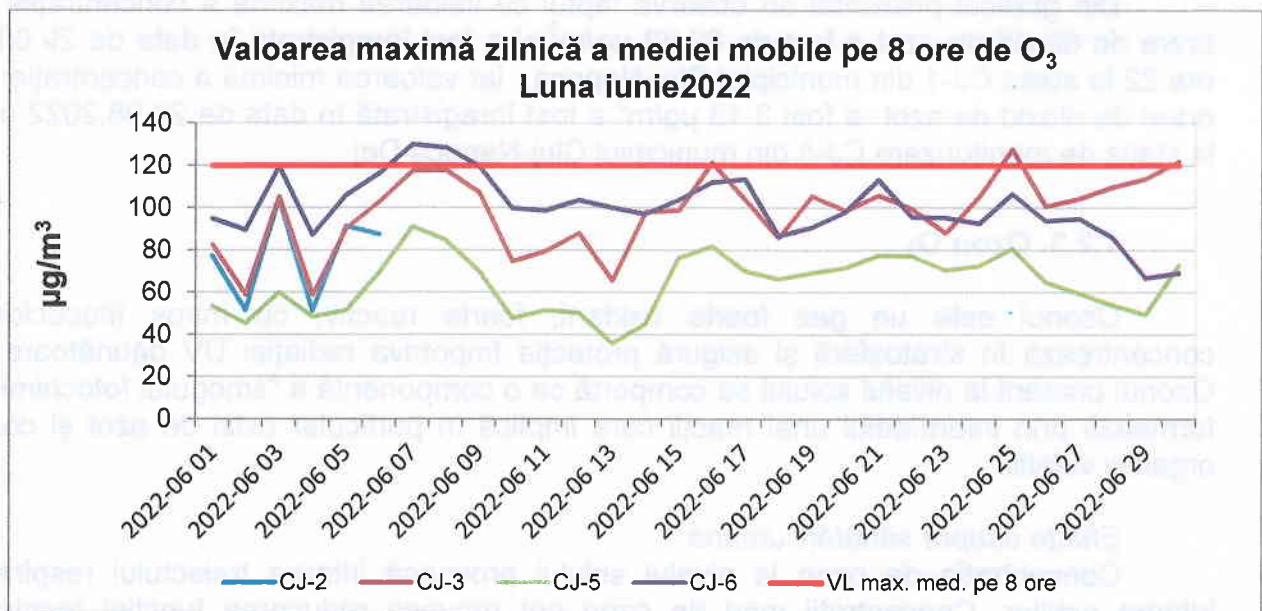
Figura 1.2.3.1. Evoluția maximelor zilnice ale mediilor mobile pe 8 ore de \text{O}_3 , în județul Cluj, în luna iunie 2022
