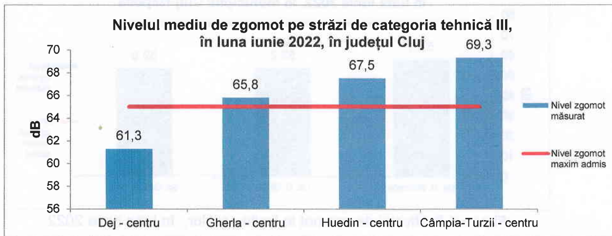
Figura 4.1. Nivelul de zgomot urban pe strazi de categoria III, în județul Cluj, în luna iunie 2022
