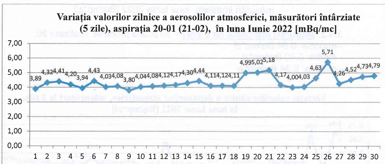
Figura nr. 3.2.3.4 Variația valorilor zilnice a aerosolilor atmosferici, măsurări la 5 zile, aspirația 20-01, în luna Iunie 2022
