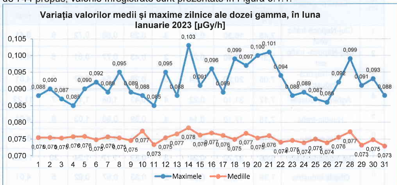
Figura nr. 3.1.1 Variația valorilor medii și maxime zilnice ale debitului dozei gamma în luna ianuarie 2023
