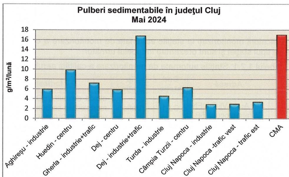
Fig. nr. 1.1.1- Evoluția concentrației de pulberi sedimentabile în județul Cluj, în luna mai 2024
