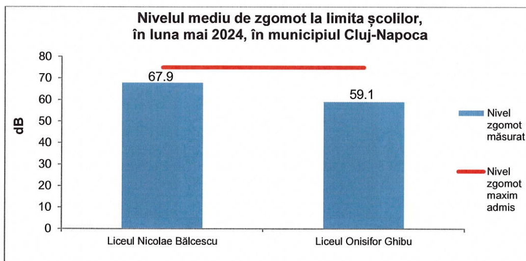
Fig. nr. 4.1. Nivelul de zgomot la limita școlilor, în luna mai 2024
