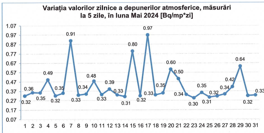
Fig. nr. 3.3.2.1-Variația valorilor zilnice a depunerilor atmosferice, măsurări la 5 zile, luna mai 2024[Bq/mp*zi]
