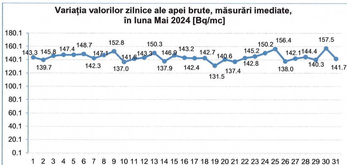
Fig. nr. 3.4.1.1.1-Variația valorilor zilnice ale apei brute, măsurări imediate, luna mai 2024
