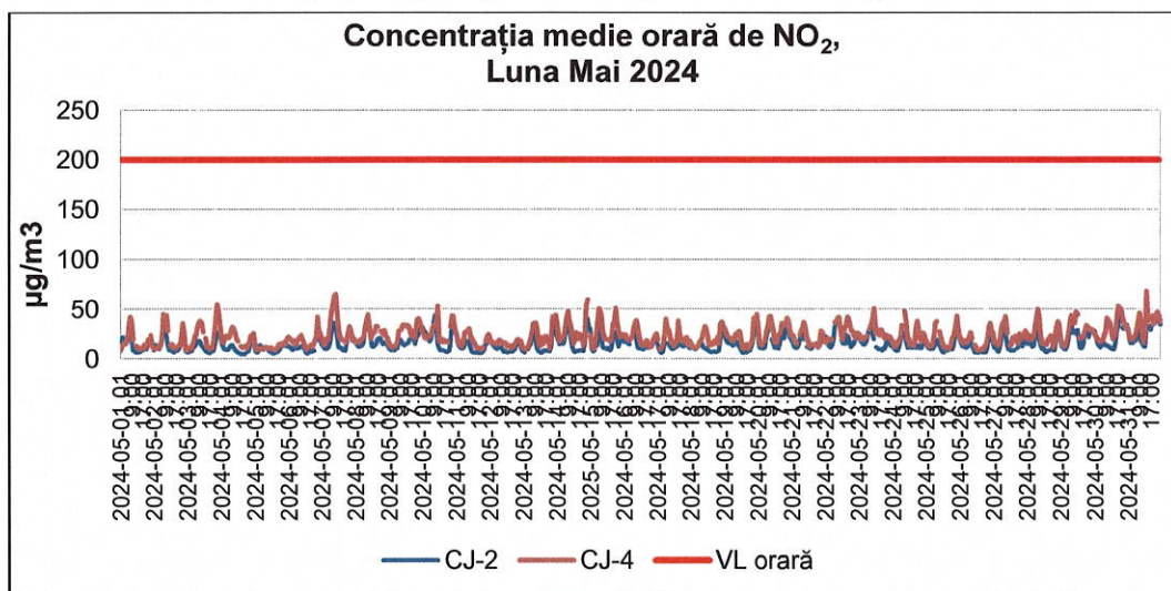
Fig. nr. 1.2.2.1. Evoluția concentrațiilor medii orare de \text{NO}_2 în județul Cluj în luna mai 2024
