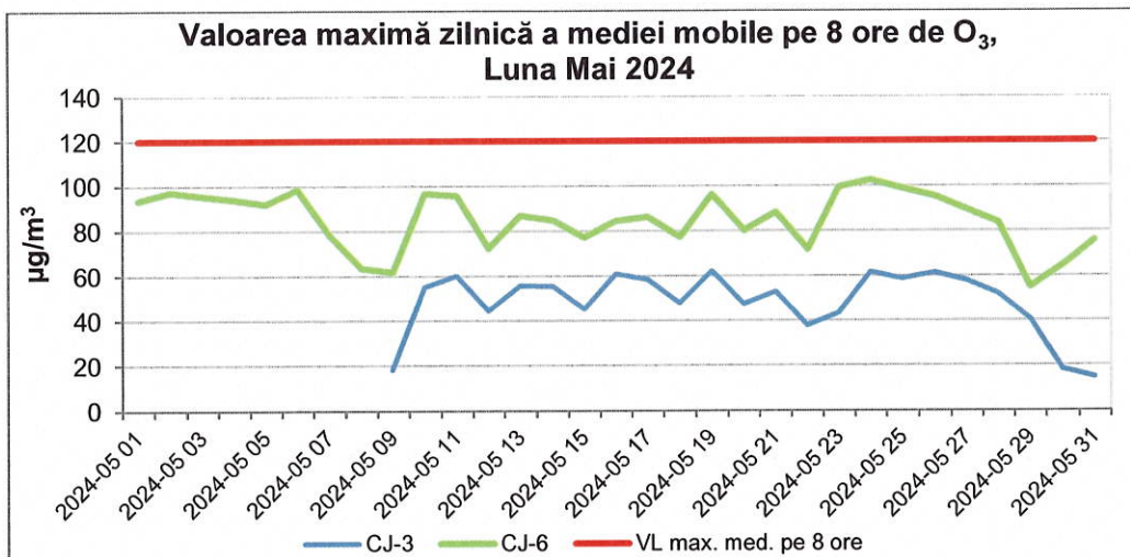
Fig. nr. 1.2.3.1. Evoluția maximelor zilnice ale mediilor mobile pe 8 ore de O 3 , în luna mai 2024
