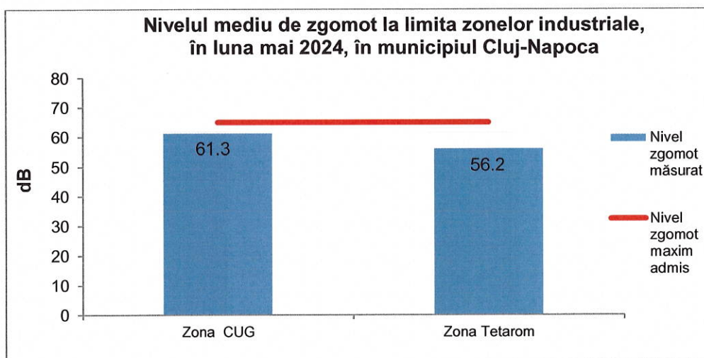
Fig. nr. 4.4. Nivelul de zgomot la limita zonelor industriale, în luna mai 2024
