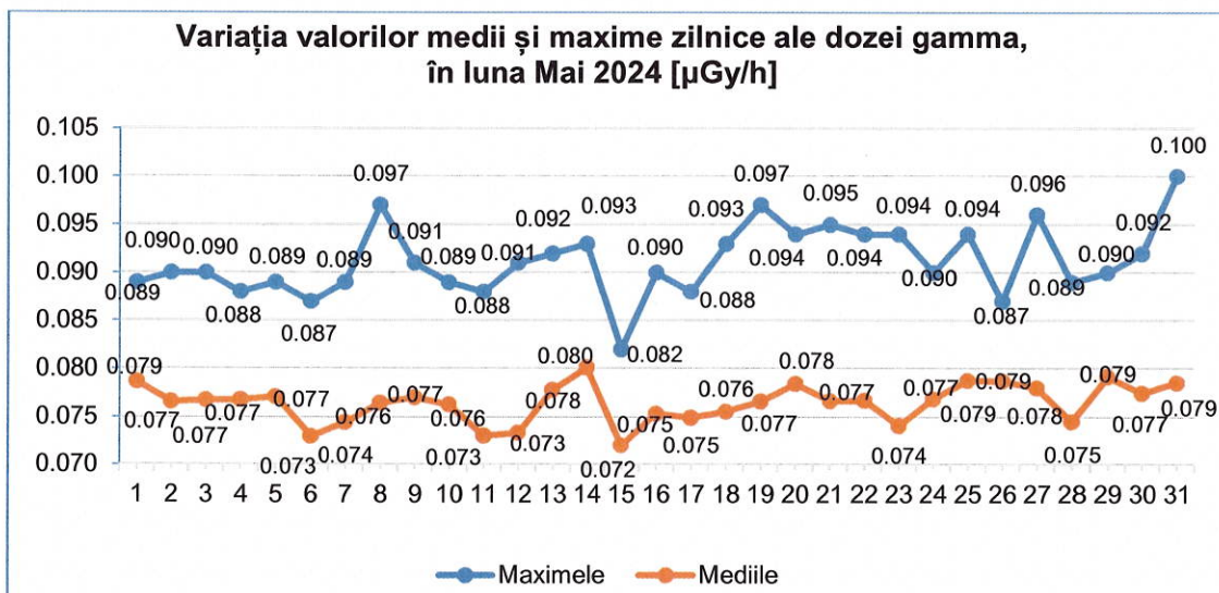
Fig. nr. 3.1.1 Variația valorilor medii și maxime zilnice ale debitului dozei gamma, în luna mai 2024
