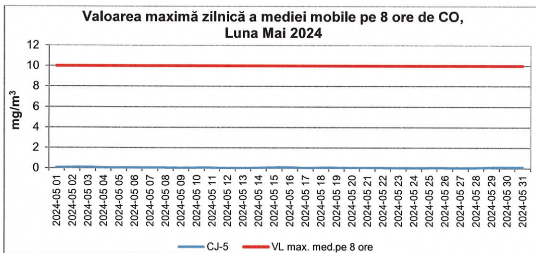
Fig. nr. 1.2.4.1. Evoluția maximelor zilnice ale mediilor mobile pe 8 ore de CO, în județul Cluj, în luna mai 2024
