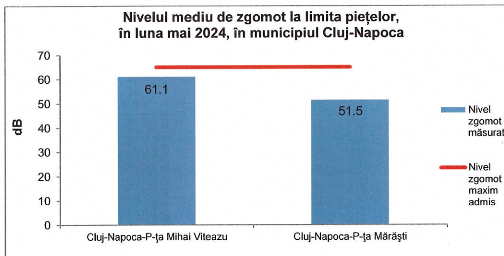
Fig. nr. 4.3. Nivelul de zgomot la limita piețelor, în luna mai 2024
