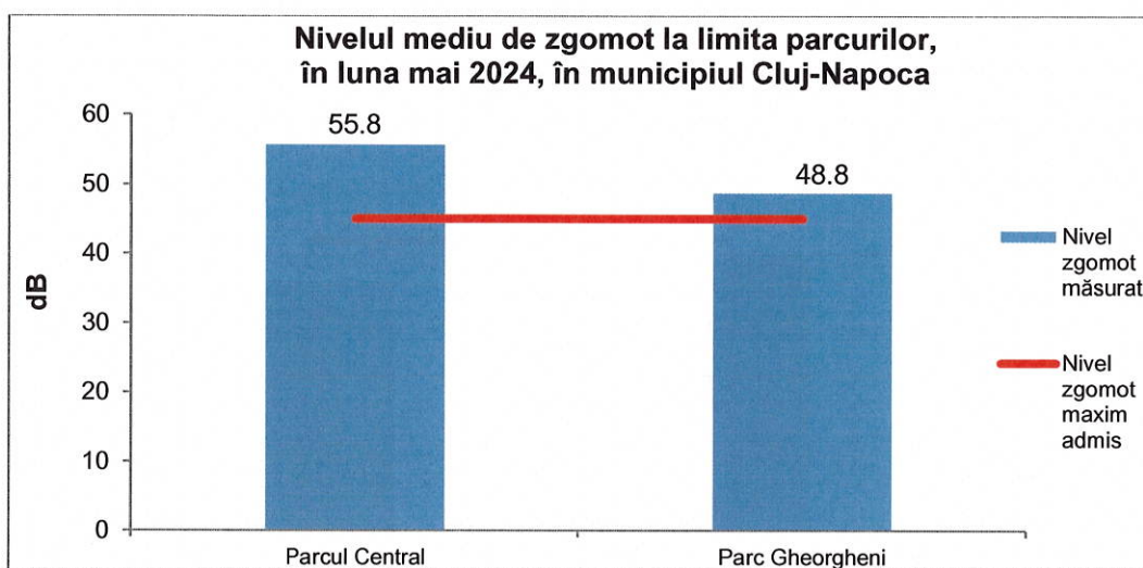
Fig. nr. 4.2. Nivelul de zgomot la limita parcurilor, în luna mai 2024
