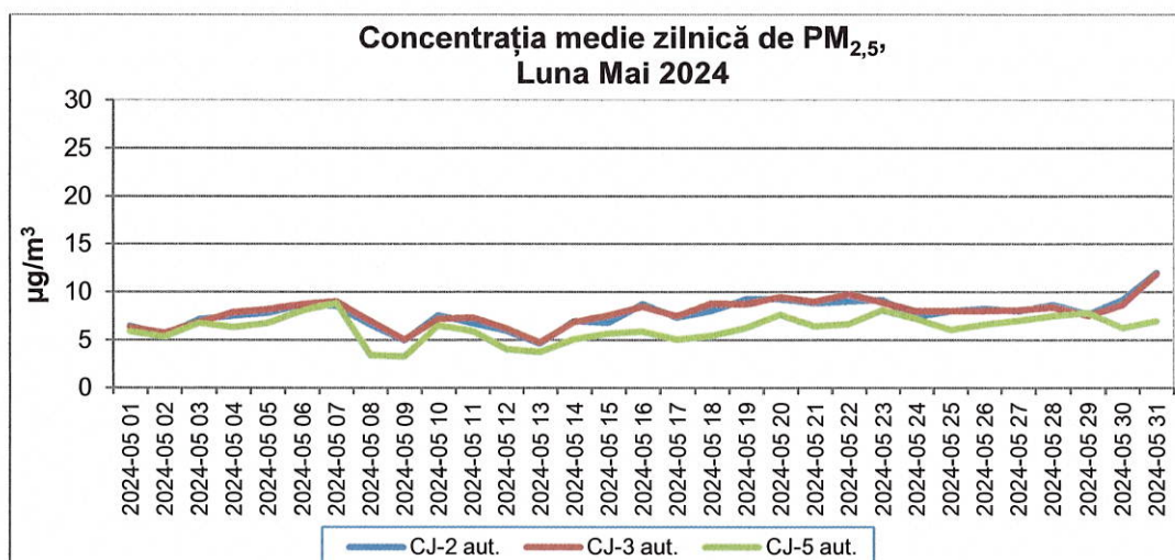
Fig. nr. 1.2.5.2. Evoluția concentrației medii zilnice de PM 2,5 , în județul Cluj, în luna mai 2024
