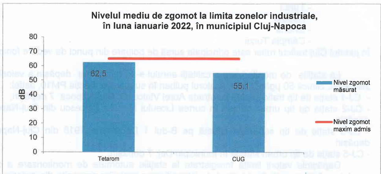
Figura 4.6. Nivelul de zgomot la limita zonelor industriale, în luna ianuarie 2022
