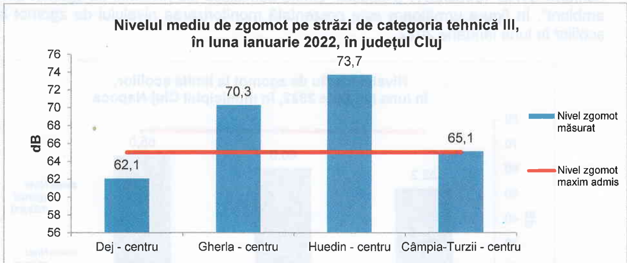
Figura 4.1. Nivelul de zgomot urban pe străzi de categoria III, în județul Cluj, în luna ianuarie 2022
