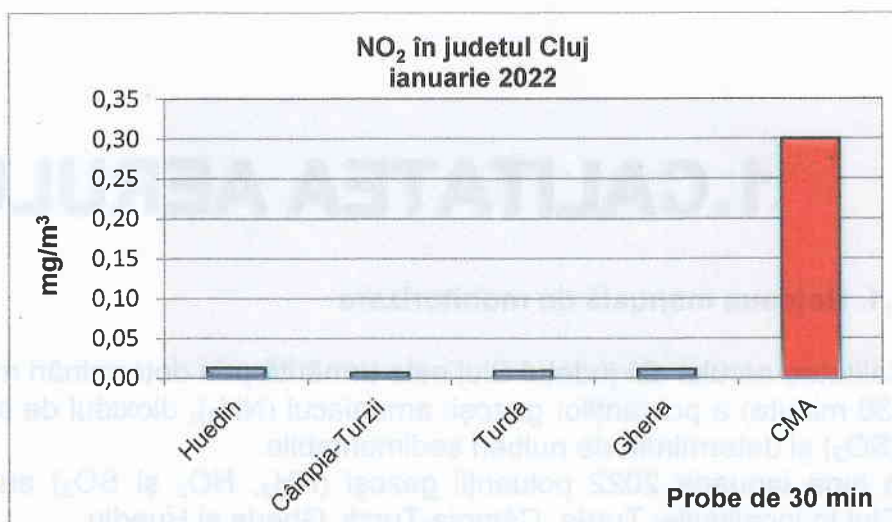
Figura 1.1.2. Evoluția concentrației de dioxid de azot în județul Cluj în luna ianuarie 2022
