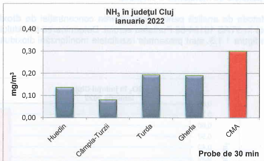
Figura 1.1.1. Evoluția concentrației de amoniac în județul Cluj în luna ianuarie 2022
