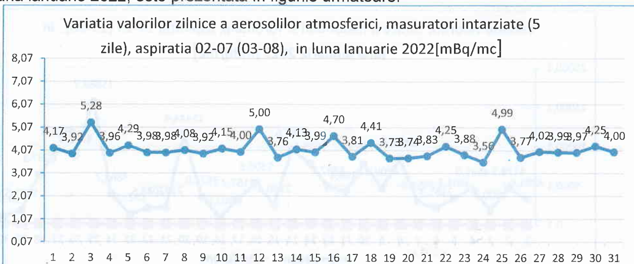
Figura nr. 3.2.3.1 Variația valorilor zilnice a aerosolilor atmosferici, măsurări la 5 zile, aspirația 02-07, în luna ianuarie 2022
