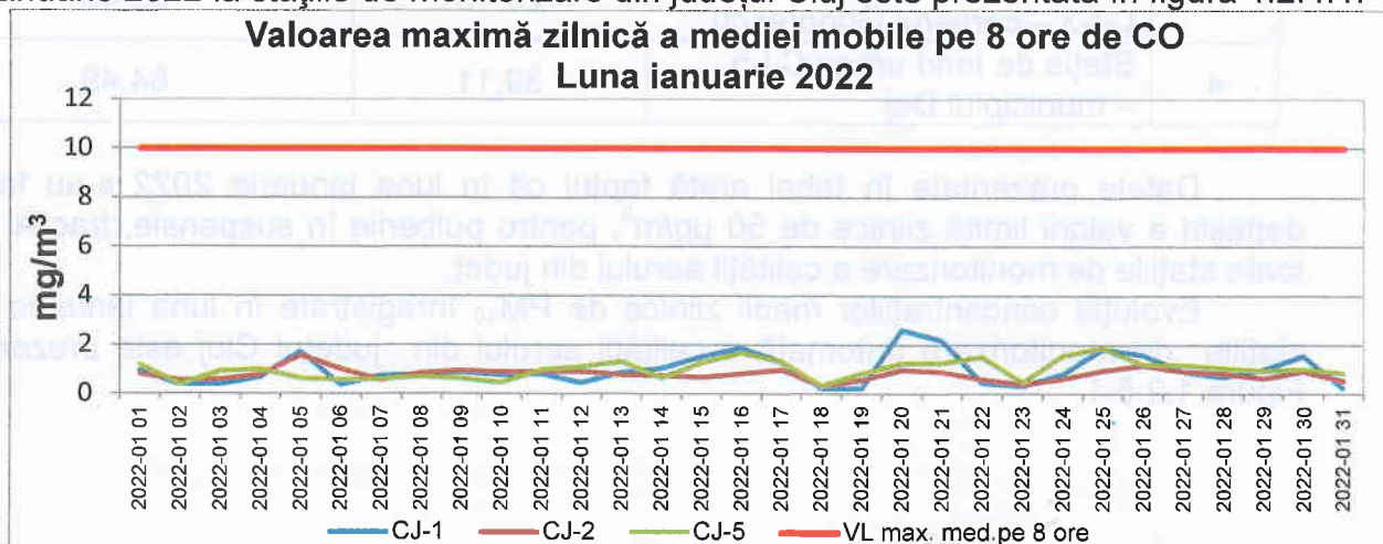
Figura 1.2.4.1. Evoluția concentrațiilor maxime zilnice a mediilor mobile pe 8 ore de CO, în județul Cluj, în luna ianuarie 2022
