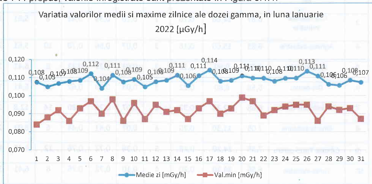
Figura nr. 3.1.1 Variația valorilor medii și maxime zilnice ale debitului dozei gamma în luna ianuarie 2022
