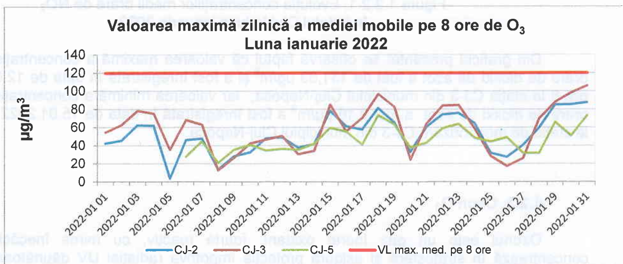
Figura 1.2.3.1. Evoluția maximelor zilnice ale mediilor mobile pe 8 ore de \text{O}_3 , în județul Cluj, în luna ianuarie 2022
