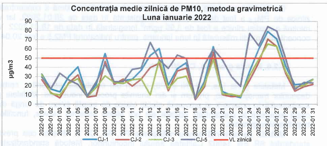
Figura 1.2.5.1. Evoluția concentrației medii zilnice de PM 10 , în județul Cluj, în luna ianuarie 2022
