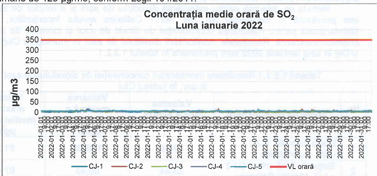
Figura 1.2.1.2. Evoluția concentrației medii orare de SO 2 în județul Cluj în luna ianuarie 2022
