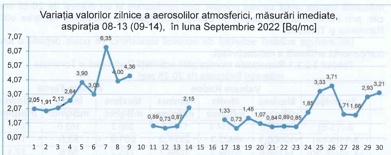
Figura nr. 3.2.1.2 aspirația 9-14
