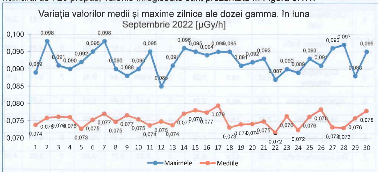
Figura nr. 3.1.1 Variația valorilor medii și maxime zilnice ale debitului dozei gamma în luna Septembrie 2022
