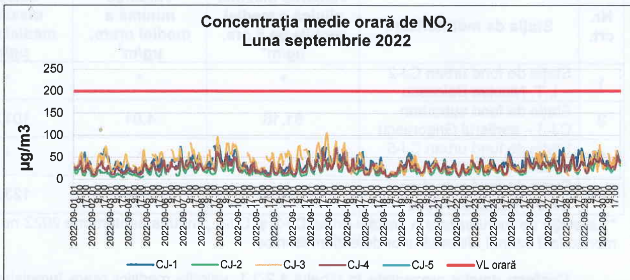
Figura 1.2.2.1. Evoluția concentrațiilor medii orare de \text{NO}_2 în județul Cluj în luna septembrie 2022
