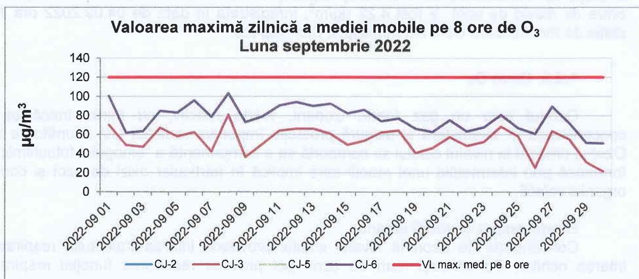
Figura 1.2.3.1. Evoluția maximelor zilnice ale mediilor mobile pe 8 ore de \text{O}_3 , în județul Cluj, în luna septembrie 2022
