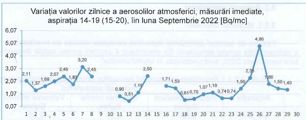
Figura nr. 3.2.1.3 aspirația 15-20
