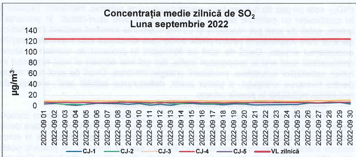
Figura 1.2.1.1. Evoluția concentrației medii zilnice de SO 2 în județul Cluj în luna septembrie 2022
