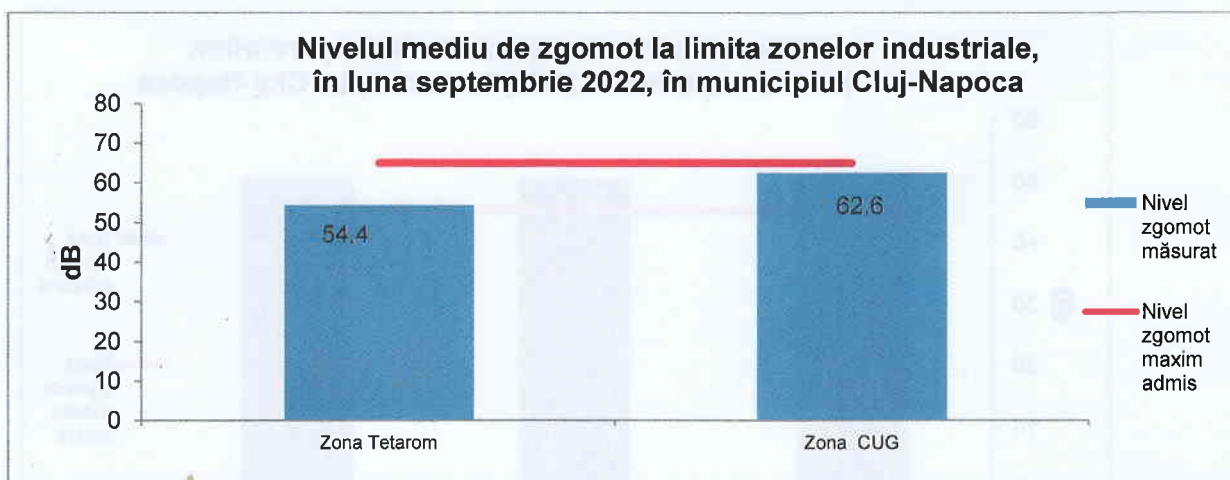
Figura 4.6. Nivelul de zgomot la limita zonelor industriale, în luna septembrie 2022
