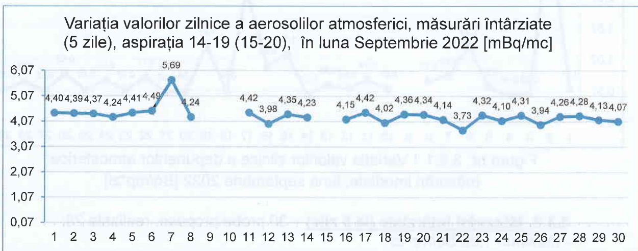
Figura nr. 3.2.3.3 Variația valorilor zilnice a aerosolilor atmosferici, măsurări la 5 zile, aspirația 14-19, în luna Septembrie 2022
