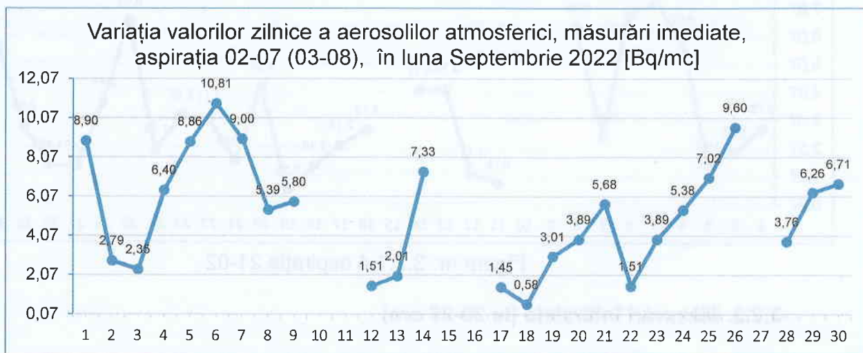
Figura nr. 3.2.1.1 aspirația 3-8
