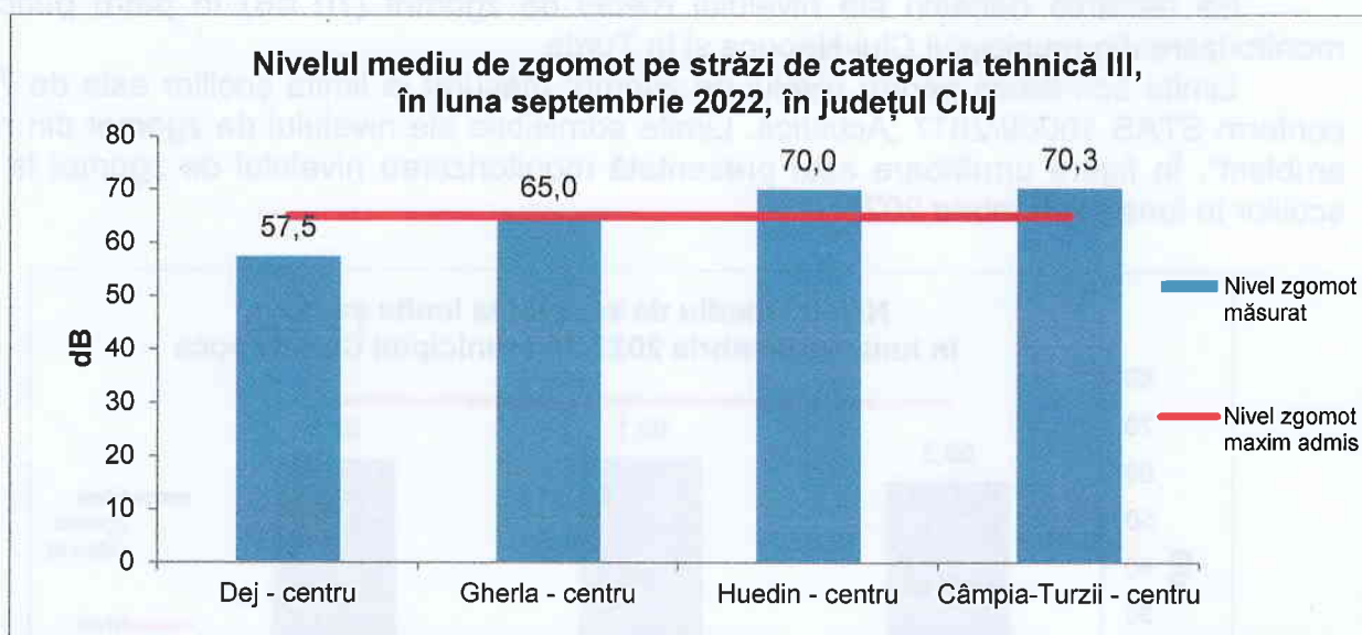
Figura 4.1. Nivelul de zgomot urban pe strazi de categoria III, în județul Cluj, în luna septembrie 2022
