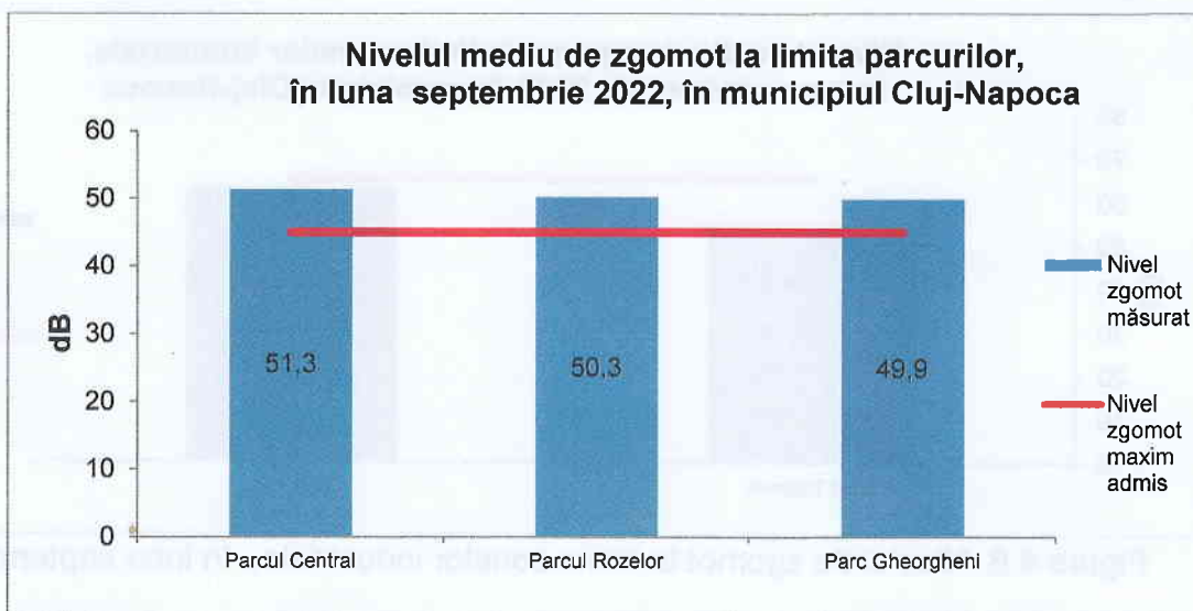
Figura 4.4. Nivelul de zgomot la limita parcurilor, în luna septembrie 2022
