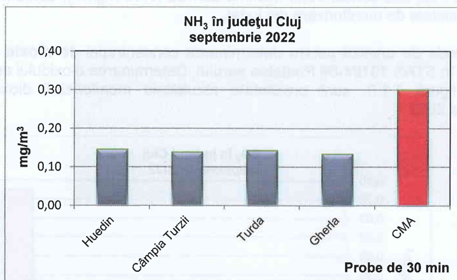
Figura 1.1.1. Evoluția concentrației de amoniac în județul Cluj în luna septembrie 2022
