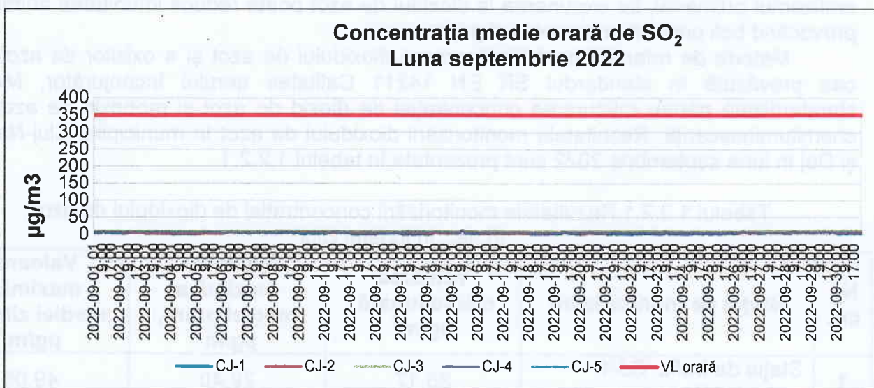
Figura 1.2.1.2. Evoluția concentrației medii orare de SO 2 în județul Cluj în luna Septembrie 2022
