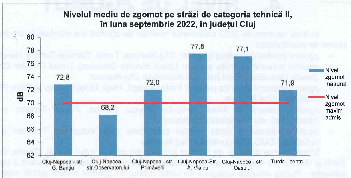
Figura 4.2. Nivelul de zgomot urban pe străzi de categoria II, în județul Cluj, în luna septembrie 2022
