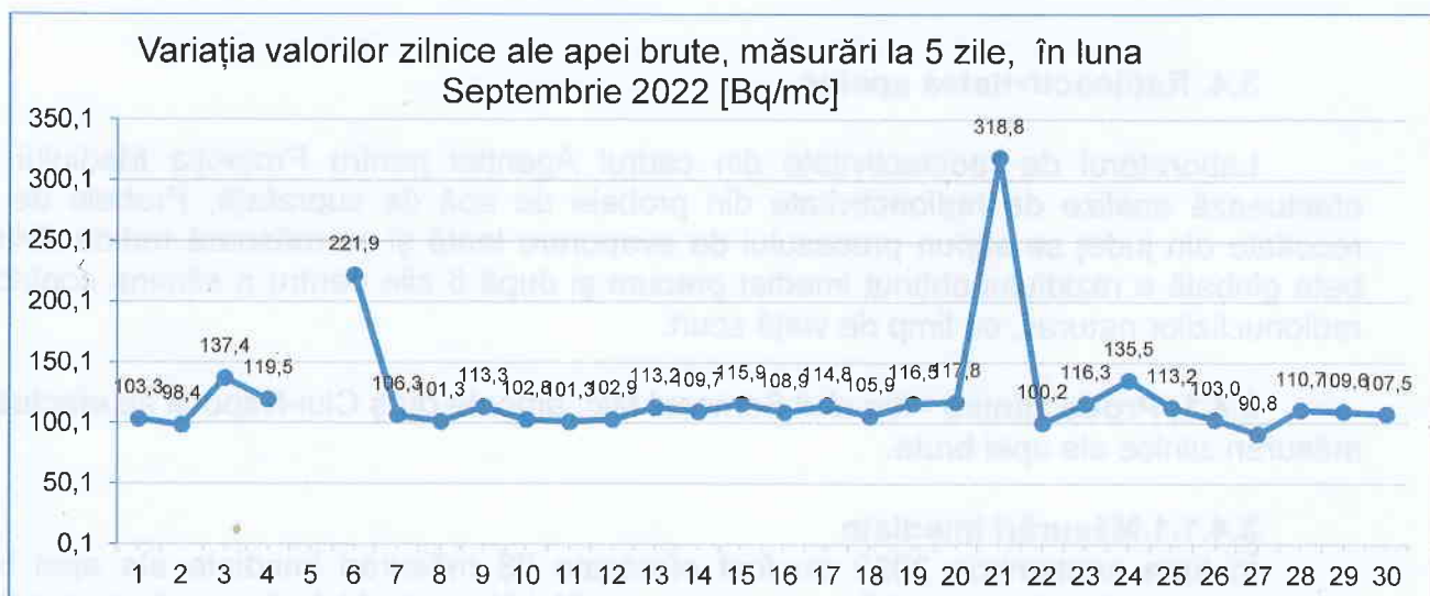
Figura nr. 3.4.1.2.1 Variația valorilor zilnice ale apei brute, măsurări la 5 zile, luna septembrie 2022
