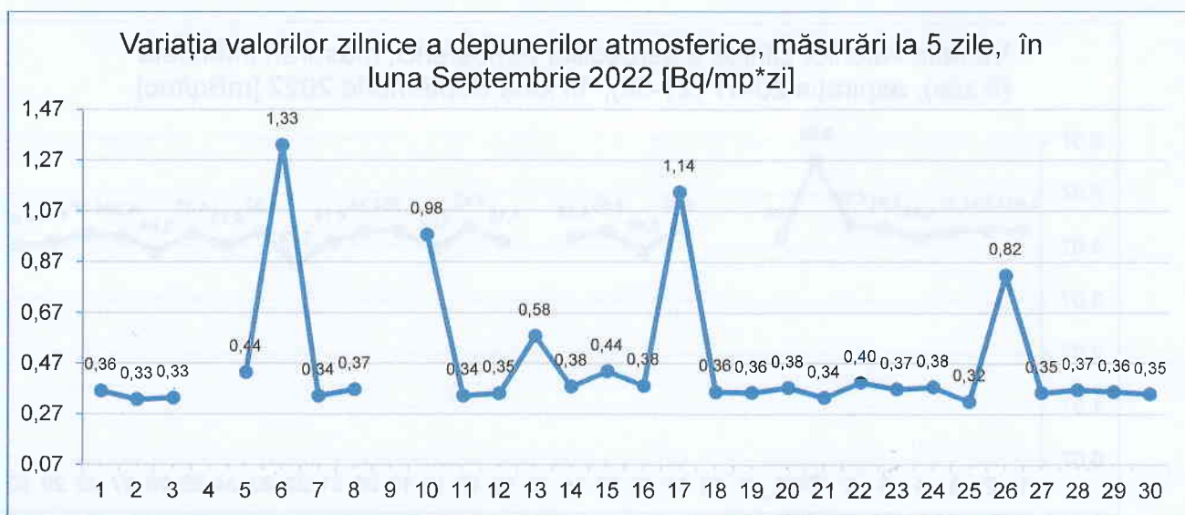
Figura nr. 3.3.2.1 Variația valorilor zilnice a depunerilor atmosferice, măsurări la 5 zile, luna septembrie 2022 [Bq/mp*zi]
