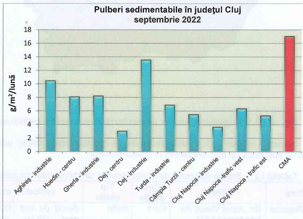
Figura 1.1.4. Evoluția concentrației de pulberi sedimentabile în județul Cluj în luna septembrie 2022
