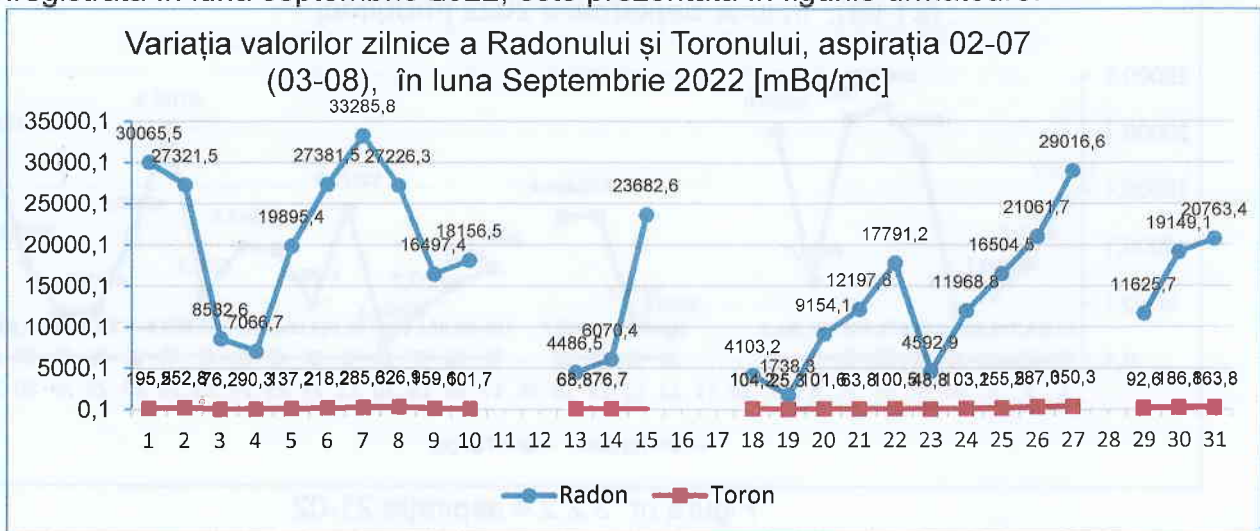
Figura nr. 3.2.2.1 aspirația 3-8
